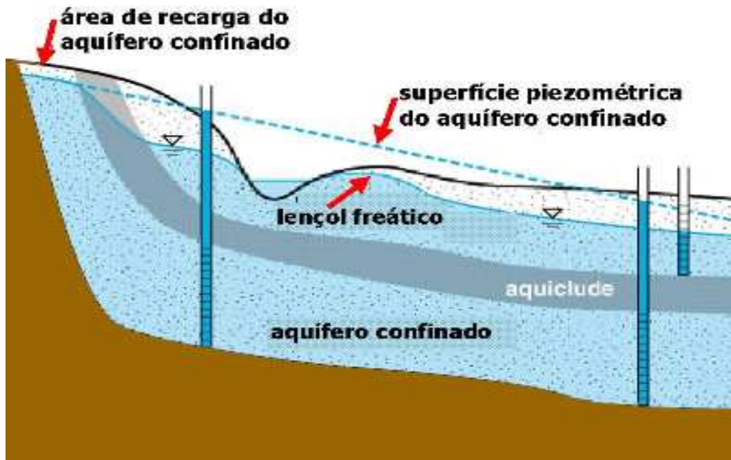
Figura 2.2 – Água subterrânea.
