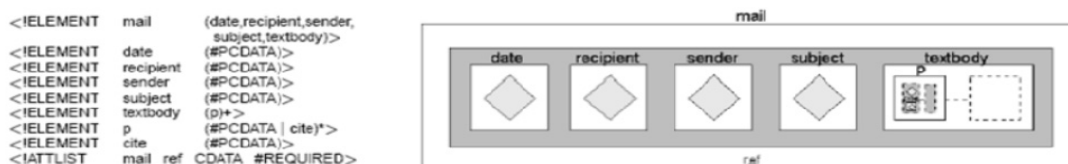
Figura 6.3: Dados XML Representados em VXT
