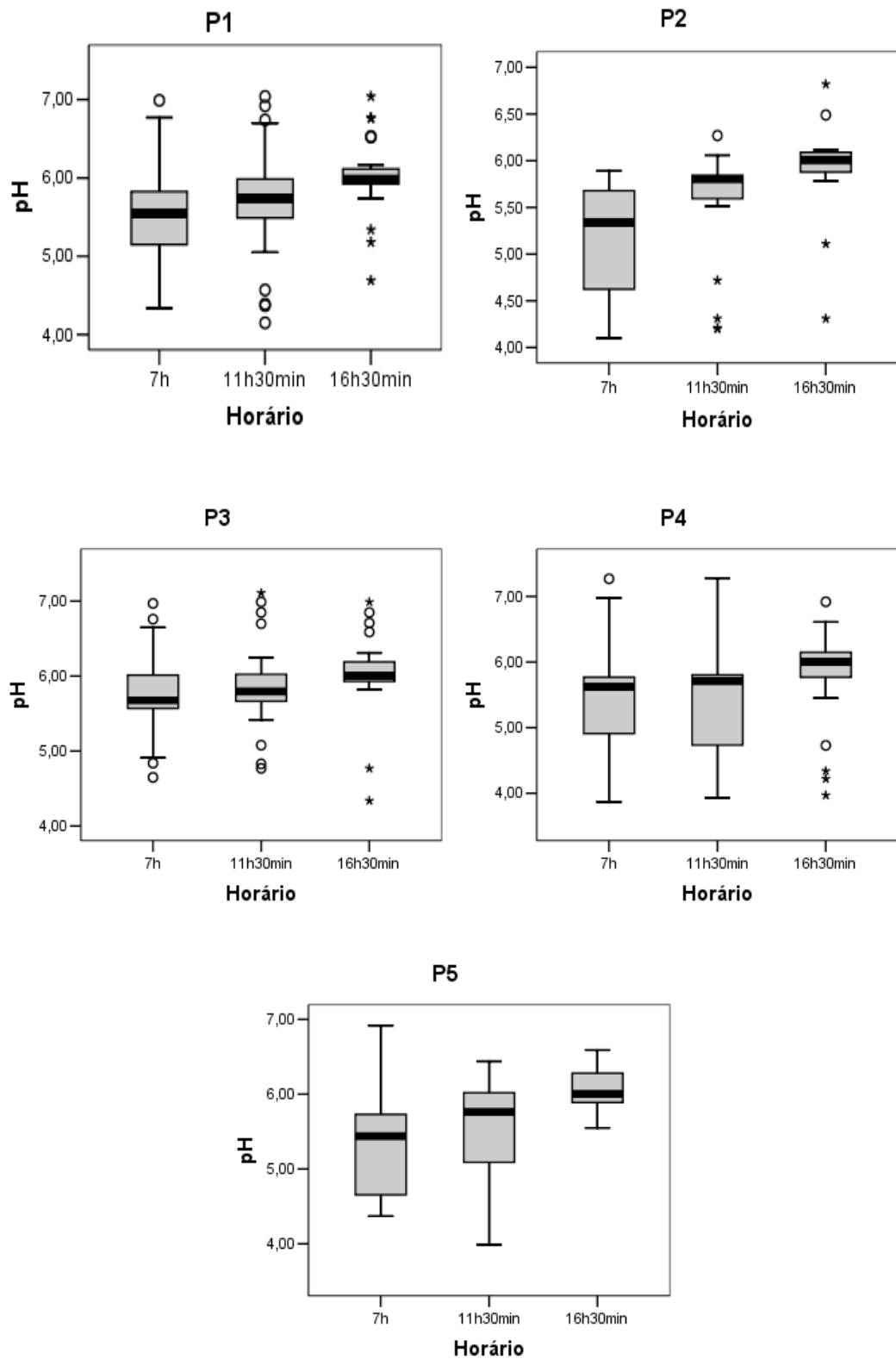
Figura 6.16 – Gráficos BOX PLOT de distribuição de valores de pH nos cinco pontos de coleta.
