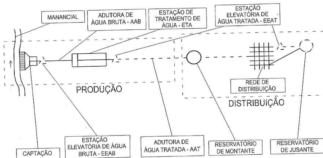
Figura 3.1 – Unidades componente de um sistema de abastecimento de água Fonte: HELLER (2006).
