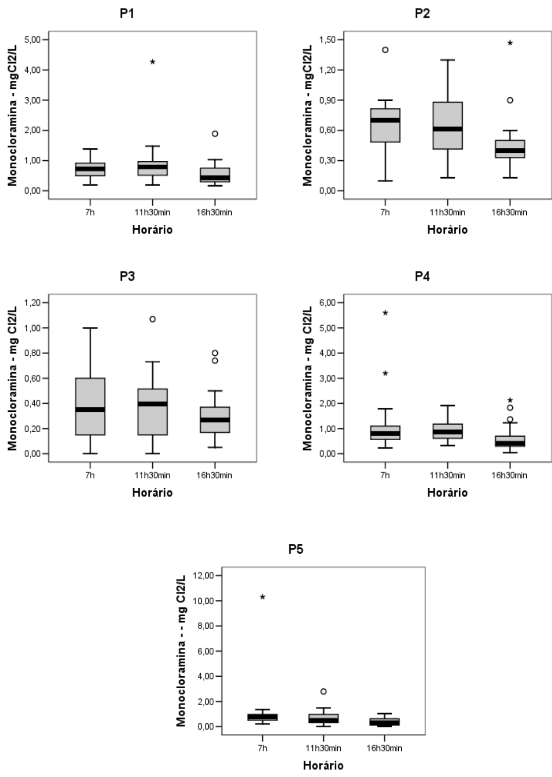
Figura 6.2 – Gráficos BOX PLOT de distribuição das concentrações de monocloramina, medidas nos três horários nos pontos de coleta.
