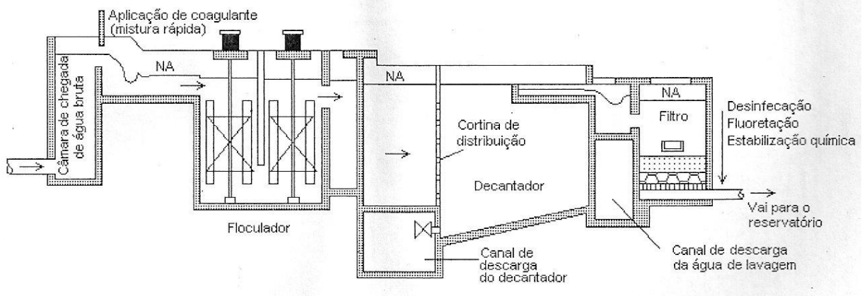
Figura 3.5 – Esquema em corte de uma ETA convencional ou de ciclo completo. Fonte: Pádua (2006).
