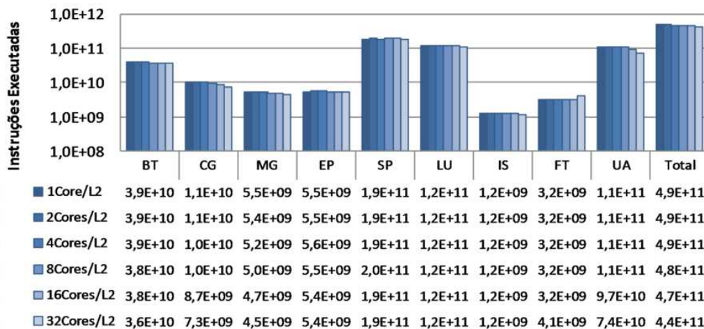
Figura 4.30: Instruções executadas do segundo experimento (4 MB).
