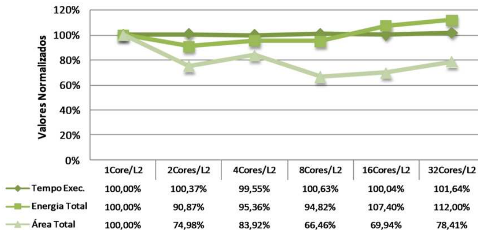
Figura 4.11: Sumário de desempenho, consumo de energia e ocupação de área do primeiro experimento.
