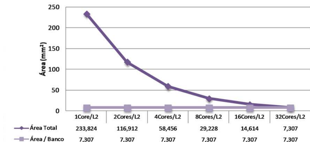
Figura 4.19: Ocupação de área pela memória cache L2 do segundo experimento (1 MB).
