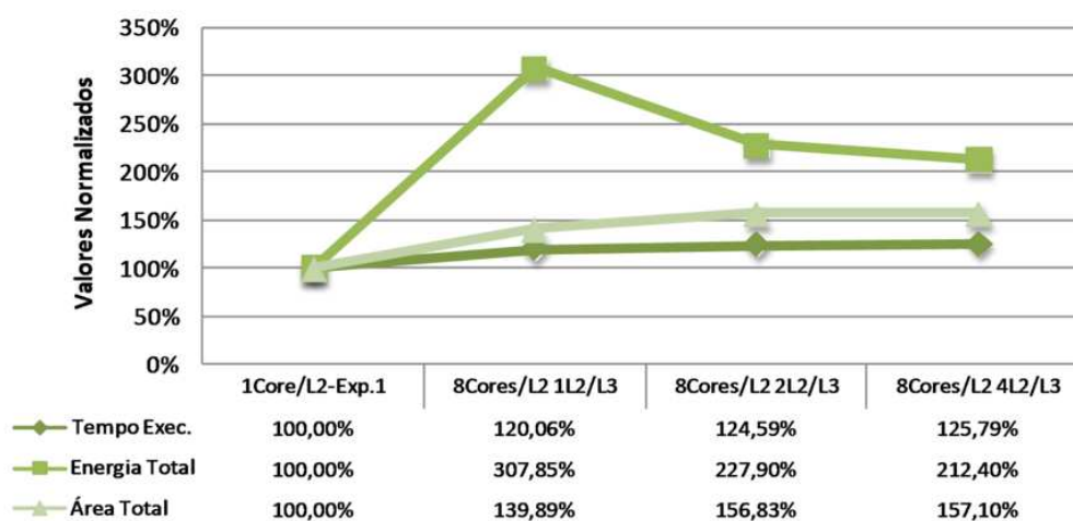
Figura 4.65: Sumário de desempenho, consumo de energia e ocupação de área do quinto experimento.
