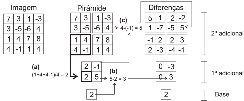
Figura 2.5: Exemplo da criação da pirâmide laplaciana para redução dos quadros.
