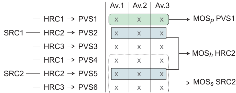
Figura 4.1: Exemplo dos votos utilizados para cálculo dos valores MOS.
