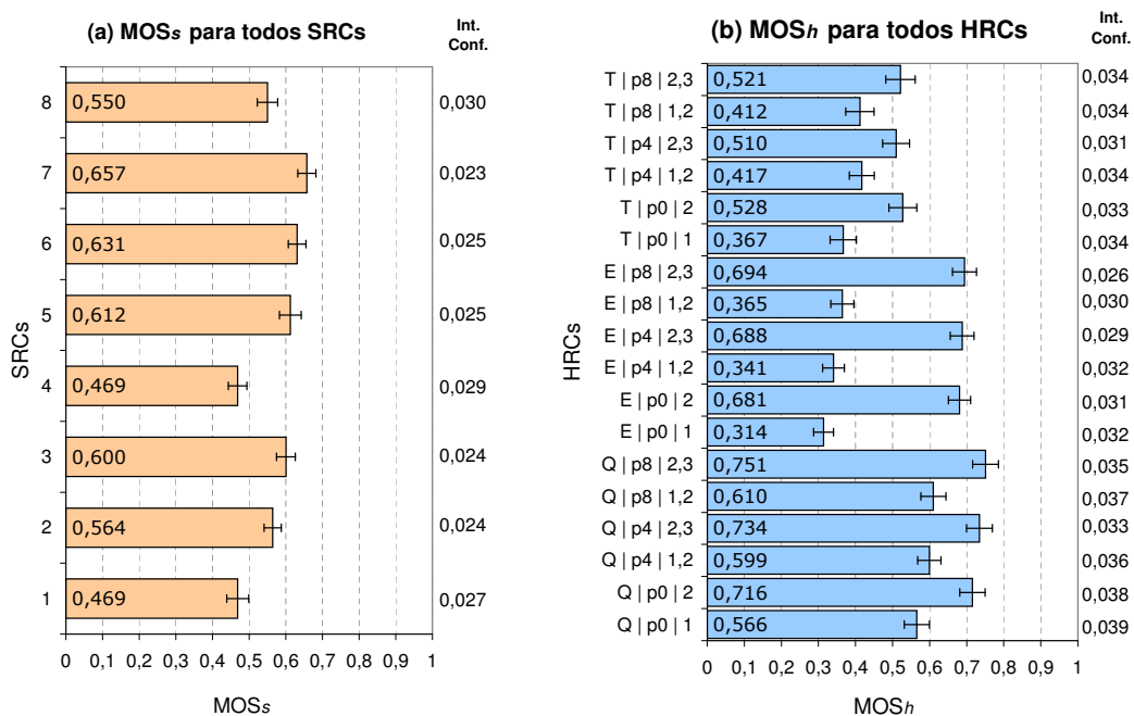
Figura 4.5: MOS para todos SRCs e HRCs.
