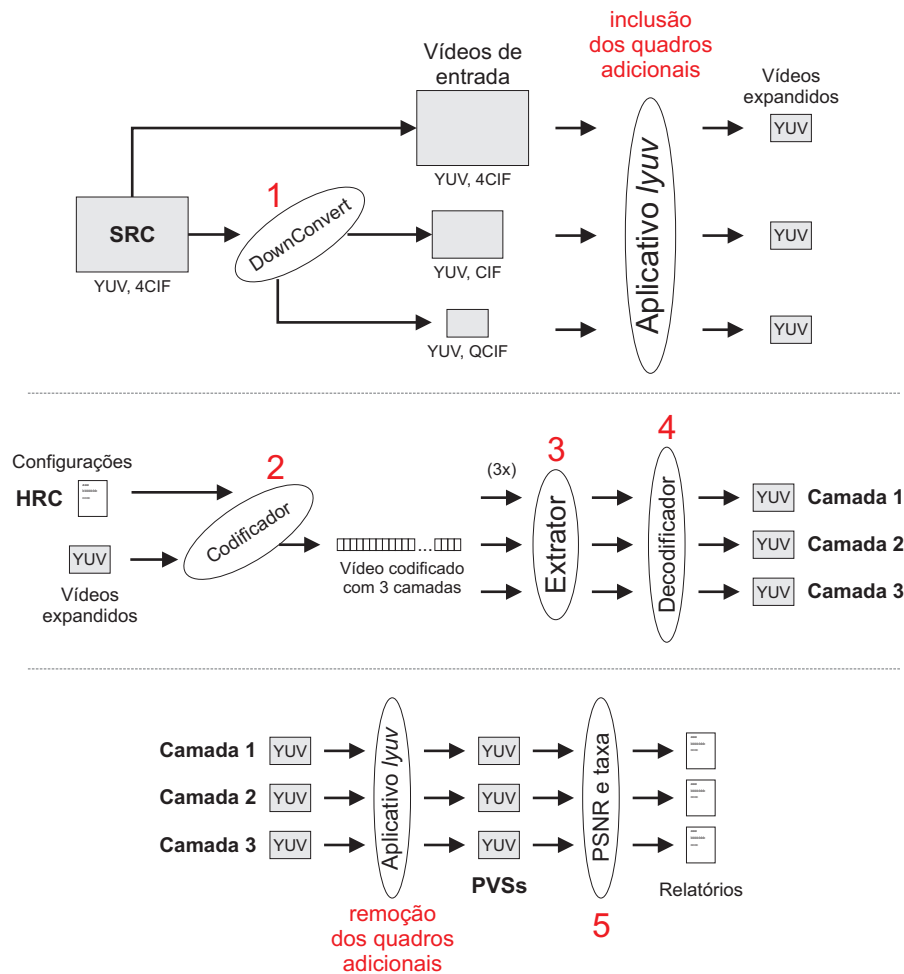
Figura 3.9: Etapas do processo de codificação escalável utilizando o JSVM.
