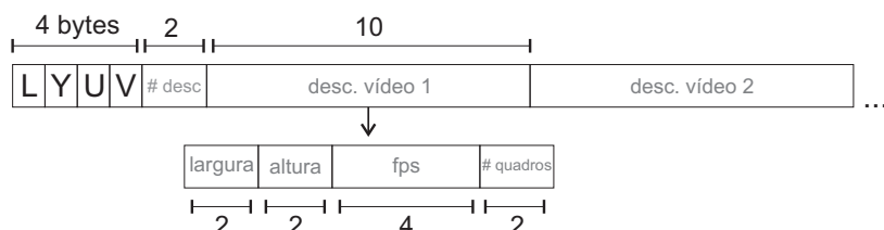
Figura B.1: Cabeçalho incluído pela operação “Encode”.
