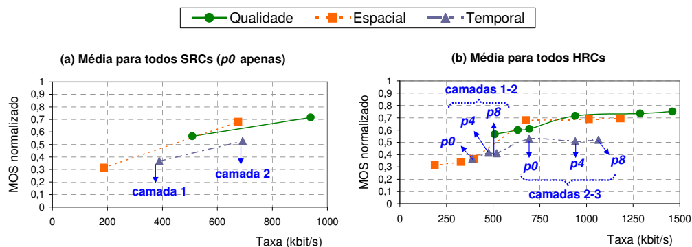
Figura 4.7: Análise da qualidade em relação à taxa de codificação dos vídeos.
