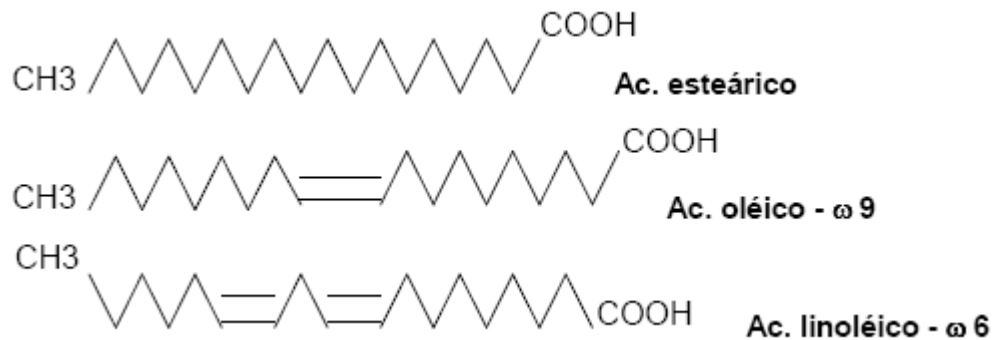
Figura 3 – Estrutura dos ácidos graxos esteárico, oléico e linoléico.
