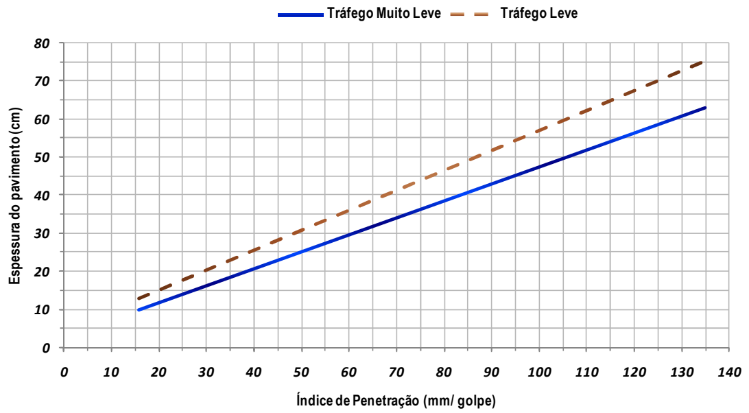
Figura 4.23 – Âbaco de dimensionamento da espessura total da estrutura do pavimento em função do índice de penetração do CPD, e do tráfego (T), para o método proposto
