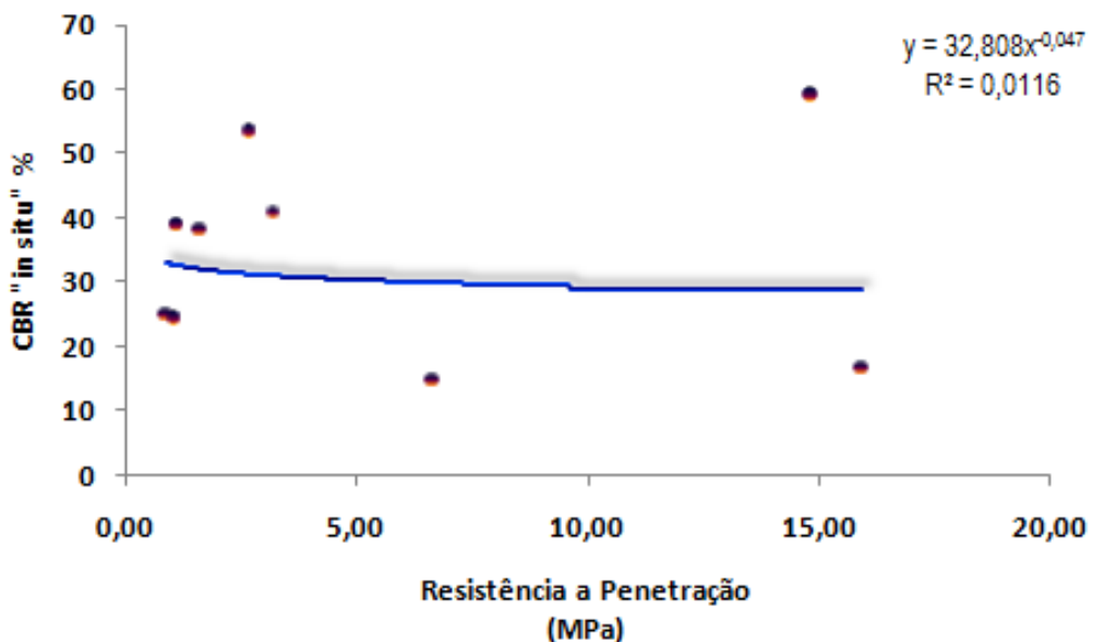
Figura 4.21 – Gráfico de correlação entre os valores da Resistência a Penetração do CPE versus
