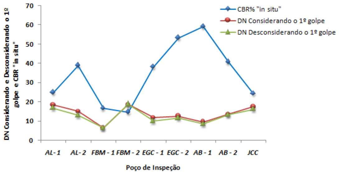
Figura 4.2 – Índice de Penetração (considerando e desconsiderando o 1º golpe) e CBR “in situ”.
