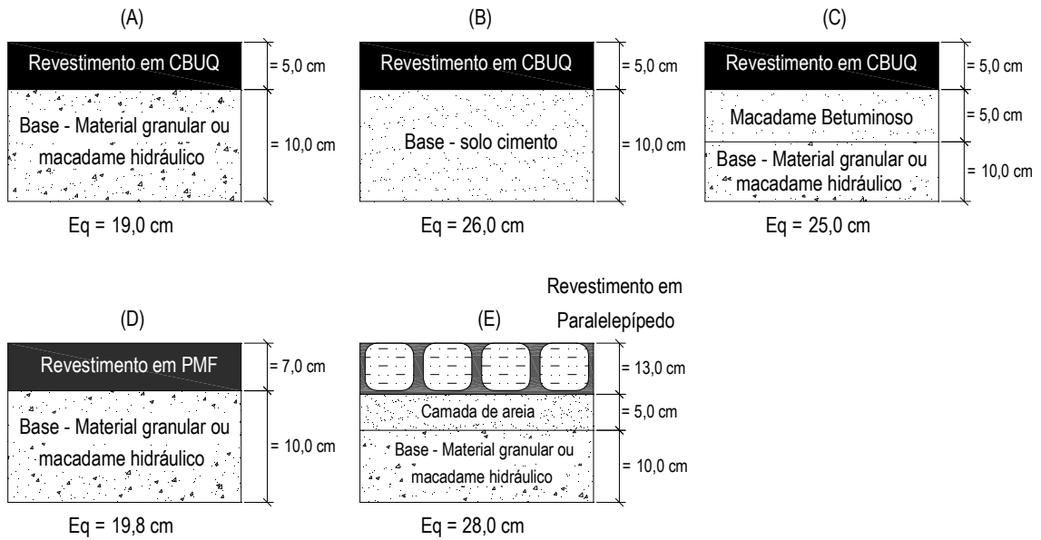
Figura 4.25 – Projetos-tipo de pavimentos para o tráfego leve, método proposto (GUEDES, 2008).
