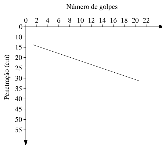
Figura 2.18 – Gráfico do CPD
