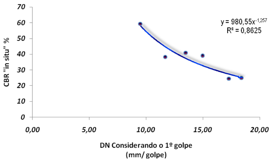
Figura 4.5 – Gráfico de correlação CPD Considerando o 1º golpe x CBR "in situ".
