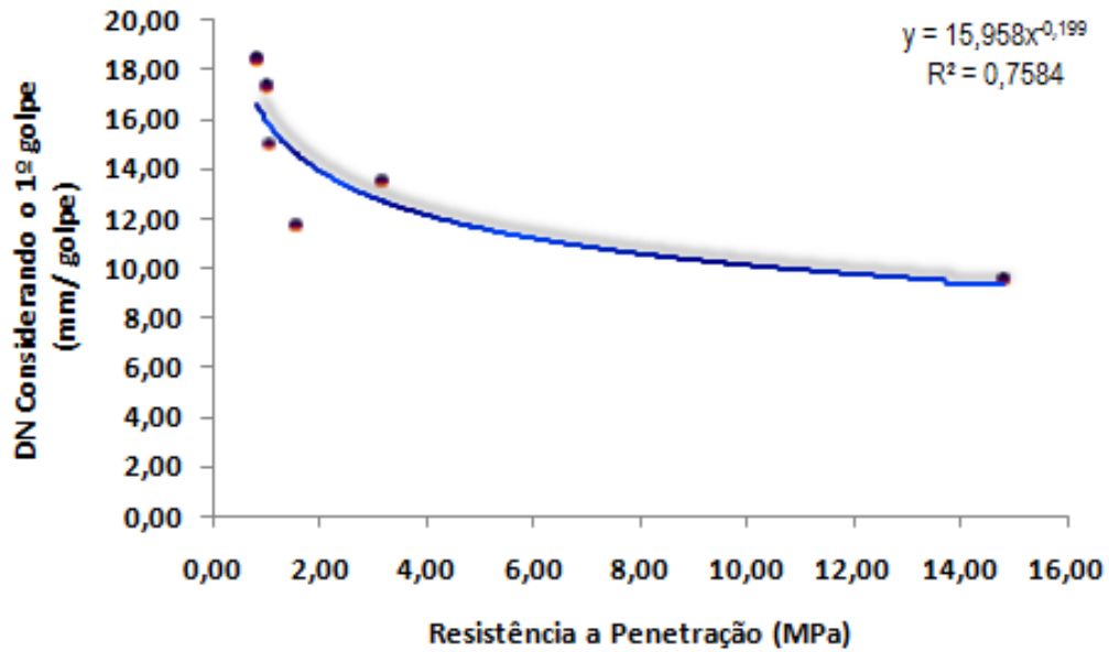
Figura 4.15 – Gráfico de correlação DN Considerando o 1º golpe x CPE.
