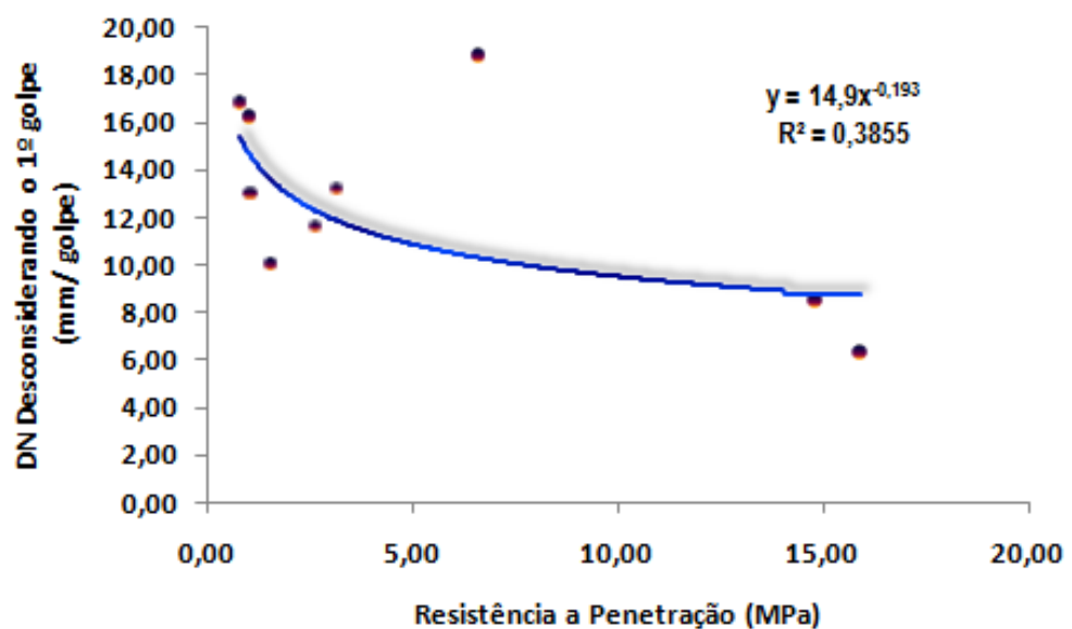
Figura 4.14 – Gráfico de correlação DN Desconsiderando o 1º golpe x CPE.
