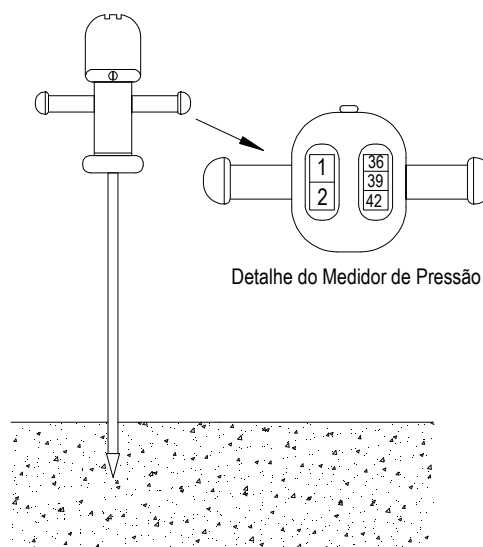
Figura 2.15 – Penetrômetro Britânico
