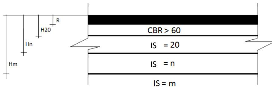
Figura 2.10 – Camadas do Pavimento (SENÇO, 1997).
