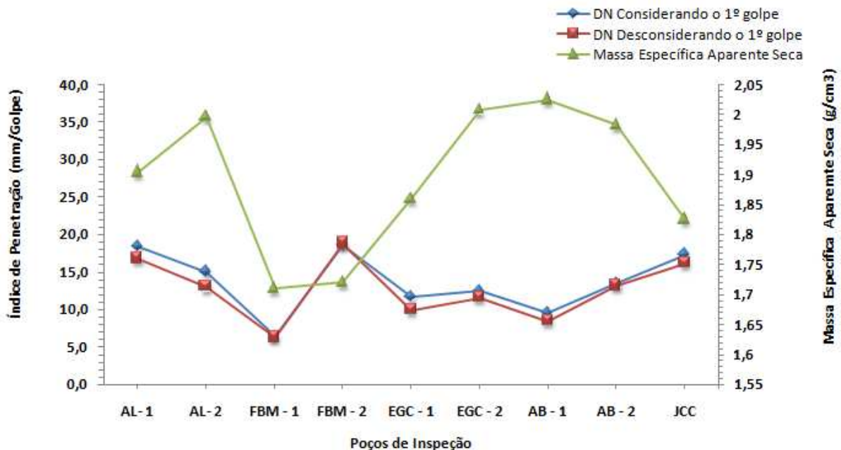
Figura 4.7 - Índice de Penetração (considerando e desconsiderando o 1º golpe) e valores da Massa Específica Aparente Seca.
