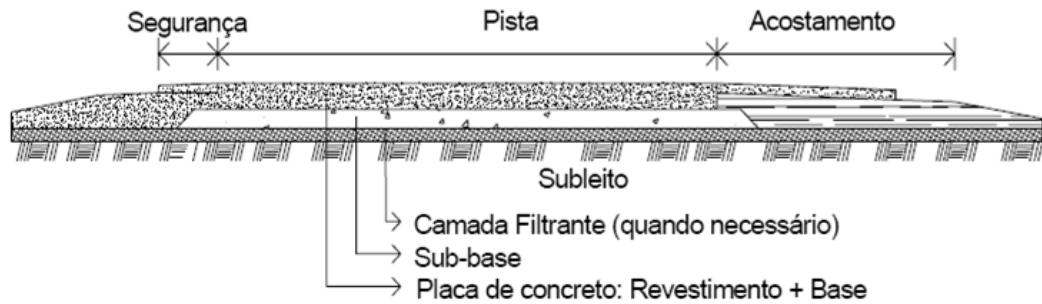
Figura 2.5 – Estrutura do pavimento rígido (Fonte: SILVA JÚNIOR, 2005).
