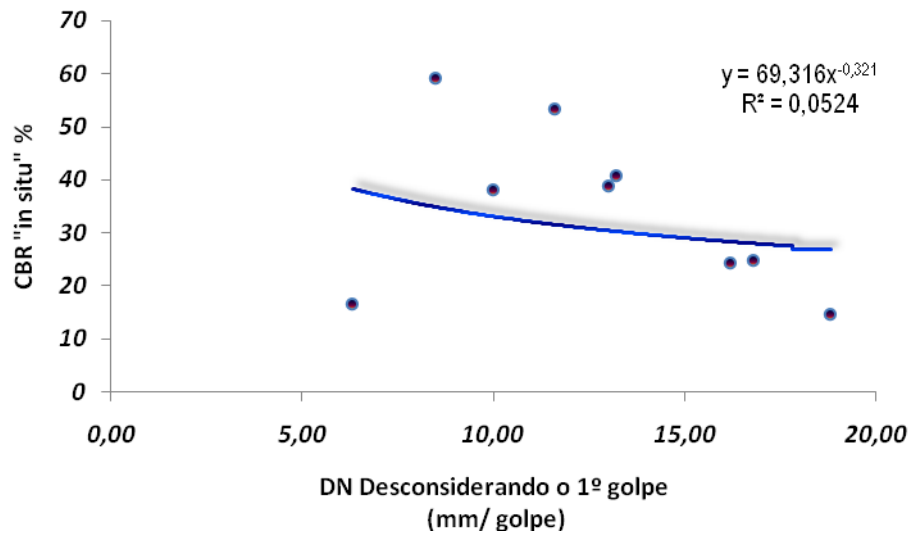
Figura 4.4 – Gráfico de correlação CPD Desconsiderando o 1º golpe x CBR "in situ".
