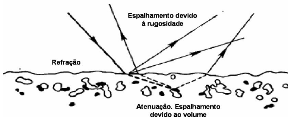
Figura 2.2. Mecanismos de espalhamento acústico no fundo, incluindo a refração na interface água-sedimento, além da atenuação e espalhamento no volume de sedimento. Modificado de Jackson et al (1986)
