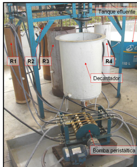
Figura (3.3b): Fotografia da estrutura dos reatores.
