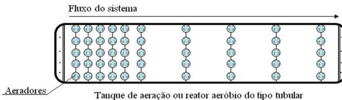
Figura (2.3): Tanque de aeração com distribuição de oxigênio escalonada ao longo do reator em função da demanda prevista
