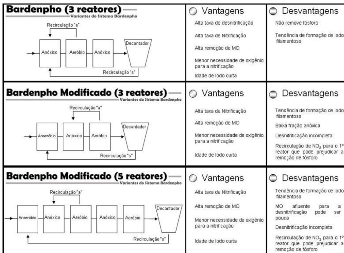
Figura (2.4): Variantes do sistema do tipo Bardenpho, assim como algumas de suas vantagens e desvantagens.
