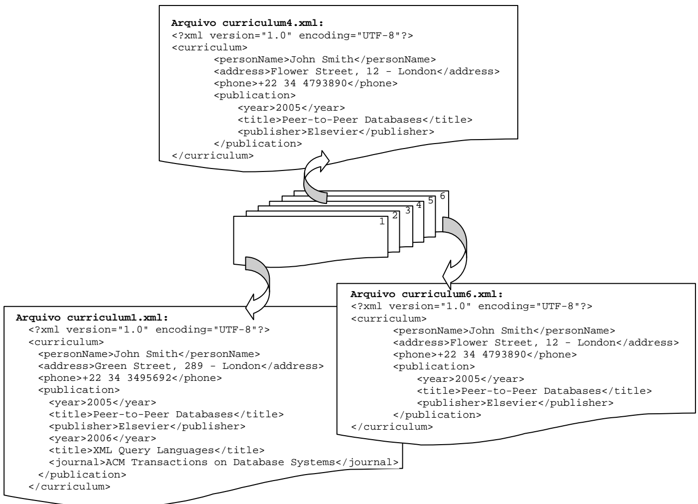
Figura 4.1: Arquivos XML “ curriculum1.xml ”, “ curriculum4.xml ” e “ curriculum6.xml ”
