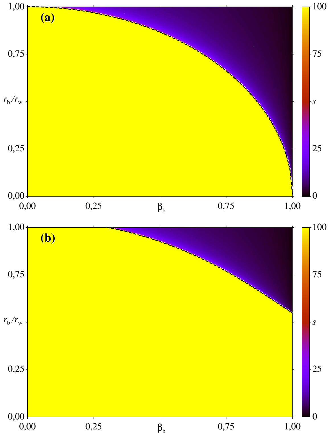
Figura 3.7: Resultados numéricos para o teste massivo da condição de estabilidade de (a) feixes com emitâncias iniciais \epsilon = 0 (frio) e (b) feixes quentes tipo waterbag com emitâncias iniciais \epsilon = 0,3\sigma_0 r_w^2 . A escala de cores indica o tempo s em que o feixe perde a estabilidade, caso ocorra (regiões azul e preto). Na região amarela, o feixe é estável. As curvas teóricas são mostradas em linhas pontilhadas, obtidas da condição de estabilidade teórica, para cada caso de emitância inicial.
