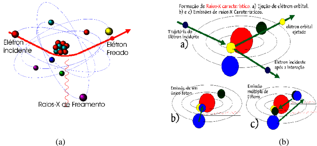
Figura II. 1: Conversão de energia cinética dos elétrons em radiação X. (a) Raios X de bremstrahlung ou freamento, resultante da interação de elétrons rápidos com o campo coulombiano do núcleo do alvo, o elétron é bruscamente desacelerado. (b) Raios X característicos, devido à interação coulombiana entre um elétron energético do feixe e o elétron atômico. O elétron incidente pode ceder energia suficiente para retirar um elétron de seu nível de energia muito negativo e ejetá-lo do átomo, deixando o átomo num estado altamente excitado. O átomo poderá voltar a seu estado fundamental emitindo um conjunto de fótons de alta energia, cuja energia é igual à diferença de energia entre o estado inicial e o final.
