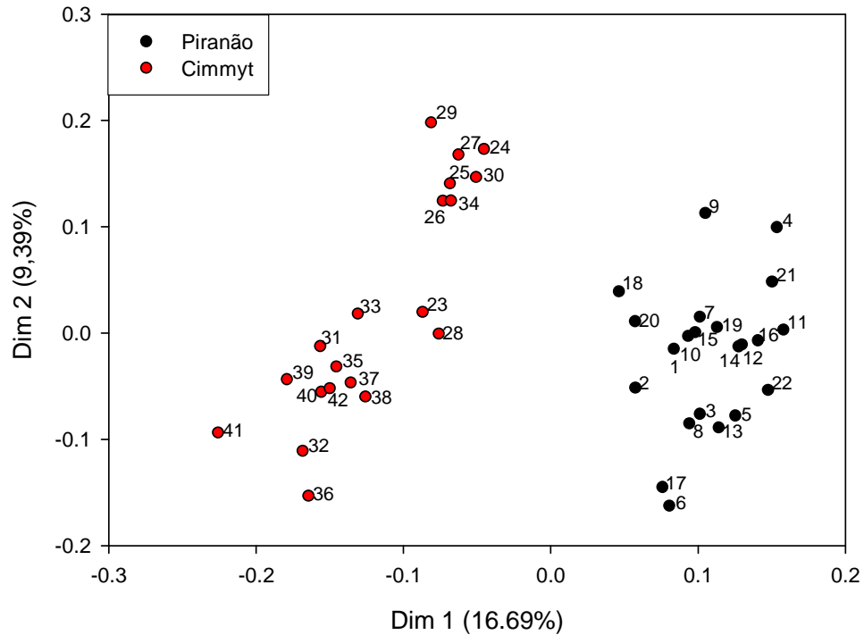
Figura 2: Gráfico das Coordenadas Principais, gerado pelo programa Darwin 5.0, das 42 famílias selecionadas para a etapa de recombinação. Os genótipos de 1 a 22 pertencem ao grupo Piranão e os genótipos de 23 a 42 pertencem ao grupo CIMMYT (Apêndice C).
