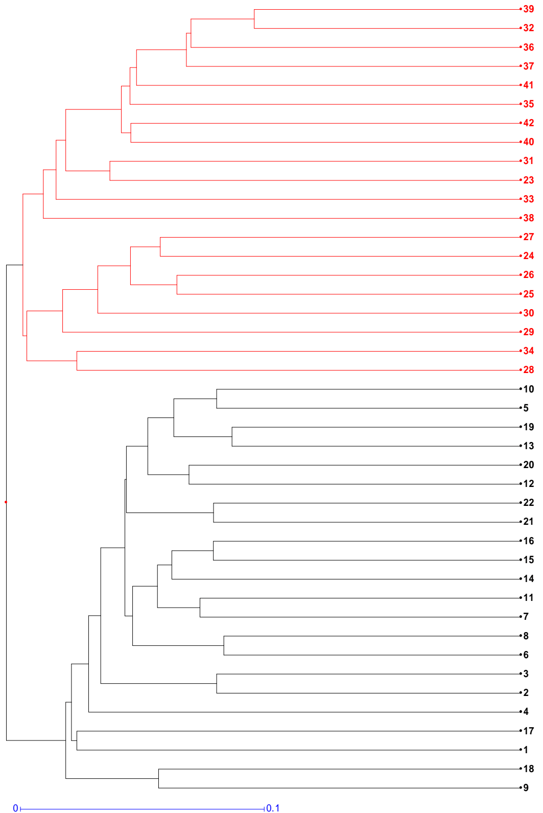
Figura 3: Dendrograma obtido pelo método hierárquico UPGMA, utilizando, como medida de dissimilaridade, o complemento aritmético do índice de Jaccard. Os números em preto correspondem aos genótipos provenientes da população Piranão e os números circulosados em vermelho, provenientes da população CIMMYT (Apêndice C).
