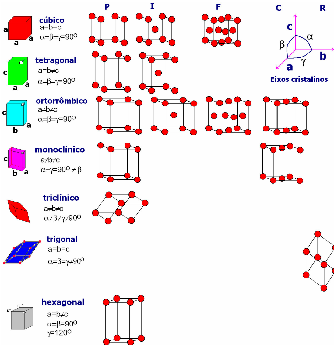
Figura 13: Os 14 retículos de Bravais. Eles são formados a partir de sete sistemas cristalinos: cúbico, tetragonal, ortorrômbico, monoclinico, triclinico, trigonal e hexagonal.
