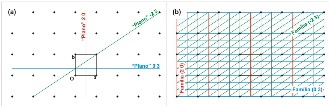
Figura 15: Uma rede cristalina bidimensional ilustrando os índices de Miller para certo conjunto de “planos”. (a) Rede cristalina com uma cela unitária situada na origem O e três “planos” cruzando os eixos a e b. (b) As três famílias de “planos” são obtidas com a repetição dos “planos” originais.
