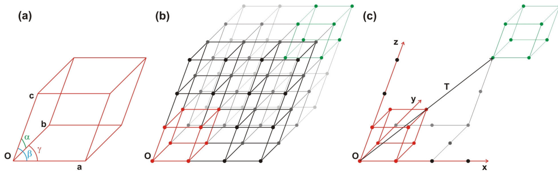
Figura 12: Representação de uma cela unitária geral. (a) Cela unitária com eixos a , b e c e ângulos \alpha , \beta e \gamma situada na origem O . (b) A rede cristalina é obtida com o arranjo tridimensional das células unitárias. (c) Qualquer cela unitária do cristal está relacionada com a cela da origem por uma operação de translação T .
