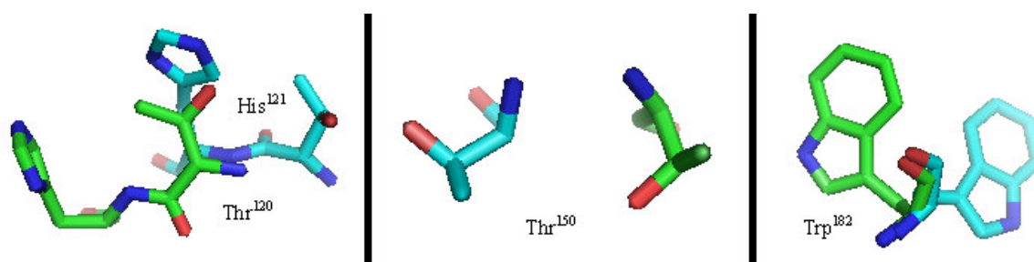
Figura 33.a: Sobreposição dos resíduos com o valor de RMSD relativamente altos da proteína CML nativa (em verde claro) e CML complexada com o açúcar man 1-6 man (em azul claro).
