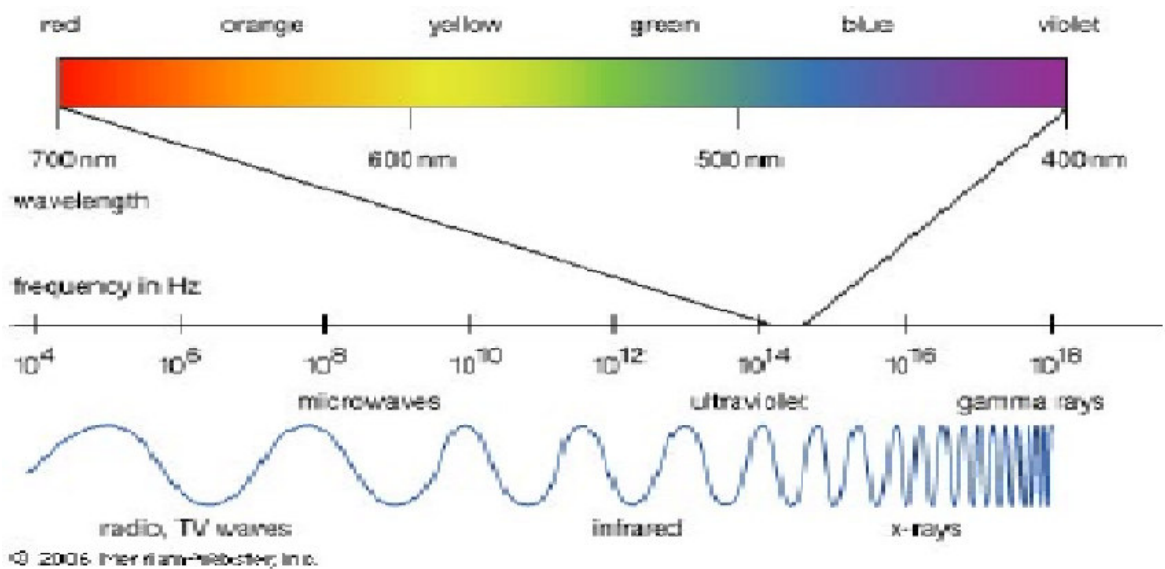
Figura 16: Espectro eletromagnético.
