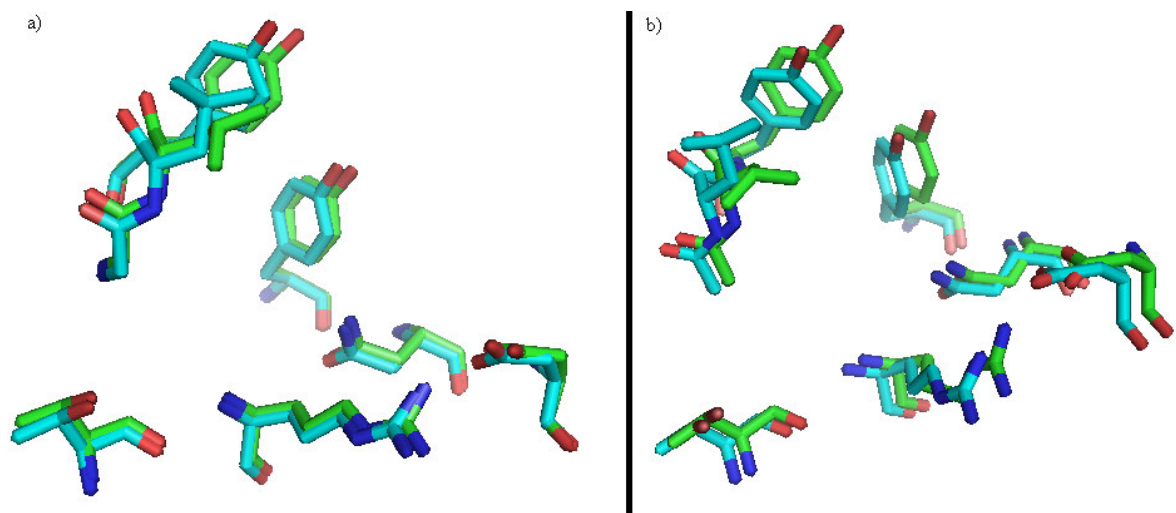
Figura 35.a: Sobreposição dos resíduos do sítio ativo das proteínas CML nativa (em verde claro) e CML complexada com o açúcar man 1-6 man (em azul claro). a) Monômero A. b) Monômero B. Programa utilizado Pymol (DELANO, 2004).
