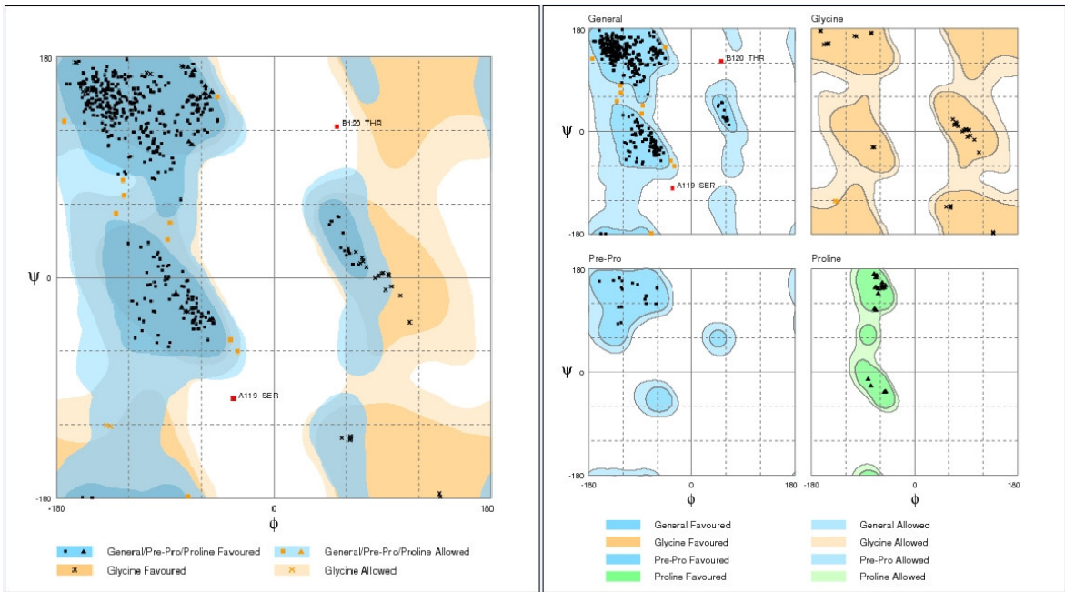
Figura 31.a: Diagrama de Ramachandran \Phi - \Psi para a estrutura CML man 1-6 man. Imagem gerada utilizando o webservice RAMPAGE ( http://mordred.bioc.cam.ac.uk/~rapper/rampage.php ).
