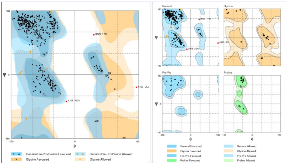
Figura 31.b: Diagrama de Ramachandran \Phi - \Psi para a estrutura CGL man 1-6 man. Imagem gerada utilizando o webservice RAMPAGE ( http://mordred.bioc.cam.ac.uk/~rapper/rampage.php ).
