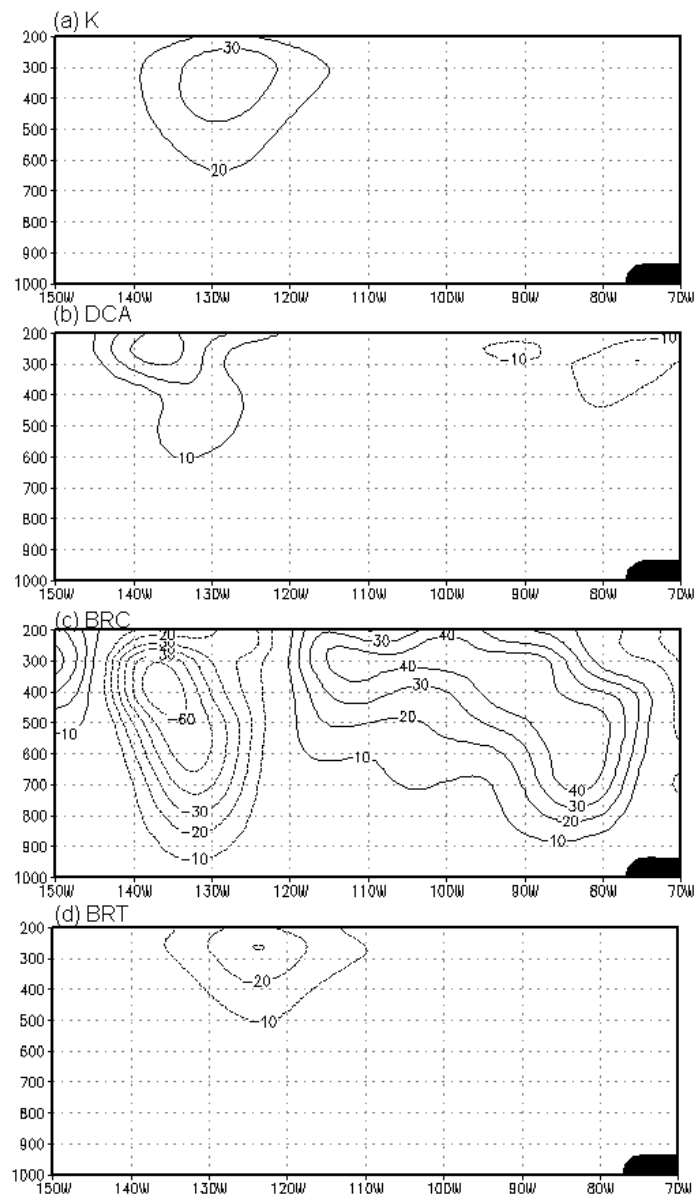
Figura 4.3- Corte longitude versus pressão na latitude de 50°S para o Dia-4. (a) K ( m^2/s^2 ), (b) Termo DCA ( 10^4 m^2/s^3 ), (c) Conversão BRC ( 10^4 m^2/s^3 ) e (d) Conversão BRT ( 10^4 m^2/s^3 ).
