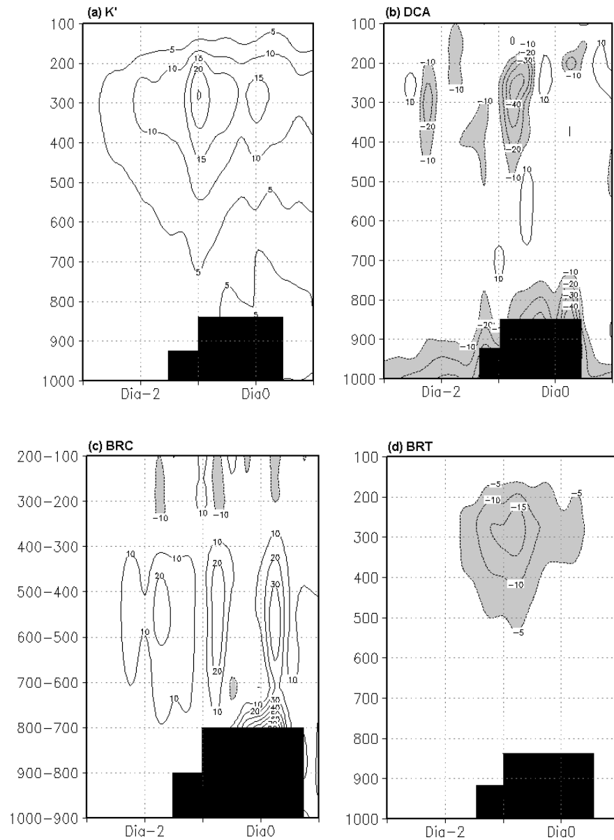
Figura 5.7 – Energética da anomalia positiva corrente acima da AN2: (a) K' ( m^2s^{-2} ), (b) DCA ( 10^5m^2s^{-3} ), (c) BRC ( 10^5m^2s^{-3} ) e (d) BRT ( 10^5m^2s^{-3} ). Os valores correspondem a média na área de 15^\circ \times 15^\circ centrado no ponto de máxima hgt' em cada nível. A área pintada de preto corresponde aos Andes.
