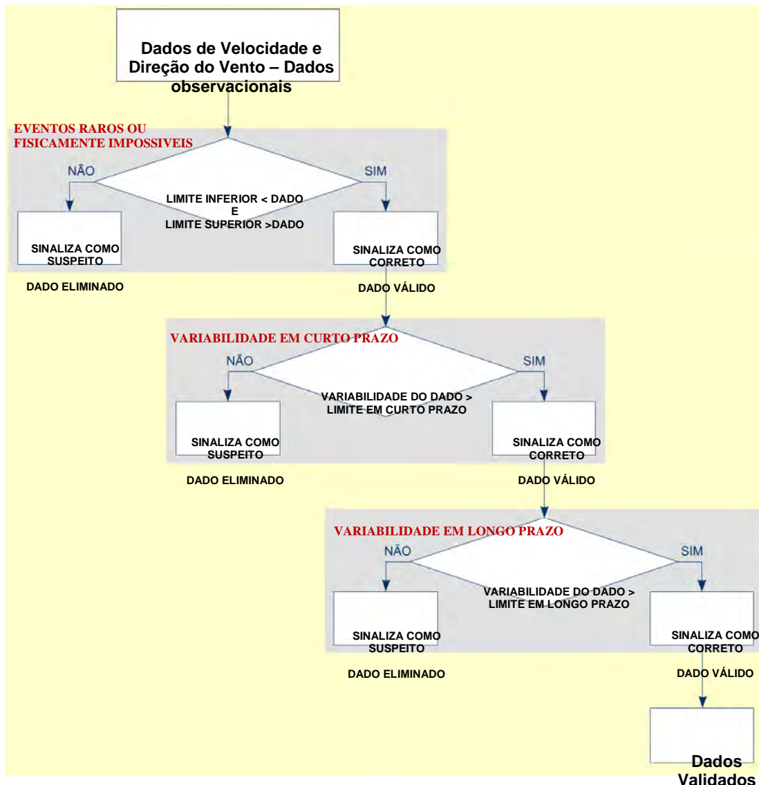
Figura 4.8 – Fluxograma representativo do algoritmo empregado para qualificação dos dados de direção e velocidade do vento.
