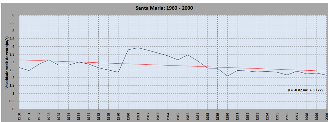
Gráfico de tendência da série observacional da estação de Santa Maria
