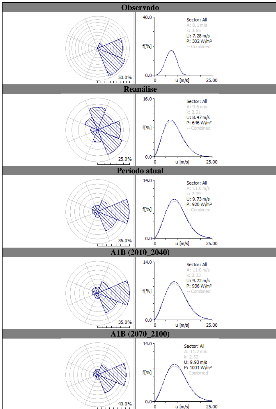
Histograma com direção e distribuição de Weibull para a estação de Santa Maria (Lat 29°42'39"S / Lon 053°41'32"W).
