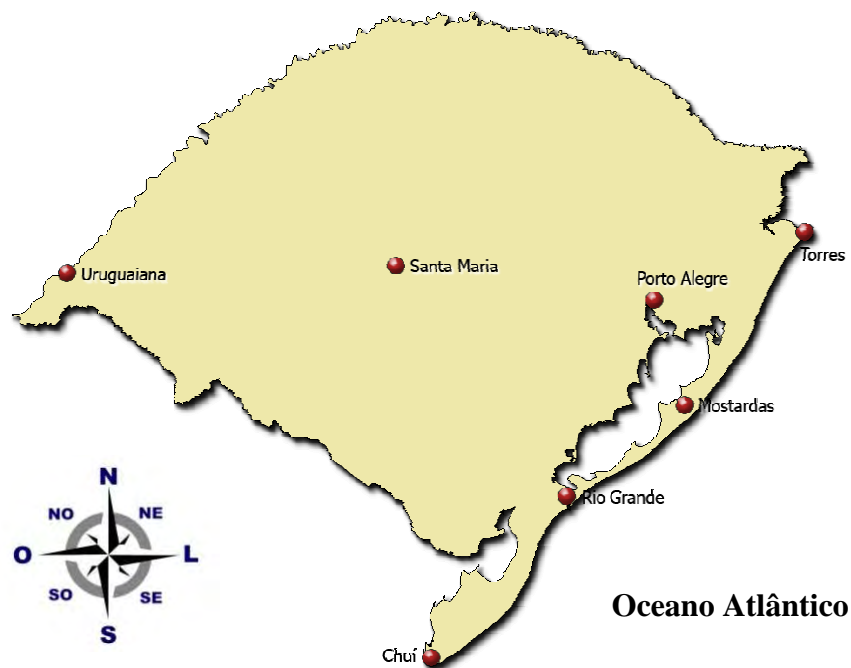
Figura 4.5 – Localização das estações de superfície utilizadas, no estado do Rio Grande do Sul.
