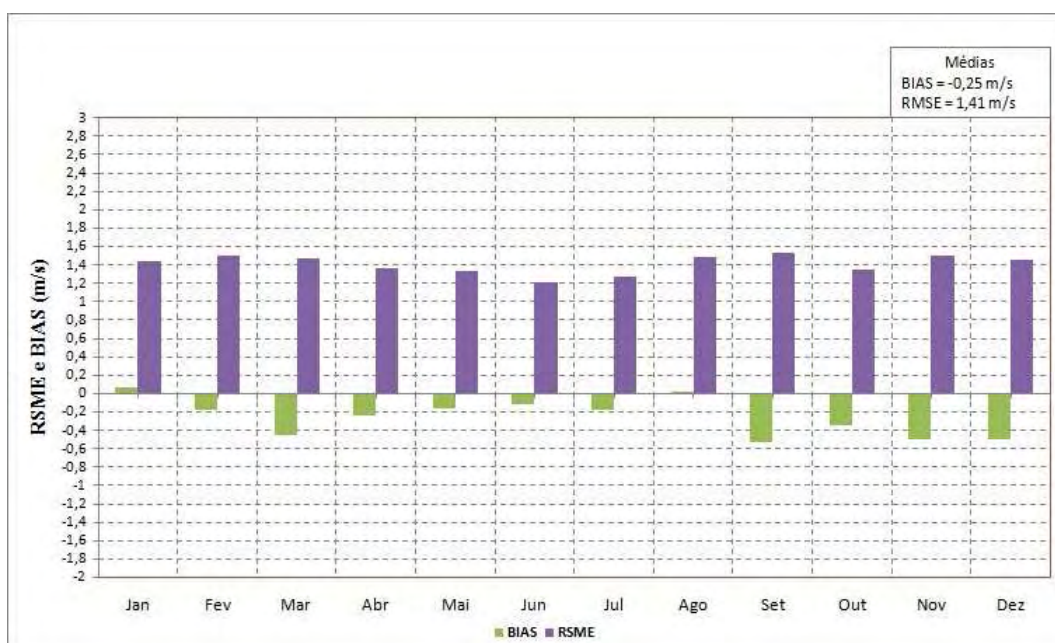
Figura 5.5 – RMSE e BIAS obtidos a partir do ciclo anual da velocidade do vento modelo Eta HadCM e observações para a estação de Chuí no período de 1964 a 1990.
