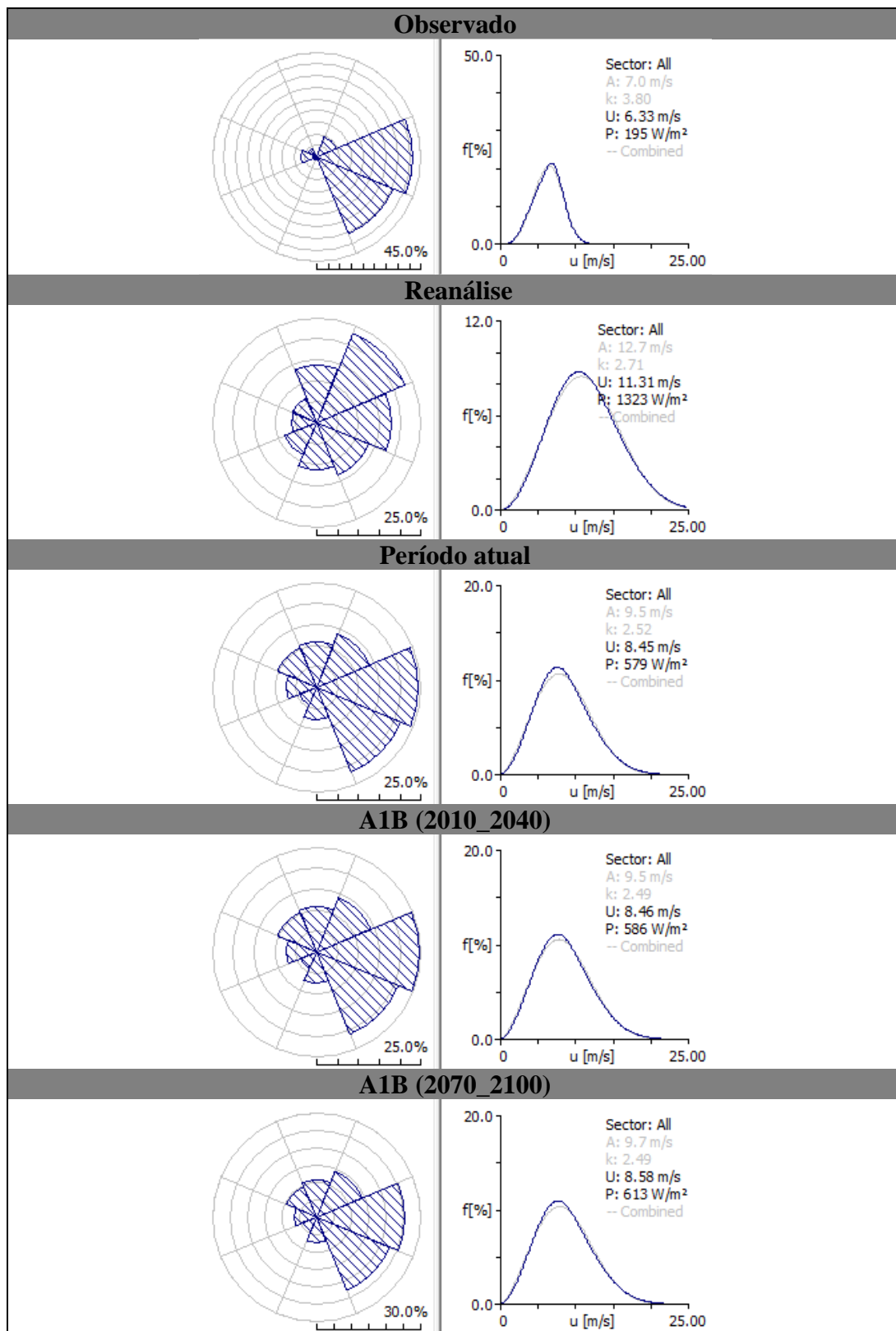
Histograma com direção e distribuição de Weibull para a estação de Porto Alegre (Lat 29°59'40"S / Lon 051°10'18"W).
