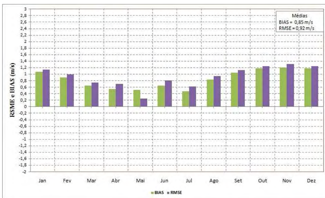
Figura 5.31 – RMSE e BIAS obtidos a partir do ciclo anual da velocidade do vento modelo Eta HadCM e reanálises ERA-40 para o período atual de Urugaiana.
