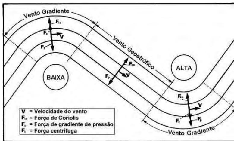
Figura 2.8 – Esquema mostrando o balanço entre força gradiente de pressão, força centrífuga e força de Coriolis para regiões em que as isóbaras são retas e regiões em que formam curvas.
