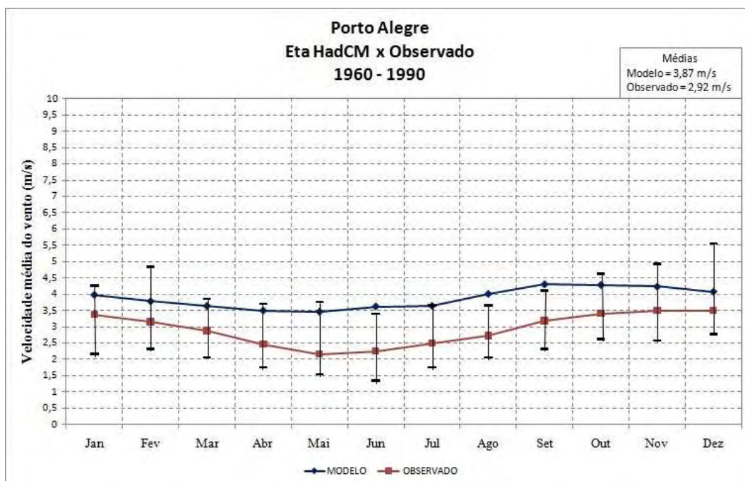
Figura 5.10 – Ciclo anual da velocidade do vento a 10 metros do modelo Eta HadCM e observações para a estação de Porto Alegre no período de 1960 a 1990.
