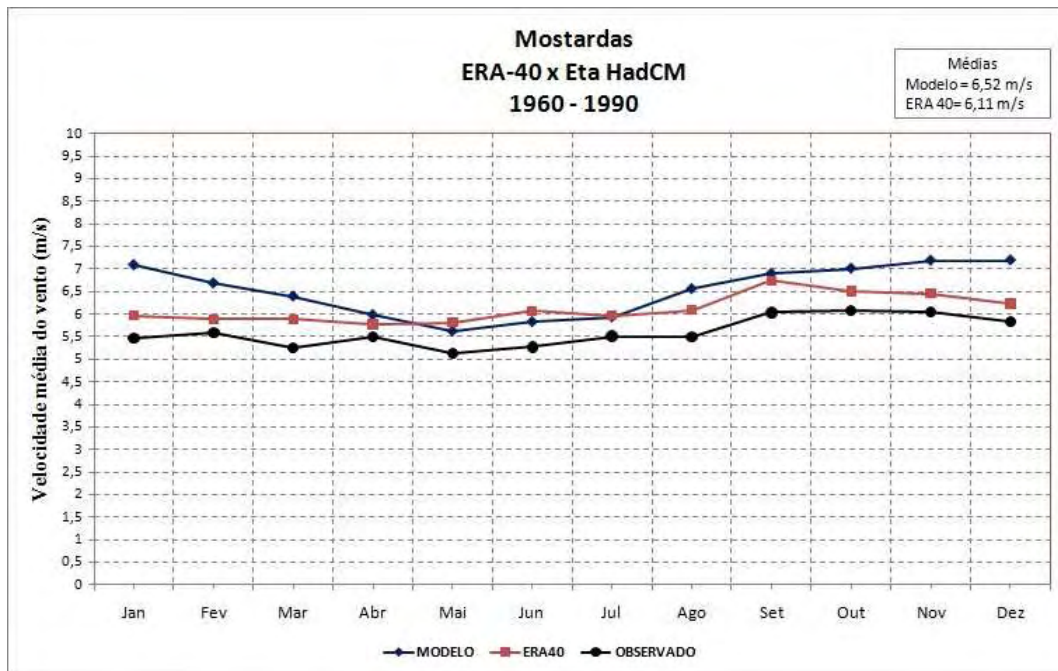
Figura 5.20 – Ciclo anual da velocidade do vento a 10 metros do modelo Eta HadCM e reanálises ERA-40 para o período atual de Mostardas.
