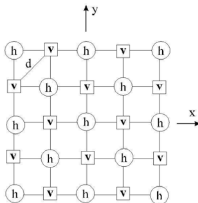
Figura 4.1 – Grade horizontal tipo E de Arakawa. Fonte: Modificado de Nickovic et al. (1998).
