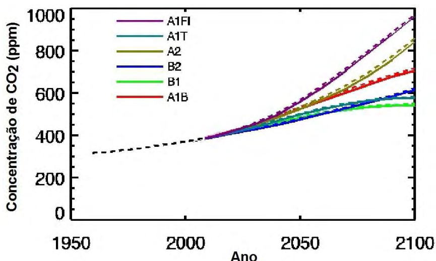
Figura 4.4 – Concentração real de CO 2 na atmosfera até o ano 2000. A partir de 2000 observa-se a concentração de CO 2 para os cenários de emissões do IPCC em partículas por milhão (ppm).
