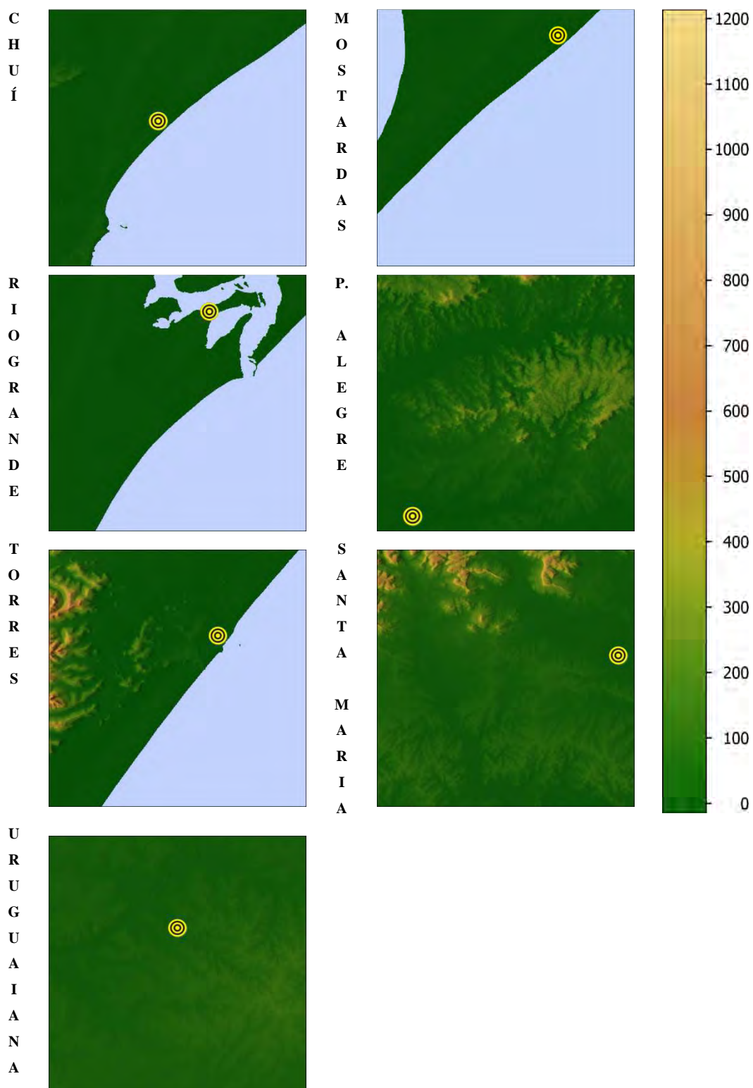
Figura 5.1 – Topografia de 40x40 km referente às grades do modelo Eta HadCM. A escala representa a altitude do continente em relação ao nível do mar, o qual está representado em azul. Por convenção, o nome do ponto de grade foi determinado com base no nome da estação que
