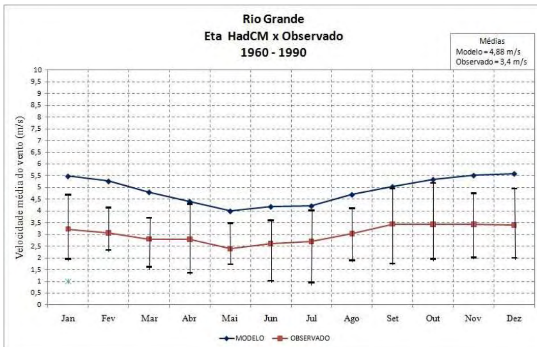
Figura 5.8 – Ciclo anual da velocidade do vento a 10 metros do modelo Eta HadCM e observações da estação de Rio Grande no período de 1960 a 1990.
