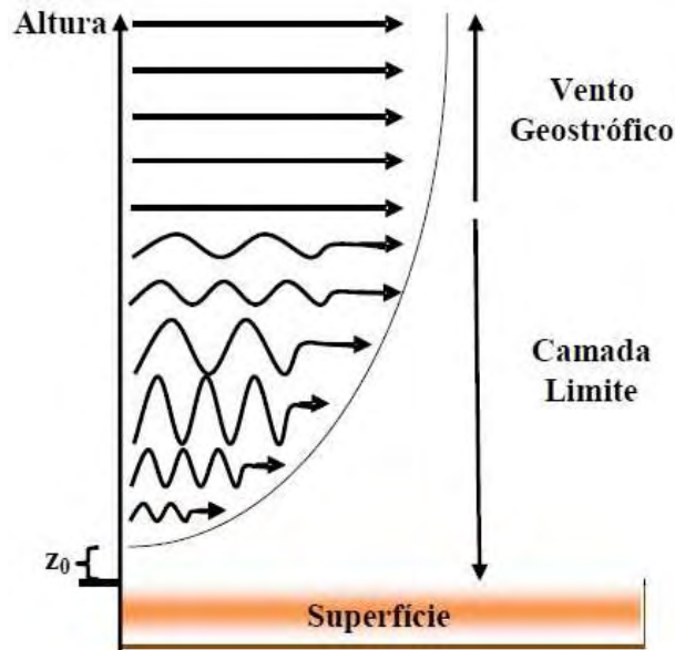
Figura 2.10 – Distribuição vertical do regime de circulação do vento.
