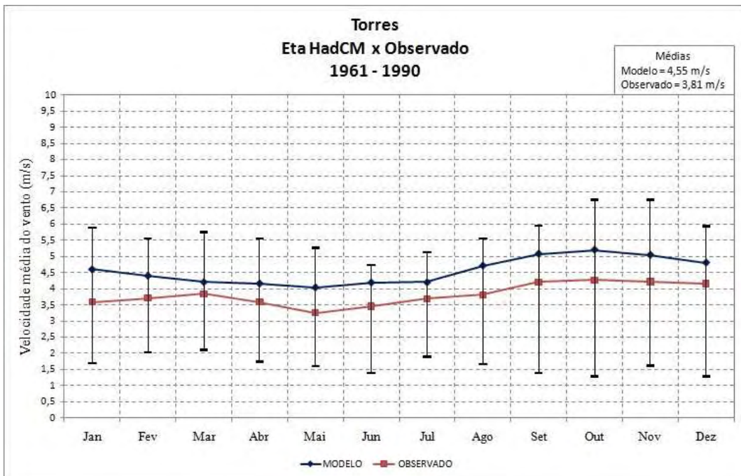
Figura 5.12 – Ciclo anual da velocidade do vento a 10 metros do modelo Eta HadCM e observações para a estação de Torres no período de 1961 a 1990.
