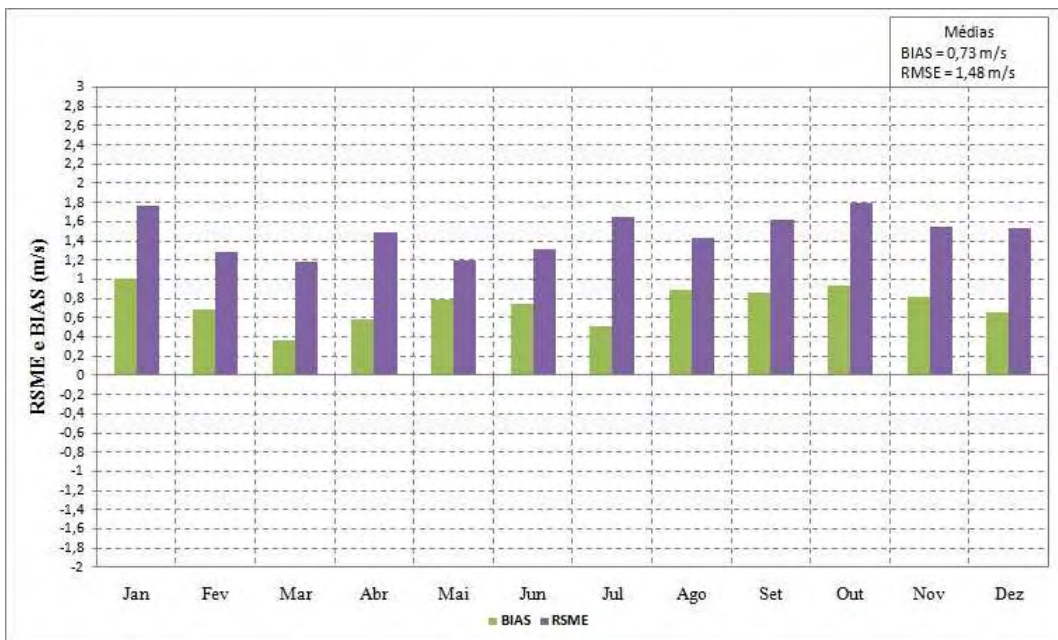
Figura 5.13 – RMSE e BIAS obtidos a partir do ciclo anual da velocidade do vento modelo Eta HadCM e observações para a estação de Torres no período de 1961 a 1990.
