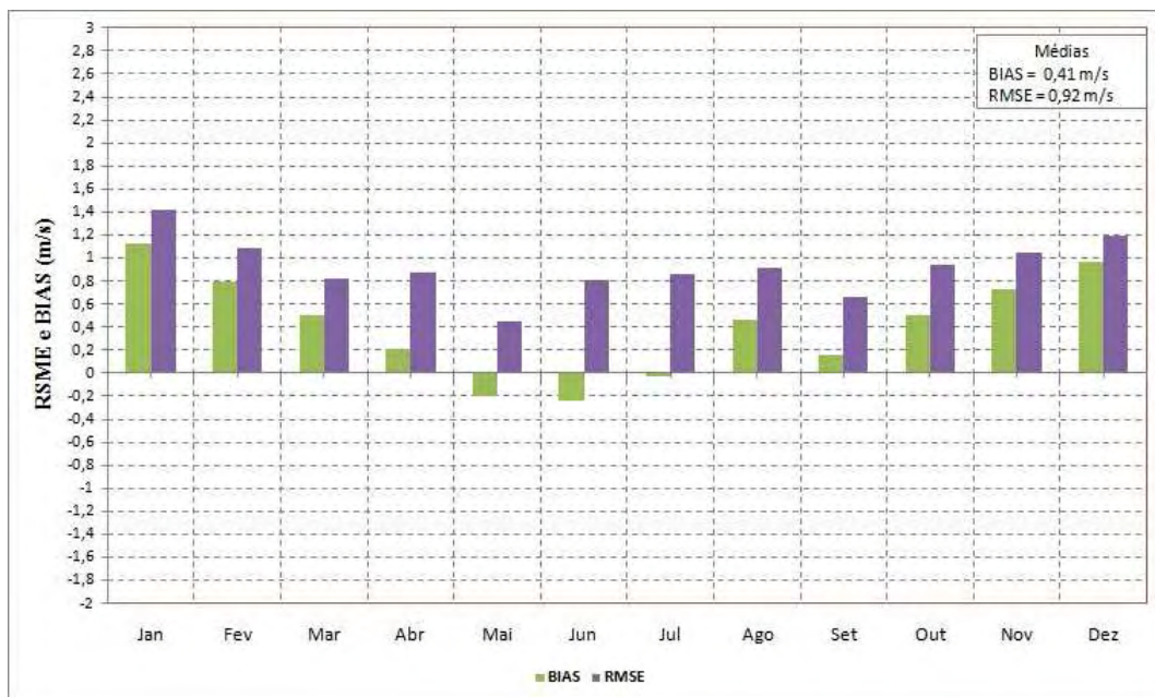
Figura 5.21 – RMSE e BIAS obtidos a partir do ciclo anual da velocidade do vento modelo Eta HadCM e reanálises ERA-40 para o período atual de Mostardas.
