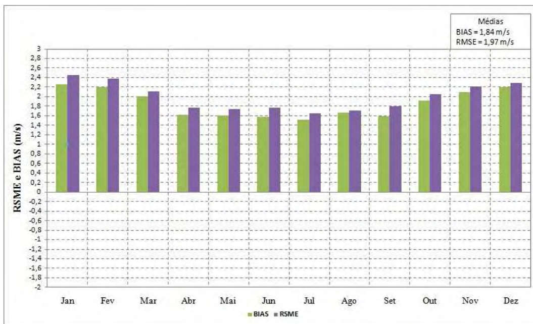
Figura 5.9 – RMSE e BIAS obtidos a partir do ciclo anual da velocidade do vento modelo Eta HadCM e observações para a estação de Rio Grande no período de 1960 a 1990.
