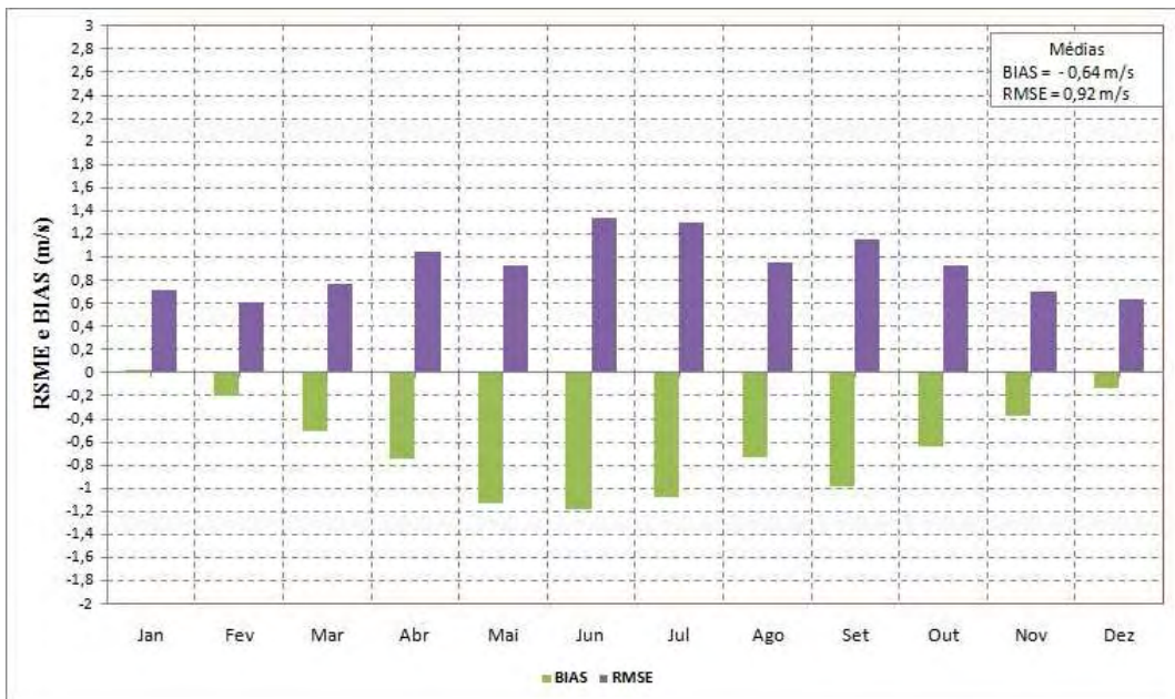
Figura 5.23 – RMSE e BIAS obtidos a partir do ciclo anual da velocidade do vento modelo Eta HadCM e reanálises ERA-40 para o período atual de Rio Grande.
