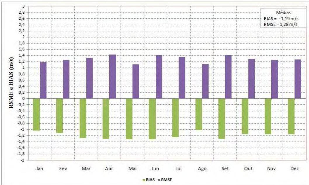
Figura 5.25 – RMSE e BIAS obtidos a partir do ciclo anual da velocidade do vento modelo Eta HadCM e reanálises ERA-40 para o período atual de Porto Alegre.
