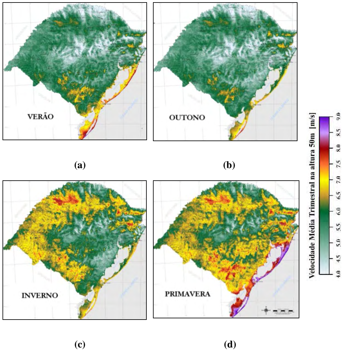
Figura 3.3 – Variação sazonal da velocidade média do vento no Rio Grande do Sul.
