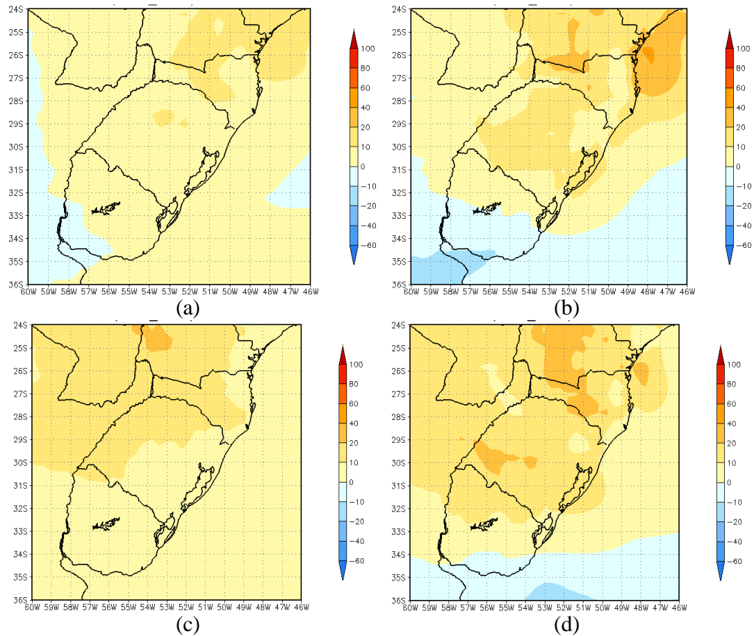
Figura 5.40 – Variação sazonal em porcentagem da densidade de potência do vento ao nível de 10 metros para os dois períodos do Cenário A1B em relação ao período atual, para inverno e primavera. (a) JJA, A1B (2010-2040) menos Referência; (b) JJA, A1B (2070-2100) menos Referência; (c) SON, A1B (2010-2040) menos Referência; (d) SON, A1B (2070-2100) menos Referência.
