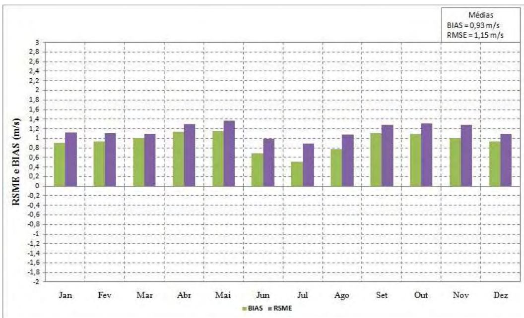
Figura 5.15 – RMSE e BIAS obtidos a partir do ciclo anual da velocidade do vento modelo Eta HadCM e observações para a estação de Santa Maria no período de 1960 a 1990.
