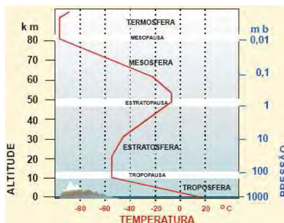
Figura 2.1 – Perfil vertical da atmosfera determinado pela variação da temperatura em função da altitude. No eixo direito, a variação da pressão atmosférica em função da altura.
