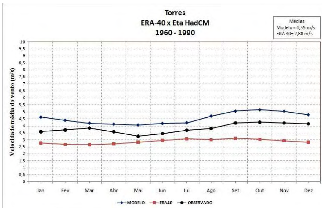
Figura 5.26 – Ciclo anual da velocidade do vento a 10 metros do modelo Eta HadCM e reanálises ERA-40 para o período atual de Torres.
