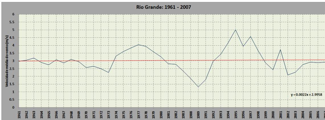
Gráfico de tendência da série observacional da estação de Rio Grande
