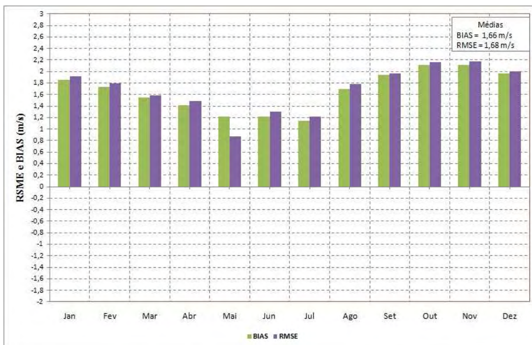
Figura 5.27 – RMSE e BIAS obtidos a partir do ciclo anual da velocidade do vento modelo Eta HadCM e reanálises ERA-40 para o período atual de Torres.
