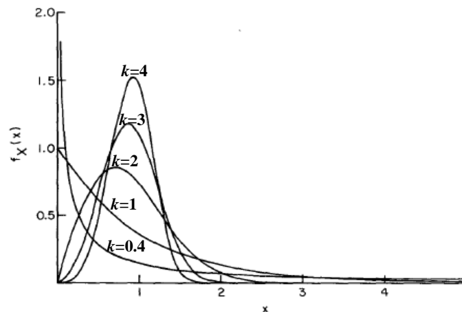
Figura 2.12 – Distribuição de Weibull para diferentes fatores de forma. Fonte: Adaptado de Hennessey (1977).
