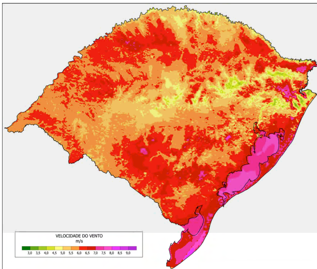
Figura 3.4 – Velocidade média anual do vento para o estado do Rio Grande do Sul.
