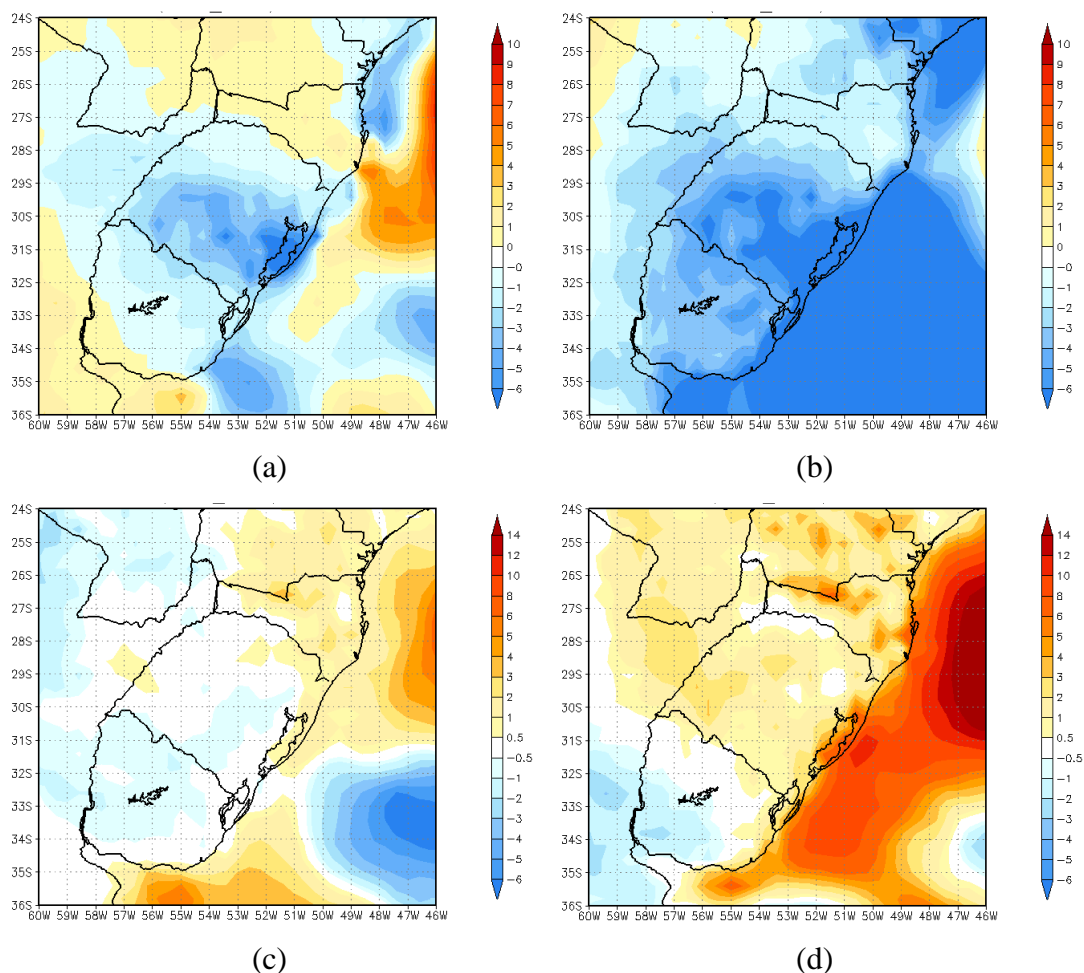
Figura 5.37 – Variação sazonal da densidade média de potência ao nível de 10 metros para os períodos do Cenário A1B em relação ao período atual; (a) DJF, A1B (2010-2040) menos Referência; (b) DJF, A1B (2070-2100) menos Referência; (c) MAM, A1B (2010-2040) menos Referência; (d) MAM, A1B (2070-2100) menos Referência.
