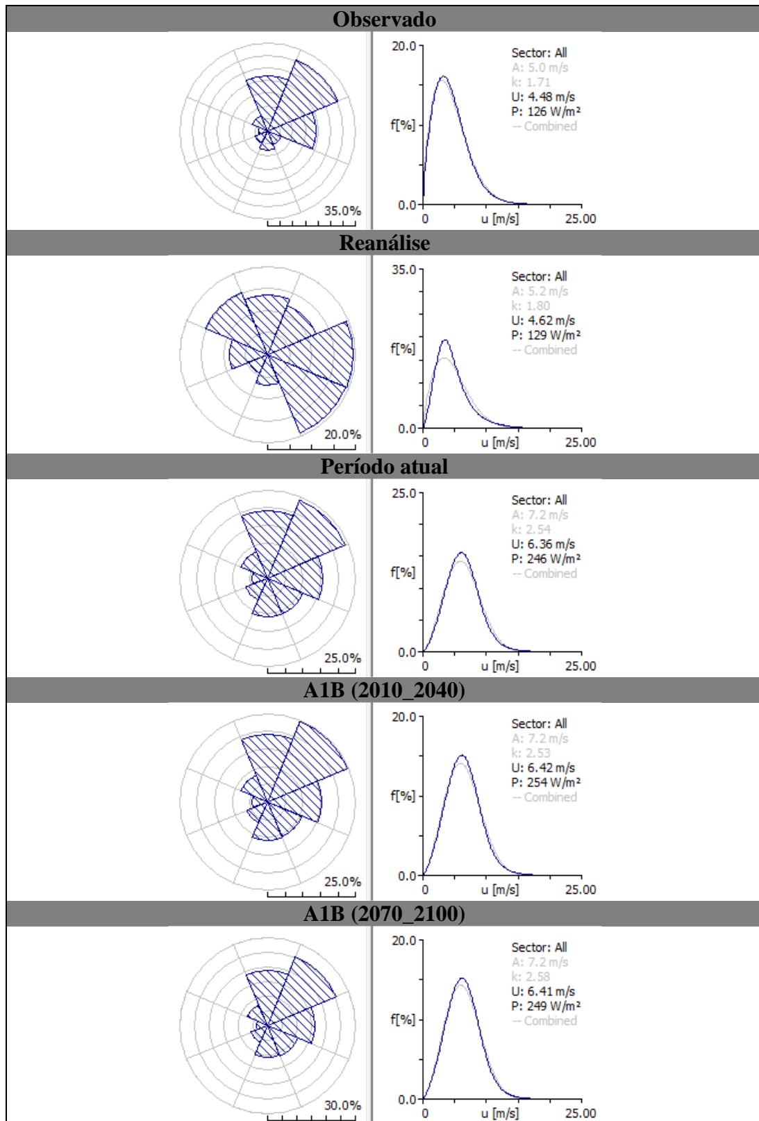
Histograma com direção e distribuição de Weibull para a estação de Torres (Lat 029°21'S / Lon 049°43' W).
