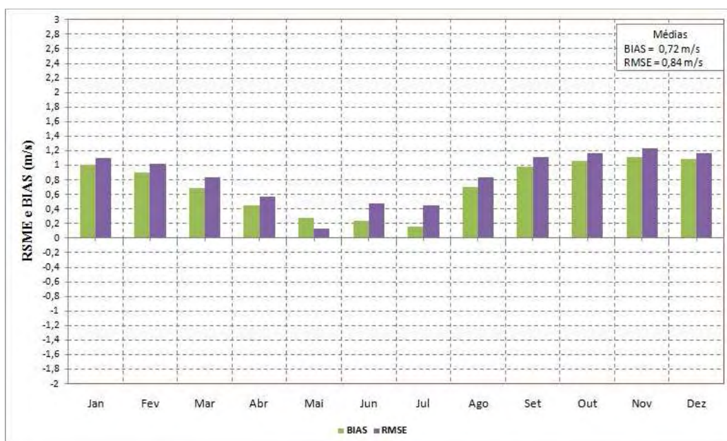
Figura 5.29 – RMSE e BIAS obtidos a partir do ciclo anual da velocidade do vento modelo Eta HadCM e reanálises ERA-40 para o período atual de Santa Maria.
