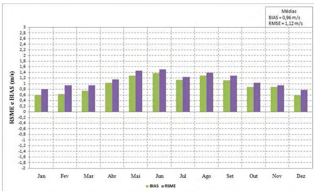
Figura 5.11 – RMSE e BIAS obtidos a partir do ciclo anual da velocidade do vento modelo Eta HadCM e observações para a estação de Porto Alegre no período de 1960 a 1990.
