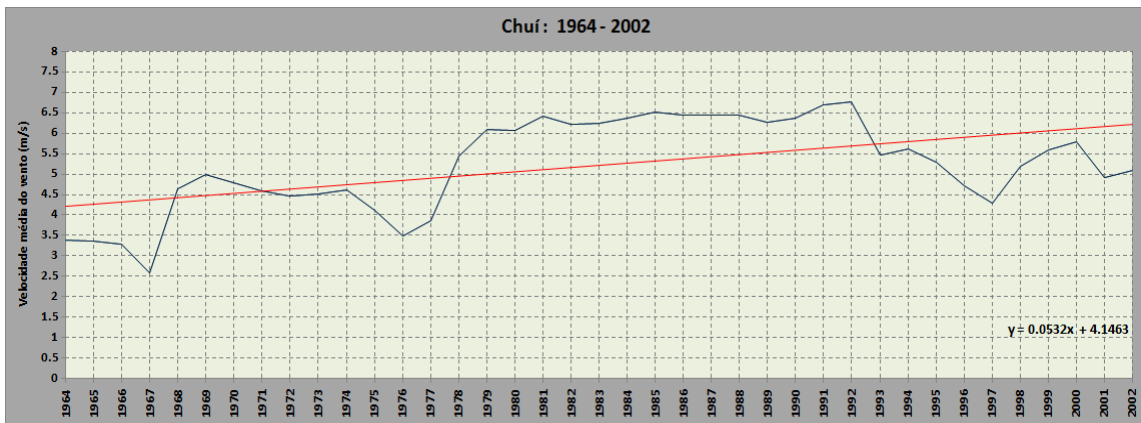
Gráfico de tendência da série observacional da estação de Chuí
