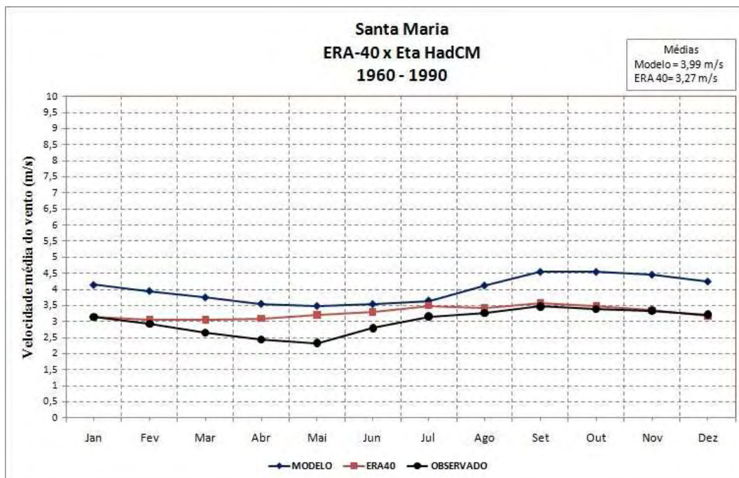
Figura 5.28 – Ciclo anual da velocidade do vento a 10 metros do modelo Eta HadCM e reanálises ERA-40 para o período atual de Santa Maria.
