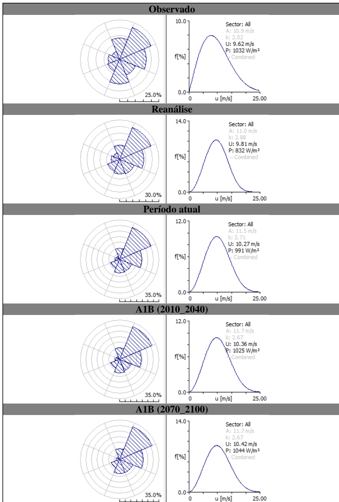
Histograma com direção e distribuição de Weibull para a estação de Mostardas (Lat 31°14'52"S / Lon 050°54'24"W).
