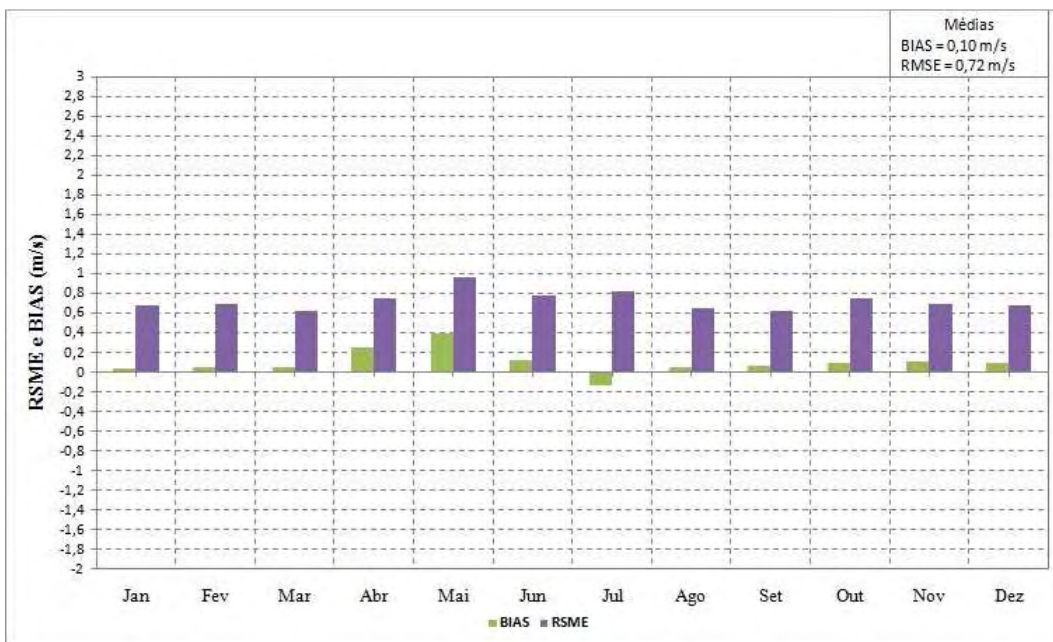
Figura 5.17 – RMSE e BIAS obtidos a partir do ciclo anual da velocidade do vento modelo Eta HadCM e observações para a estação de Uruguaiiana no período de 1960 a 1990.
