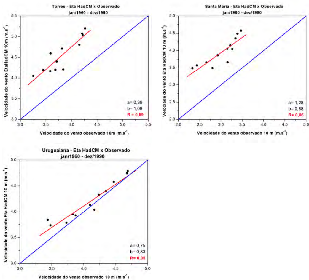
Figura 5.3 – Diagrama de dispersão das médias mensais da velocidade do vento a 10 metros para as estações de Santa Maria, Torres e Uruguaiiana.
