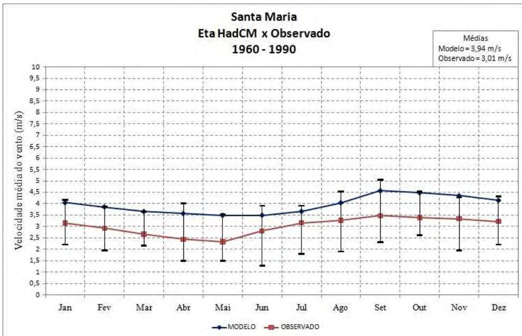
Figura 5.14 – Ciclo anual da velocidade do vento a 10 metros do modelo Eta HadCM e observações para a estação de Santa Maria no período de 1960 a 1990.
