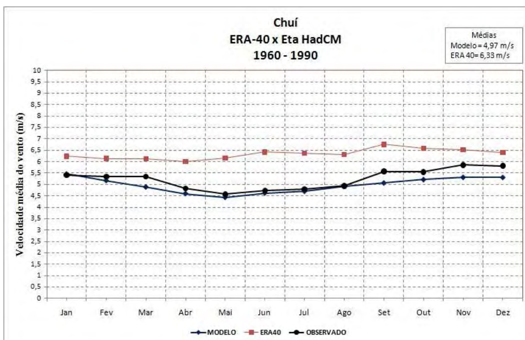
Figura 5.18 – Ciclo anual da velocidade do vento a 10 metros do modelo Eta HadCM e reanálises ERA-40 para o período atual de Chuí.
