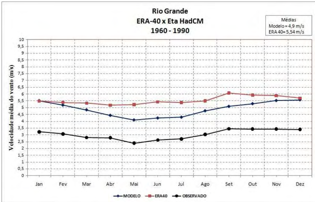
Figura 5.22 – Ciclo anual da velocidade do vento a 10 metros do modelo Eta HadCM e reanálises ERA-40 para o período atual de Rio Grande.
