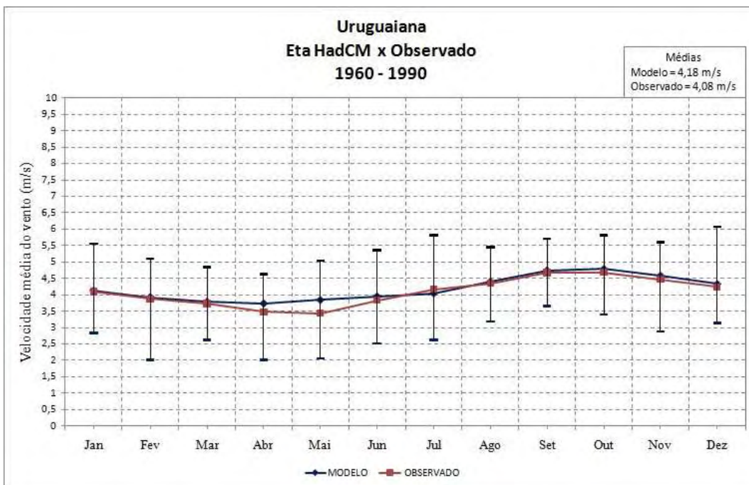
Figura 5.16 – Ciclo anual da velocidade do vento a 10 metros do modelo Eta HadCM e observações para a estação de Uruguaiiana no período de 1960 a 1990.
