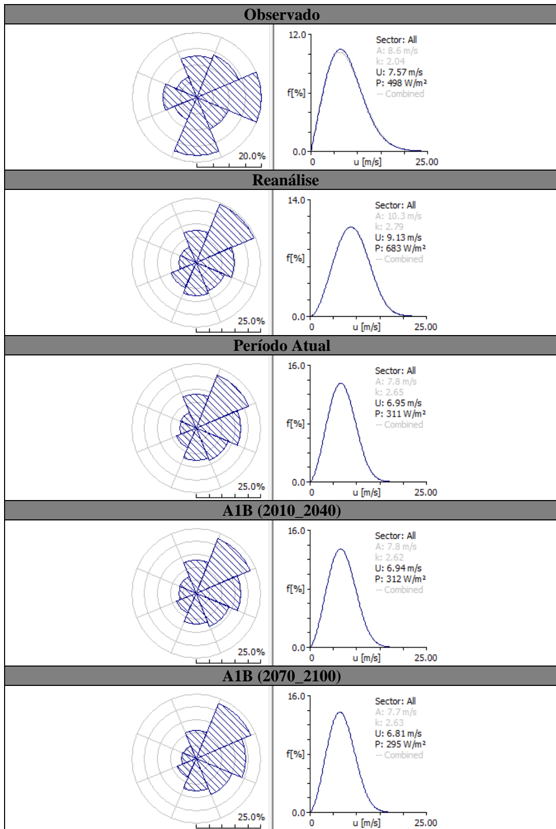
Histograma com direção e distribuição de Weibull para a estação de Chuí (Lat 33°44'30"S / Lon 053°22'18"W).
