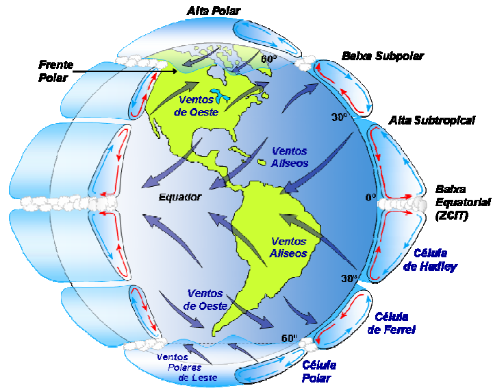
Figura 2.4 – Modelo da circulação global atmosférica, indicando a estrutura vertical das células de circulação e os ventos próximos à superfície. A relação entre o tamanho da atmosfera e da Terra está ampliada para facilitar a visualização. Fonte: Adaptado de Lutgens e Tarbuck, 1995.
