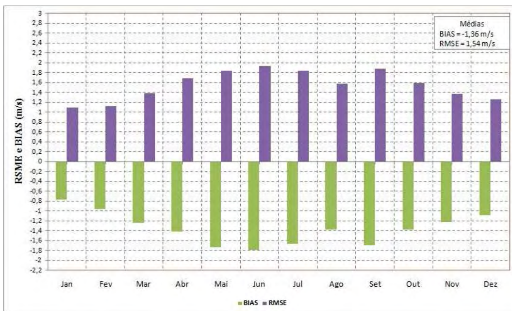
Figura 5.19 – RMSE e BIAS obtidos a partir do ciclo anual da velocidade do vento modelo Eta HadCM e reanálises ERA-40 para o período atual de Chuí.
