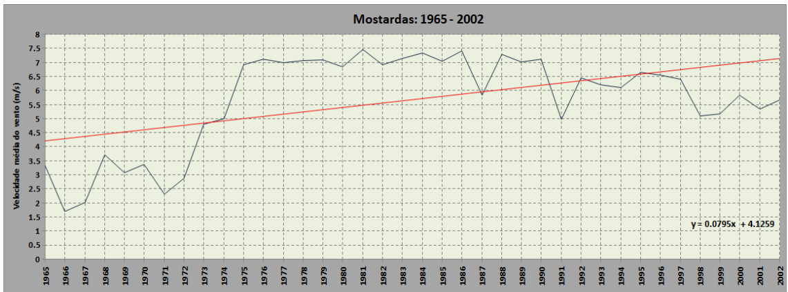
Gráfico de tendência da série observacional da estação de Mostardas
