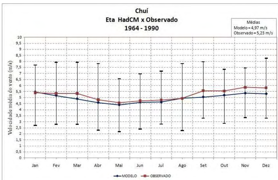
Figura 5.4 – Ciclo anual da velocidade do vento a 10 metros do modelo Eta HadCM e observações para a estação de Chuí no período de 1964 a 1990.
