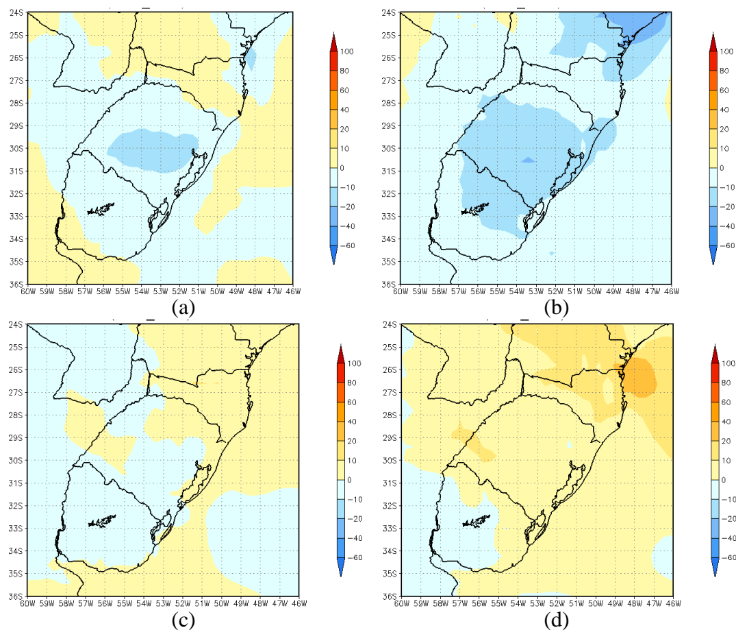
Figura 5.39 – Variação sazonal em porcentagem de densidade de potência do vento ao nível de 10 metros para os dois períodos do Cenário A1B em relação ao período atual. (a) DJF, A1B (2010-2040) menos Referência; (b) DJF, A1B (2070-2100) menos Referência; (c) MAM, A1B (2010-2040) menos Referência; (d) MAM, A1B (2070-2100) menos Referência.
