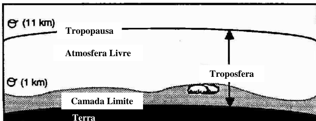
Figura 2.2 – Representação da Camada Limite Atmosférica (boundary layer) e da Atmosfera Livre.
