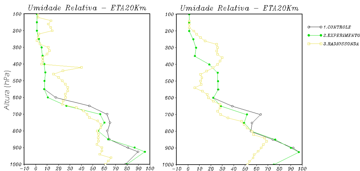
Figura 5.32 - Perfil Vertical da Umidade Relativa para OP24. Radiossondagem (amarelo), ETA incluindo radiossondagens (EXP) (verde) e sem radiossondagens CTL (preto). À esquerda para o dia 28/10/2005 às 06 UTC. A direita para o dia 28/10/2005 às 12 UTC.
