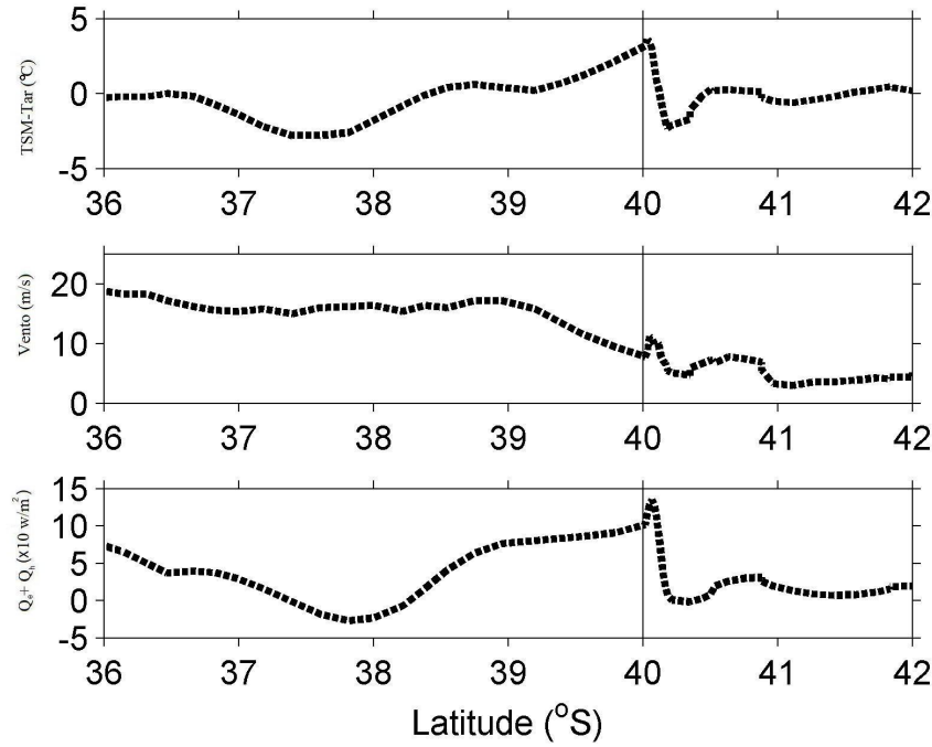
Figura 4.13 - No painel superior tem-se o parâmetro de estabilidade dado pela TSM-Tar ( ^{\circ}C ). No painel central, a velocidade do vento ( m/s ). No painel inferior os fluxos de calor sensível mais o fluxo de calor latente \times (10W/m^2) . Todos os dados são amostrados ao longo das trajetórias do NApOc Ary Rongel enquanto cruzava a região da CBM. A frente oceanográfica entre a CB (quente) e CM (fria) na OP23 se localiza em cerca de 40^{\circ}S .
