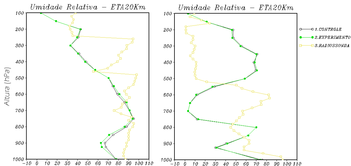
Figura 5.33 - Perfil Vertical da Umidade Relativa para OP26. Radiossondagem (amarelo), ETA incluindo radiossondagens (EXP) (verde) e sem radiossondagens CTL (preto). À esquerda para o dia 16/10/2007 às 06 UTC. A direita para o dia 16/10/2007 às 12 UTC.
