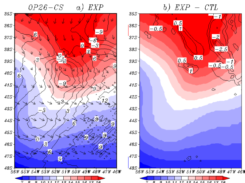
Figura 5.24 - TSM (escala sombreada) em ( ^{\circ}\text{C} ), o fluxo de Calor Sensível (linhas de contorno) em ( \text{W}/\text{m}^2 ) e o Vento em superfície (vetores) em ( \text{m}/\text{s} ). Para OP26 no período de 16/10/2007 às 12 UTC utilizando uma média de três dias. Painel a) Experimento EXP. Painel b) EXP - CTL, para o Calor Sensível.
