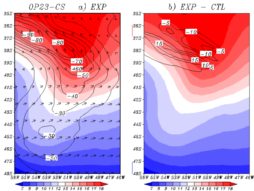
Figura 5.22 - TSM (escala sombreada) em ^{\circ}\text{C} , o fluxo de Calor Sensível (linhas de contorno) em \text{W}/\text{m}^2 e o Vento em superfície (vetores) em \text{m}/\text{s} . Para OP23 no período de 03/11/2004 às 12 UTC utilizando uma média de três dias. Painei a) Experimento EXP. Painei b) EXP - CTL, para o Calor Sensível.
