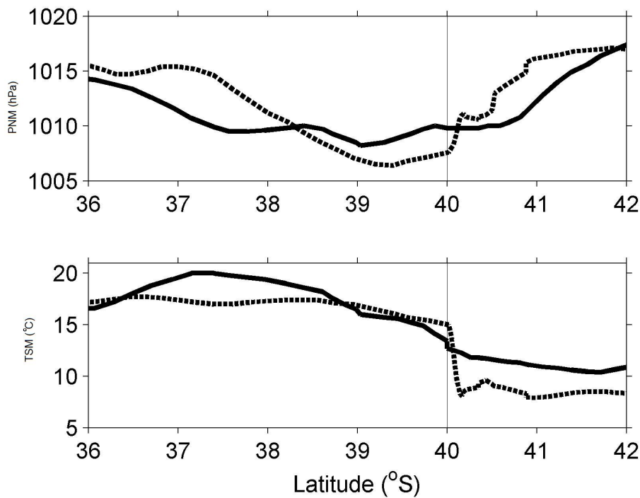
Figura 4.17 - Na parte superior tem-se a Pressão ao nível do mar ( \text{hPa} ) e abaixo a TSM ( ^{\circ}\text{C} ), para OP23 (linha pontilhada) e OP24 (linha contínua).
