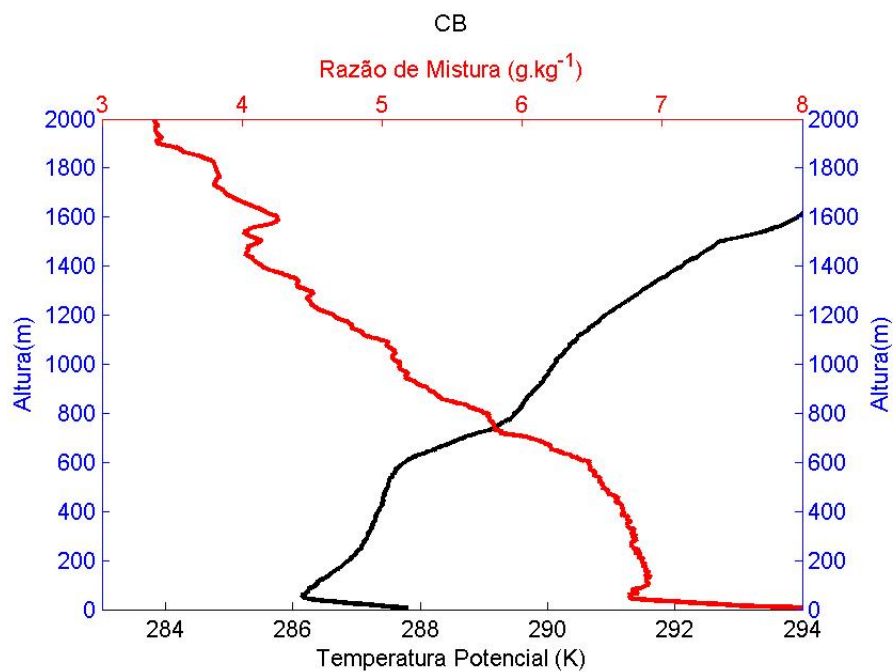
Figura 4.9 - Média da Altura da CLA na região da CB.
