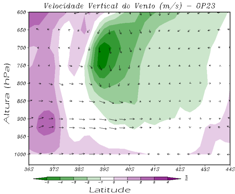
Figura 5.13 - Para OP23 no período de 03/11/2004 utilizando uma média entre os horários das 06 e 12 UTC. Velocidade Vertical do Vento ( \text{m/s} ) em cores, sobrepostos a circulação meridional do vento ( \text{m/s} ), ambos ( \times por 10^2 ). Uma média entre as longitudes 54^\circ\text{W} e 50^\circ\text{W} foi feita para o corte meridional, no qual a frente estava bem definida.
