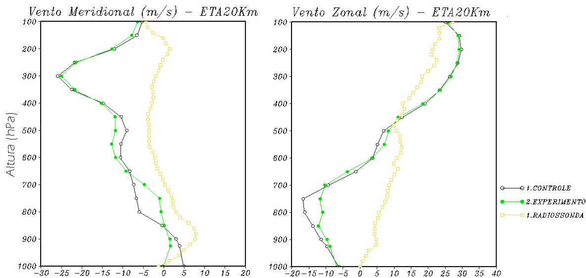
Figura 5.34 - Perfil Vertical do Vento Meridional (esquerda) e Zonal (direita) para OP23. Radiossondagem (amarelo), ETA incluindo radiossondagens (EXP) (verde) e sem radiossondagens CTL (preto). Para o dia 03/11/2004 às 06 UTC.
