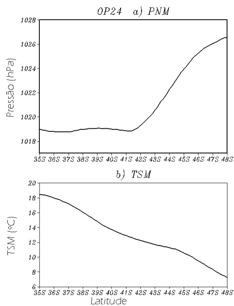
Figura 5.17 - Para OP24 no período de 28/10/2005 às 12 UTC utilizando uma média de três dias. Painei a) PNM em (h/Pa). Painei b) TSM em (°C). Para o corte meridional uma média entre as longitudes 55 °W e 51 °W foi realizada.
