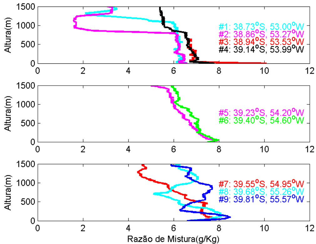
Figura 4.12 - Perfil Vertical da Umidade ( g/kg ). Medidas através de radiossondas nos dias 27 e 28 de outubro de 2006.
