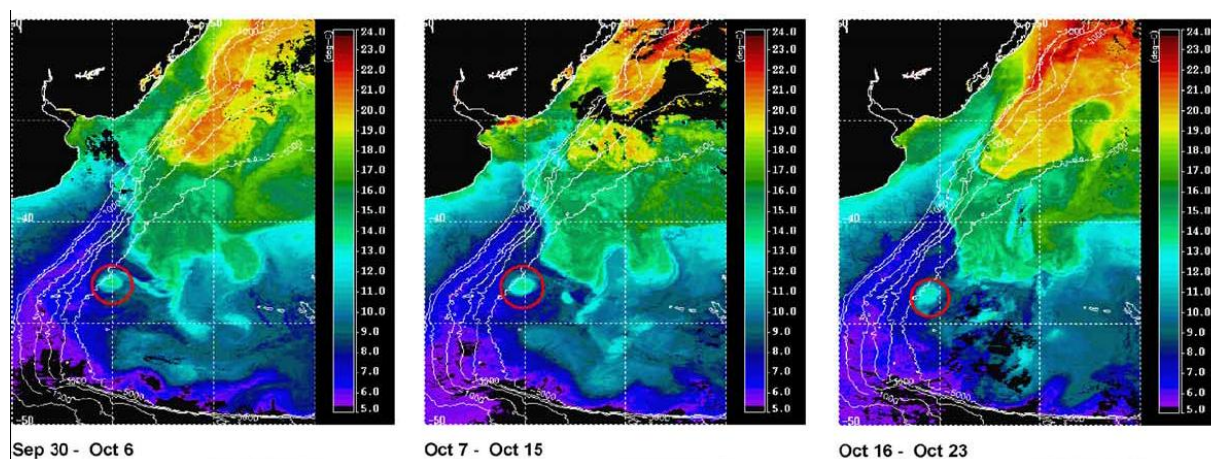
Figura 2.3 - TSM ( ^{\circ}\text{C} ) através de imagem de satélite, onde o vórtice está indicado por um círculo vermelho.
