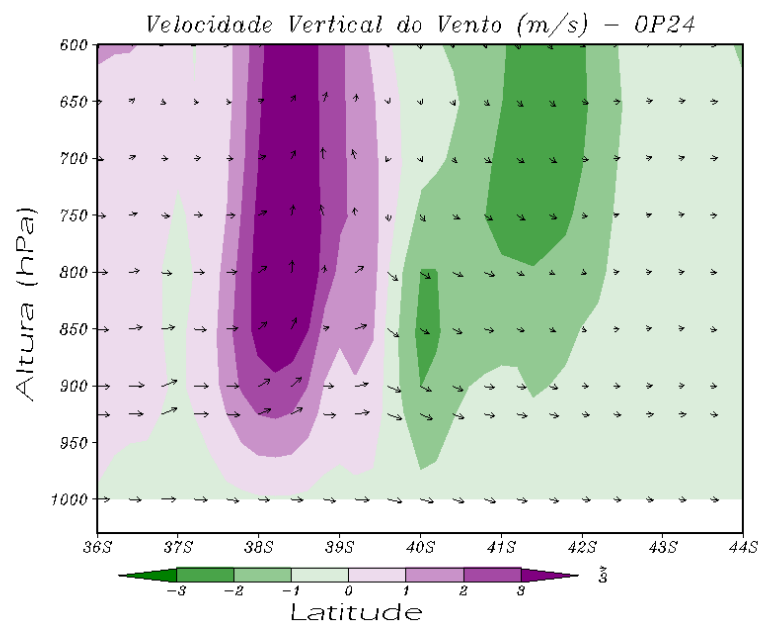
Figura 5.14 - Para OP24 no período de 28/10/2005 utilizando uma média entre os horários das 06 e 12 UTC. Velocidade Vertical do Vento (m/s) em cores, sobrepostos a circulação meridional do vento (m/s), ambos ( \times por 10^2 ). Uma média entre as longitudes 54^\circ\text{W} e 50^\circ\text{W} foi feita para o corte meridional, no qual a frente estava bem definida.
