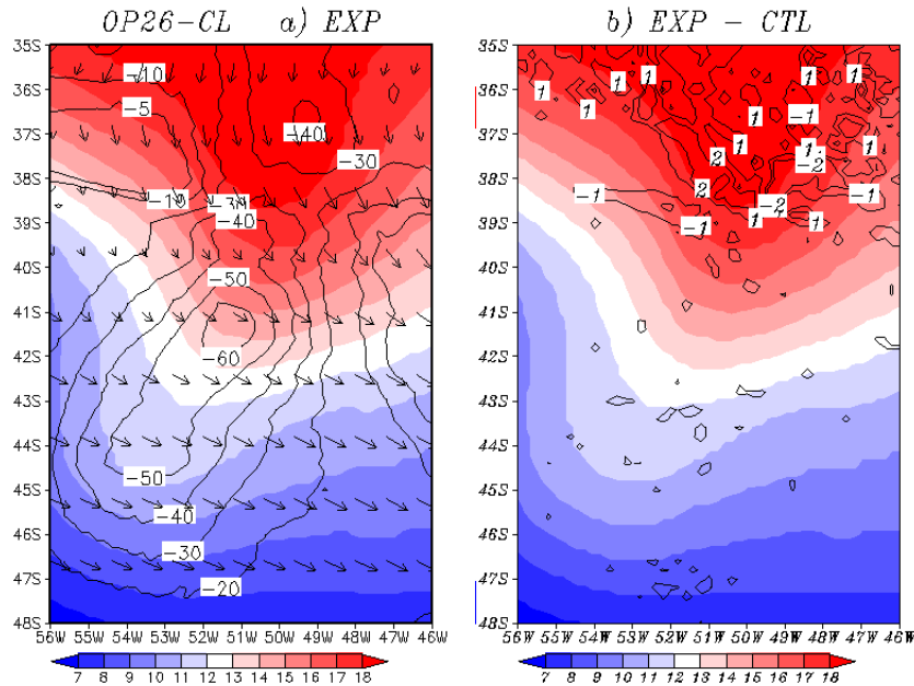
Figura 5.21 - TSM (escala sombreada) em ( ^{\circ}\text{C} ), o fluxo de Calor Latente (linhas de contorno) em ( \text{W}/\text{m}^2 ) e o Vento em superfície (vetores) em ( \text{m}/\text{s} ). Para OP26 no período de 16/10/2007 às 12 UTC utilizando uma média de três dias. Painei a) Experimento EXP. Painei b) EXP - CTL, para o Calor Latente.
