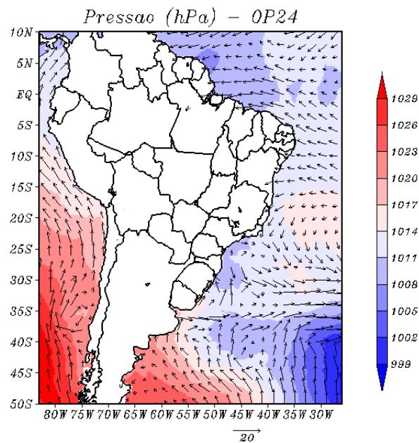
Figura 5.5 - Campo de pressão ao nível do mar ( hPa ) em cores e vento em superfície ( m/s ). Para OP24 no período 28/10/2005 utilizando uma média entre os horários das 06 e 12 UTC.
