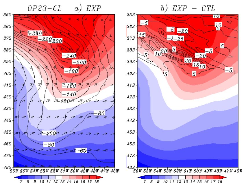
Figura 5.19 - TSM (escala sombreada) em ( ^{\circ}\text{C} ), o fluxo de Calor Latente (linhas de contorno) em ( \text{W}/\text{m}^2 ) e o Vento em superfície (vetores) em ( \text{m}/\text{s} ). Para OP23 no período de 03/11/2004 às 12 UTC utilizando uma média de três dias. Painel a) Experimento EXP. Painel b) EXP - CTL, para o Calor Latente.
