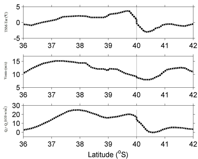
Figura 4.14 - A frente oceanográfica entre a CB (quente) e CM (fria) na OP24 se localiza em cerca de 40°S.
