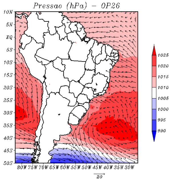
Figura 5.6 - Campo de pressão ao nível do mar ( hPa ) em cores e vento em superfície ( m/s ). Para OP26 no período 16/10/2007 utilizando uma média entre os horários das 06 e 12 UTC.
