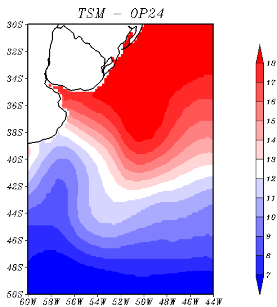
Figura 5.8 - Campo de TSM ( ^{\circ}\text{C} ). Para OP24 no período 28/10/2005 utilizando uma média entre os horários das 06 e 12 UTC.
