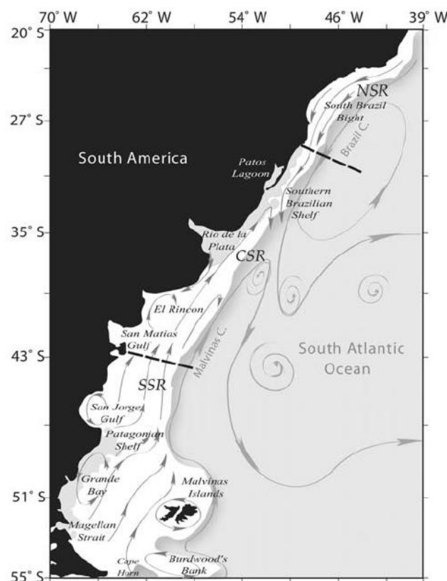
Figura 2.2 - Encontro da CB com a CM, indicando a região da CBM.
