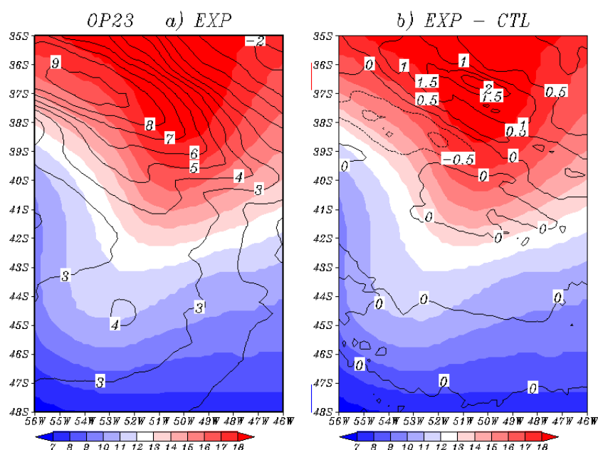
Figura 5.26 - TSM (escala sombreada) em ( ^{\circ}\text{C} ), o Vento Meridional (linhas de contorno) em ( \text{m/s} ). Para OP23 no período de 03/11/2004 às 12 UTC utilizando uma média de três dias. Painel a) Experimento EXP. Painel b) EXP - CTL.
