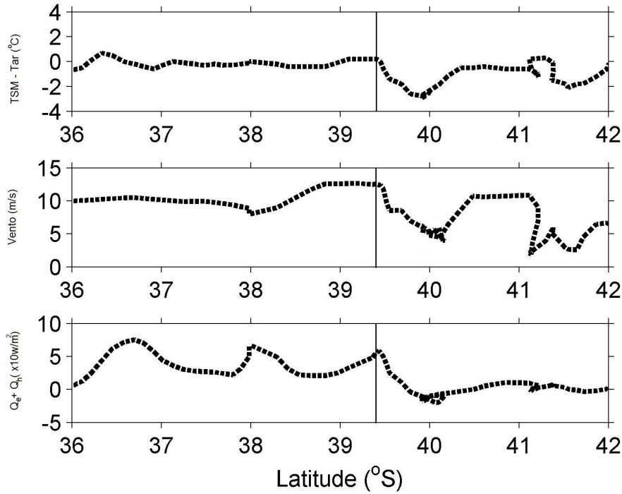
Figura 4.16 - A frente oceanográfica entre a CB (quente) e CM (fria) na OP26 se localiza em cerca de 39.5^{\circ}S .
