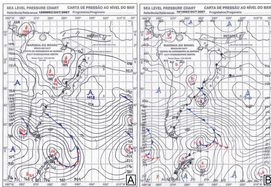
Figura 4.4 - Carta sinótica de pressão ao nível do mar. Painel A: dia 16 de outubro de 2007 no horário das 00 UTC. Painel B: dia 16 de outubro de 2007 no horário das 12 UTC.
