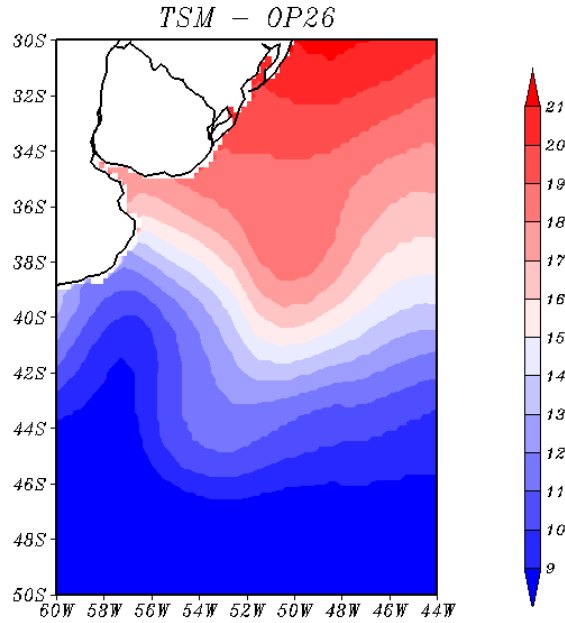
Figura 5.9 - Campo de TSM ( ^{\circ}\text{C} ). Para OP26 no período 16/10/2007 utilizando uma média entre os horários das 06 e 12 UTC.
