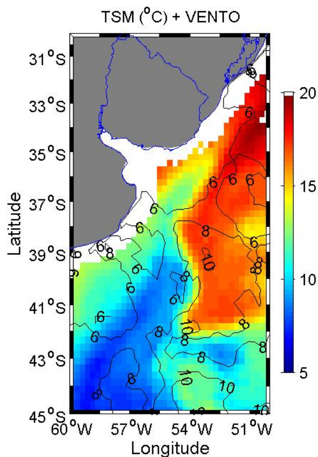
Figura 3.3 - Posicionamento da CBM com os dados de TSM (em cores) obtidas através do AMSR-E e vetores de vento à superfície, para o período da OP24.
