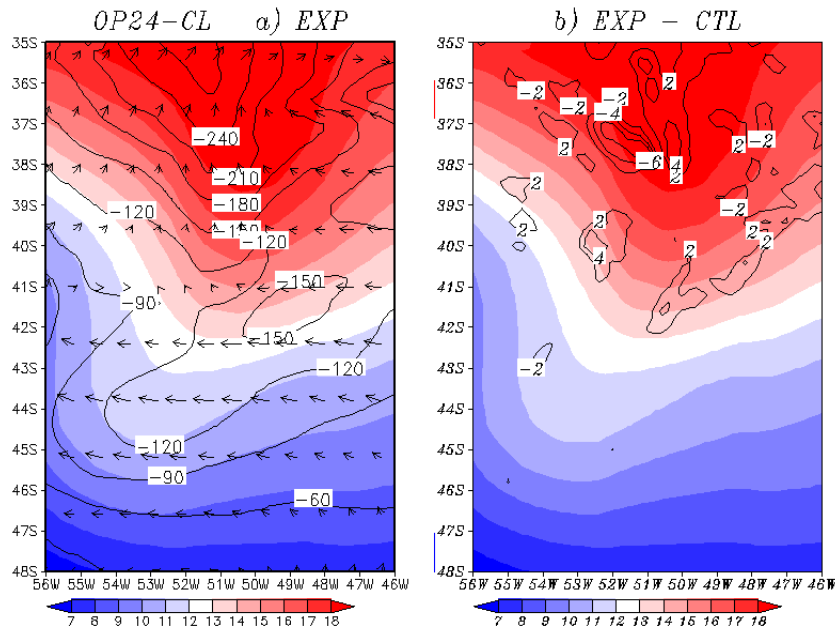
Figura 5.20 - TSM (escala sombreada) em ( ^{\circ}\text{C} ), o fluxo de Calor Latente (linhas de contorno) em ( \text{W/m}^2 ) e o Vento em superfície (vetores) em ( \text{m/s} ). Para OP24 no período de 28/10/2005 às 12 UTC utilizando uma média de três dias. Painel a) Experimento EXP. Painel b) EXP - CTL, para o Calor Latente.
