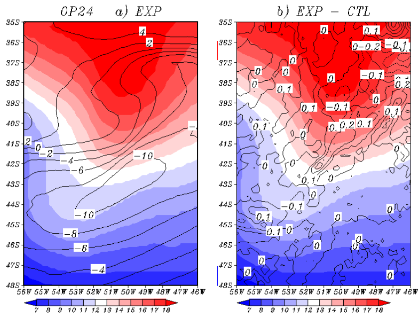
Figura 5.27 - TSM (escala sombreada) em ( ^{\circ}\text{C} ), o Vento Zonal (linhas de contorno) em ( \text{m/s} ). Para OP24 no período de 28/10/2005 às 12 UTC utilizando uma média de três dias. Painel a) Experimento EXP. Painel b) EXP - CTL.
