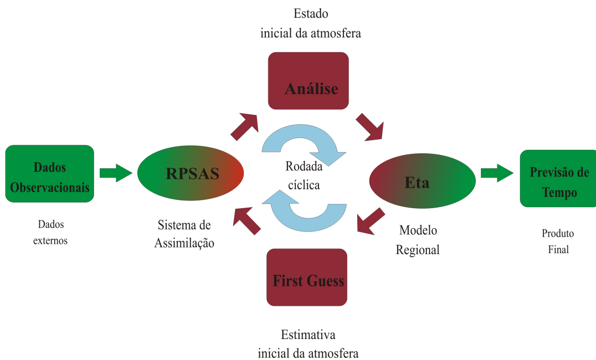
Figura 3.4 - Diagrama ilustrativo do fluxo de dados em uma rodada cíclica na versão regional do modelo PNT do CPTEC.
