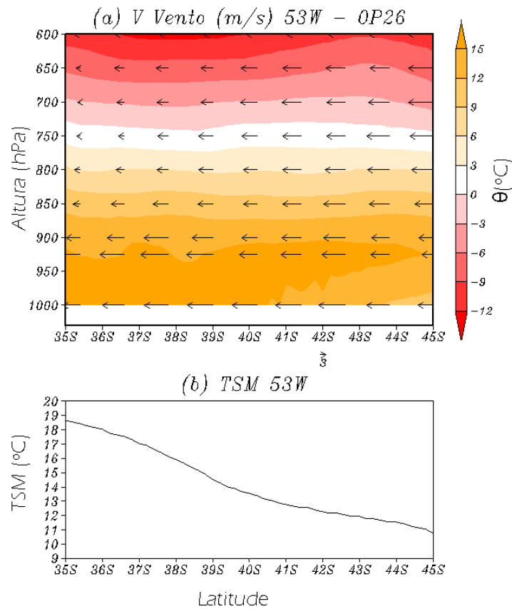
Figura 5.12 - Para OP26: Painel (a) componente meridional do vento ( V ) em m/s e da temperatura potencial ( \theta ) em ^{\circ}C , em 53^{\circ}W . Painel (b) Valor médio de TSM ( ^{\circ}C ).
