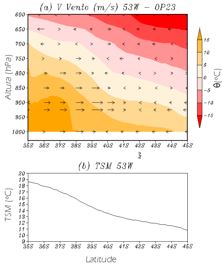
Figura 5.10 - Para OP23: Painei (a) componente meridional do vento ( V ) em m/s e da temperatura potencial ( \theta ) em °C, em 53°W. Painei (b) Valor médio de TSM (°C).
