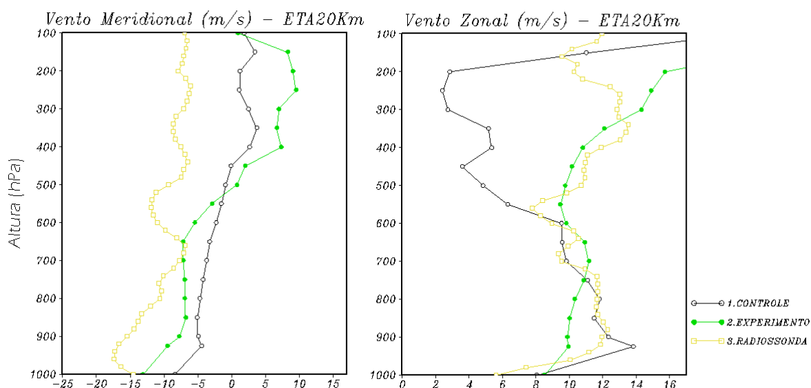
Figura 5.36 - Perfil Vertical do Vento Meridional (esquerda) e Zonal (direita) para OP26. Radiossondagem (amarelo), ETA incluindo radiossondagens (EXP) (verde) e sem radiossondagens CTL (preto). Para o dia 16/10/2007 às 12 UTC.
