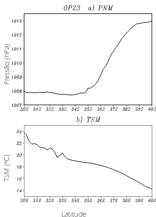
Figura 5.16 - Para OP23 no período de 03/11/2004 às 12 UTC utilizando uma média de três dias. Paineis a) PNM em (hPa). Paineis b) TSM em (°C). Para o corte meridional uma média entre as longitudes 55°W e 51°W foi realizada.
