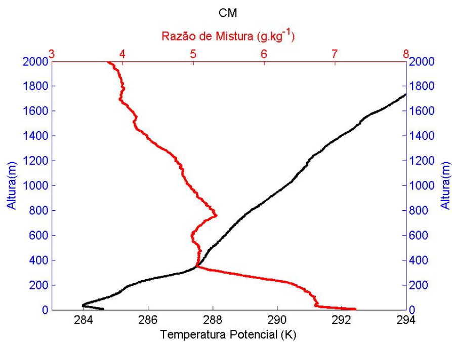
Figura 4.10 - Média da Altura da CLA na região da CM.
