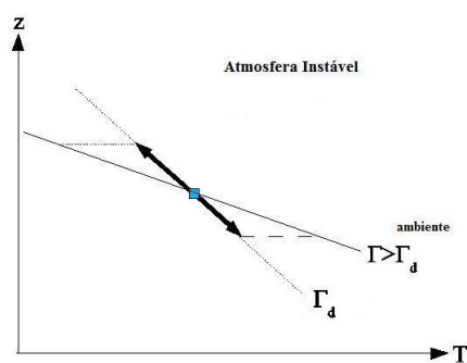
Figura 2.7 - Atmosfera instável.
