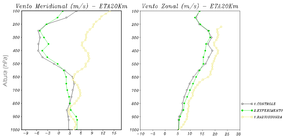
Figura 5.35 - Perfil Vertical do Vento Meridional (esquerda) e Zonal (direita) para OP24. Radiossondagem (amarelo), ETA incluindo radiossondagens (EXP) (verde) e sem radiossondagens CTL (preto). Para o dia 28/10/2005 às 12 UTC.
