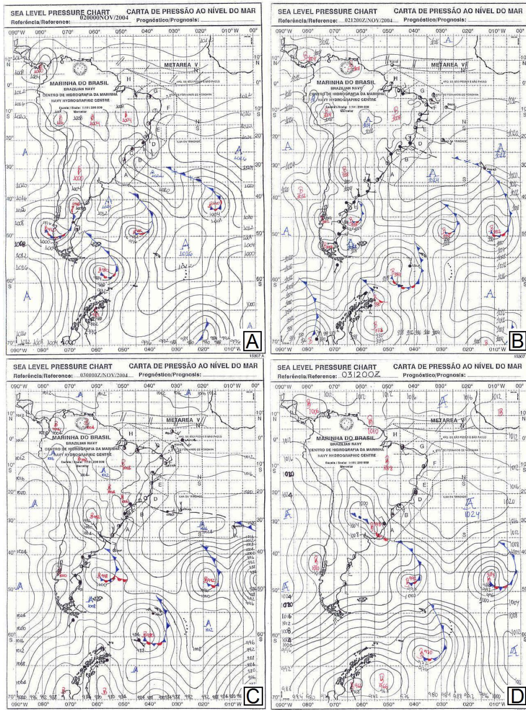
Figura 4.1 - Carta sinótica de pressão ao nível do mar. Painel A: dia 2 de novembro de 2004 no horário das 00 UTC. Painel B: dia 2 de novembro de 2004 no horário das 12 UTC. Painel C: dia 3 de novembro de 2004 no horário das 00 UTC. Painel D: dia 3 de novembro de 2004 no horário das 12 UTC.
