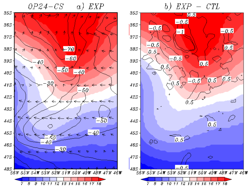
Figura 5.23 - O mesmo para OP24 no período de 28/10/2005.
