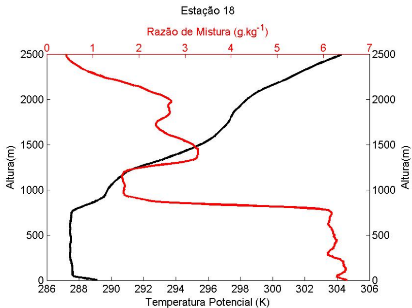
Figura 4.7 - Altura da CLA na região da CB, com a Temperatura Potencial Virtual e Razão de Mistura medidas através da radiossonda no dia 27 de outubro de 2006 às 13 UTC.
