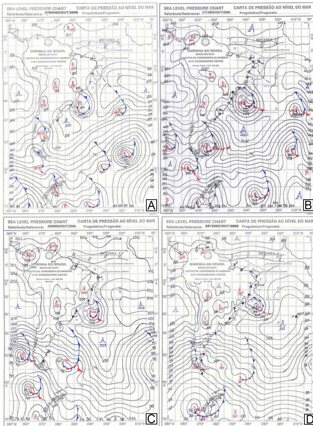
Figura 4.3 - Carta sinótica de pressão ao nível do mar. Painel A: dia 27 de outubro de 2006 no horário das 00 UTC. Painel B: dia 27 de outubro de 2006 no horário das 12 UTC. Painel C: dia 28 de outubro de 2006 no horário das 00 UTC. Painel D: dia 28 de outubro de 2006 no horário das 12 UTC.
