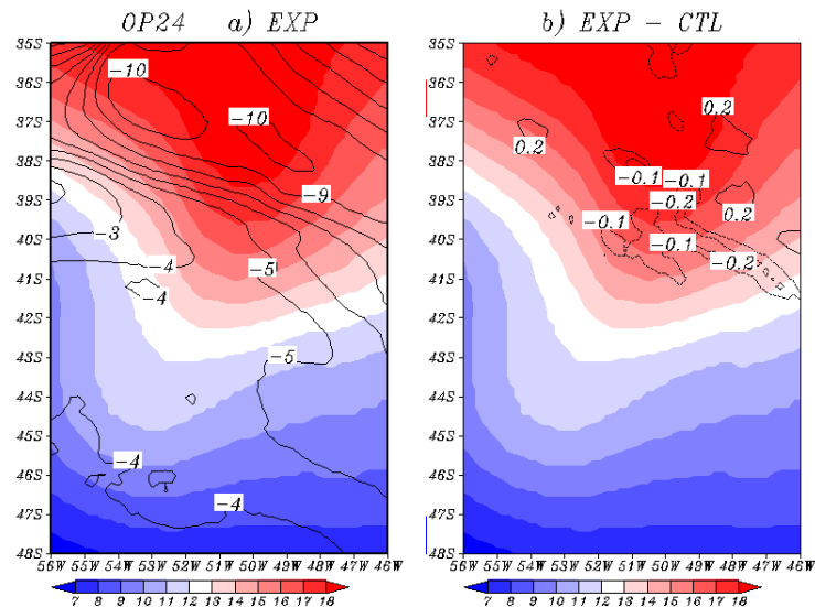
Figura 5.30 - TSM (escala sombreada) em ( ^{\circ}C ), o Vento Meridional (linhas de contorno) em ( m/s ). Para OP26 no período de 16/10/2007 às 12 UTC utilizando uma média de três dias. Painei a) Experimento EXP. Painei b) EXP - CTL.
