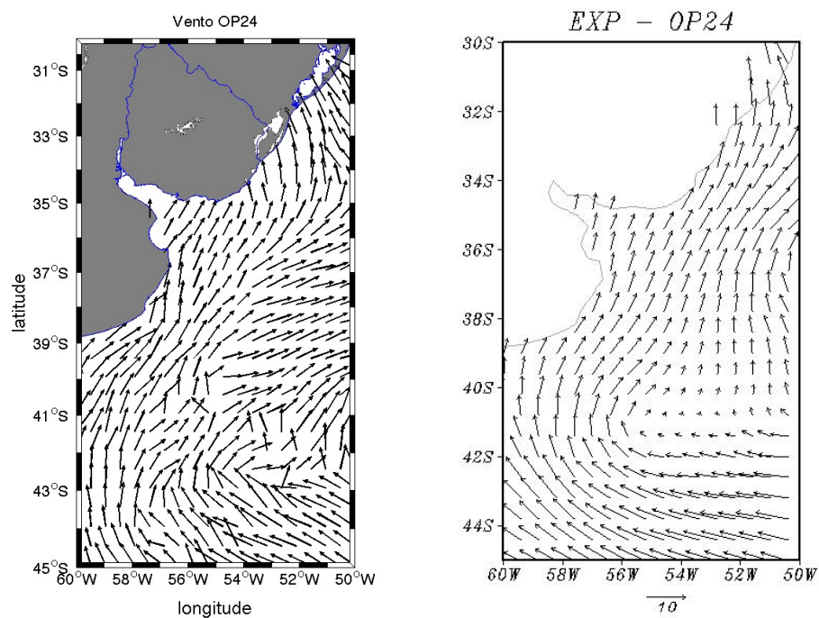
Figura 5.2 - Média de 3 dias centrada no dia 28 de outubro de 2005 (OP24).
