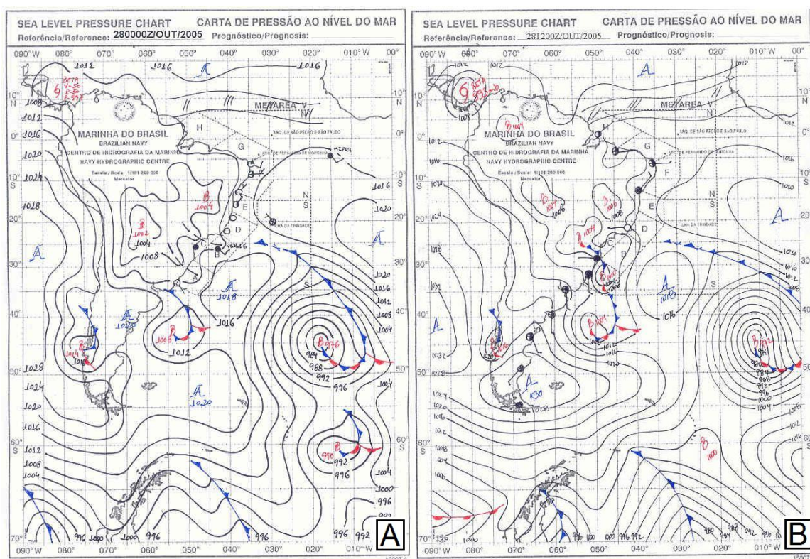
Figura 4.2 - Carta sinótica de pressão ao nível do mar. Painel A: dia 28 de outubro de 2005 no horário das 00 UTC. Painel B: dia 28 de outubro de 2005 no horário das 12 UTC.
