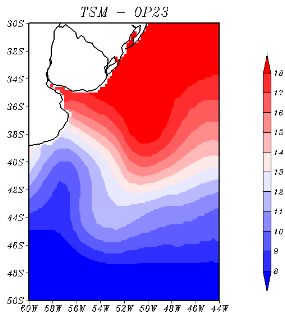
Figura 5.7 - Campo de TSM ( ^{\circ}\text{C} ). Para OP23 no período 03/11/2004 utilizando uma média entre os horários das 06 e 12 UTC.
