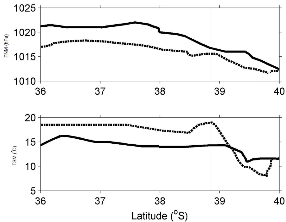
Figura 4.18 - Na parte superior tem-se a Pressão ao nível do mar ( hPa ) e abaixo a TSM ( ^{\circ}C ), para OP25 (linha pontilhada) e OP26 (linha contínua).
