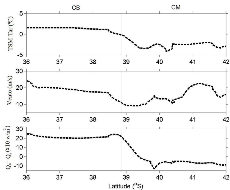
Figura 4.15 - A frente oceanográfica entre a CB (quente) e CM (fria) na OP25 se localiza em cerca de 39°S.
