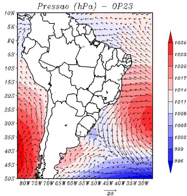
Figura 5.4 - Campo de pressão ao nível do mar ( hPa ) em cores e vento em superfície ( m/s ). Para OP23 no período 03/11/2004 utilizando uma média entre os horários das 06 e 12 UTC.
