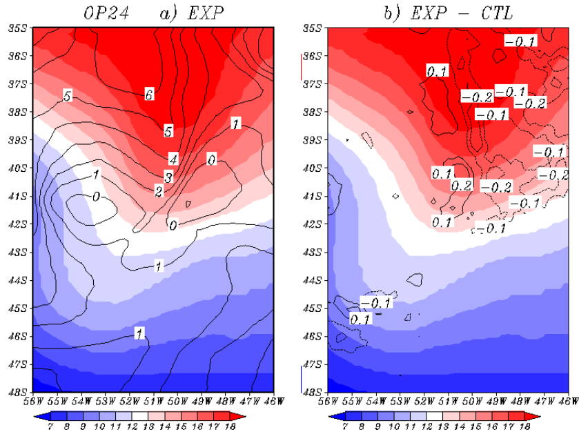
Figura 5.28 - TSM (escala sombreada) em ( ^{\circ}\text{C} ), o Vento Meridional (linhas de contorno) em ( \text{m/s} ). Para OP24 no período de 28/10/2005 às 12 UTC utilizando uma média de três dias. Painel a) Experimento EXP. Painel b) EXP - CTL.
