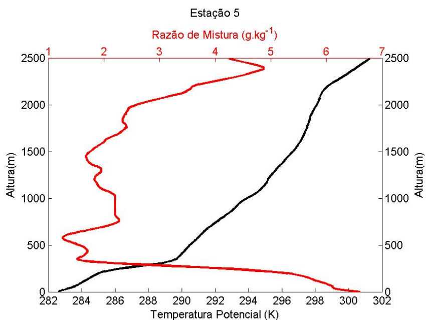
Figura 4.8 - Altura da CLA na região da CM, com a Temperatura Potencial Virtual e Razão de Mistura medidas através da radiossonda no dia 03 de novembro de 2004 às 05 UTC.
