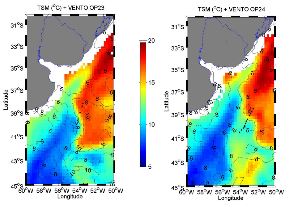
Figura 4.5 - Posições das radiossondas atmosféricas (pontos negros) a partir do NApOc Ary Rongel nas OP23 e OP24 (2004 e 2005), juntamente com a magnitude do vento obtida pelo escaterômetro a bordo do satélite QuikScat, sobrepostos ao mapa de TSM (cores) obtido pelo sensor AMSR-E do satélite Aqua.
