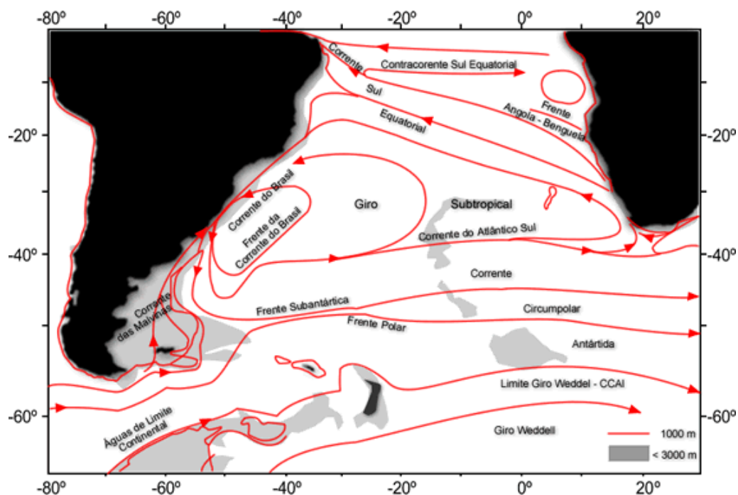
Figura 2.1 - Circulação Superficial média do Oceano Atlântico Sul.
