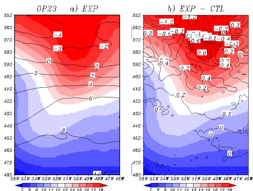
Figura 5.25 - TSM (escala sombreada) em ( ^{\circ}\text{C} ), o Vento Zonal (linhas de contorno) em ( \text{m/s} ). Para OP23 no período de 03/11/2004 às 12 UTC utilizando uma média de três dias. Painel a) Experimento EXP. Painel b) EXP - CTL.
