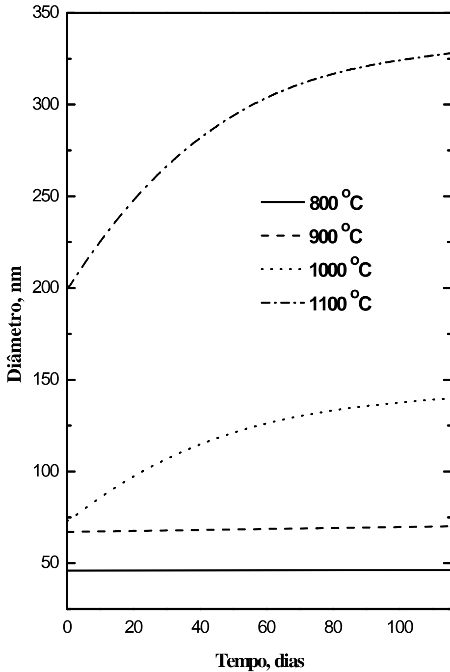
Figura 5.13 – Coalescimento das partículas de MnS a quatro temperaturas de trabalho
