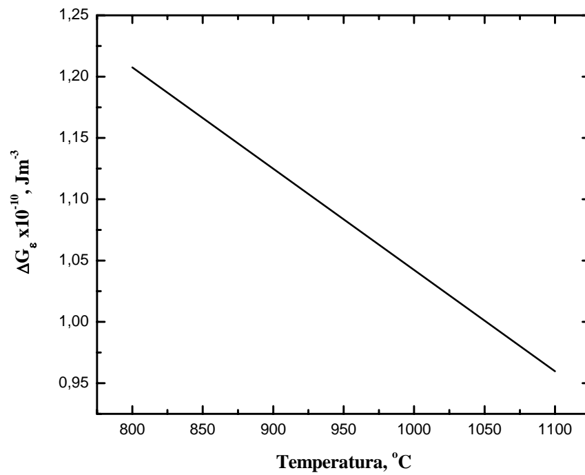
Figura 5.4a – Energia de deformação associada à nucleação coerente de MnS
