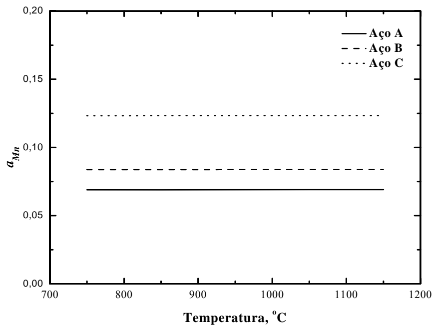
Figura 5.1a – Atividade de Mn na matriz original
