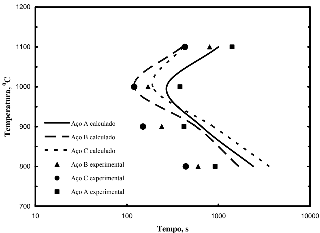
Figura 5.11 – Tempos para início de precipitação: curvas calculadas e pontos experimentais
