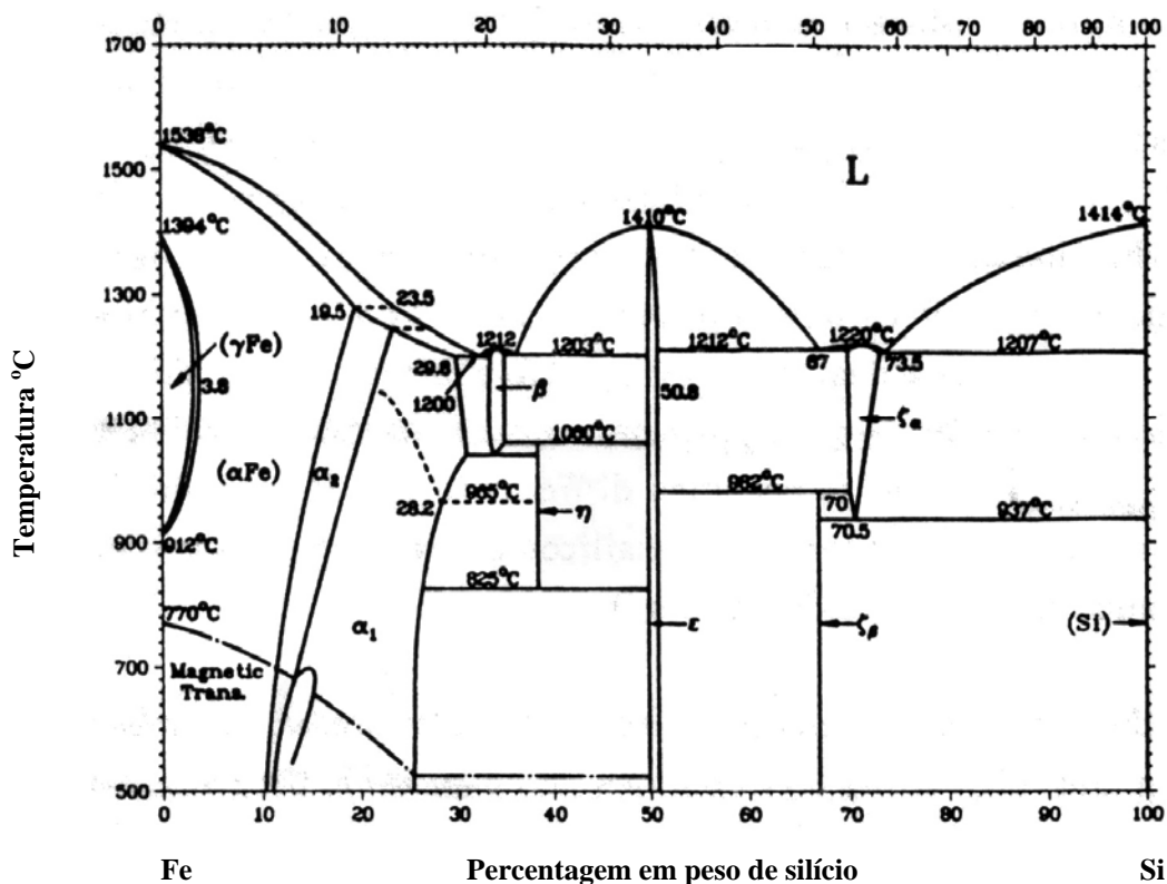
Figura 3.1 – Diagrama de fases Fe-Si contendo 0,03% de C (2)
