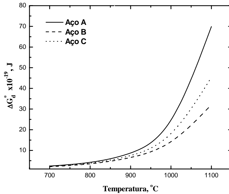
Figura 5.8a – Variação da energia livre crítica para precipitação semi-coerente em deslocações.
