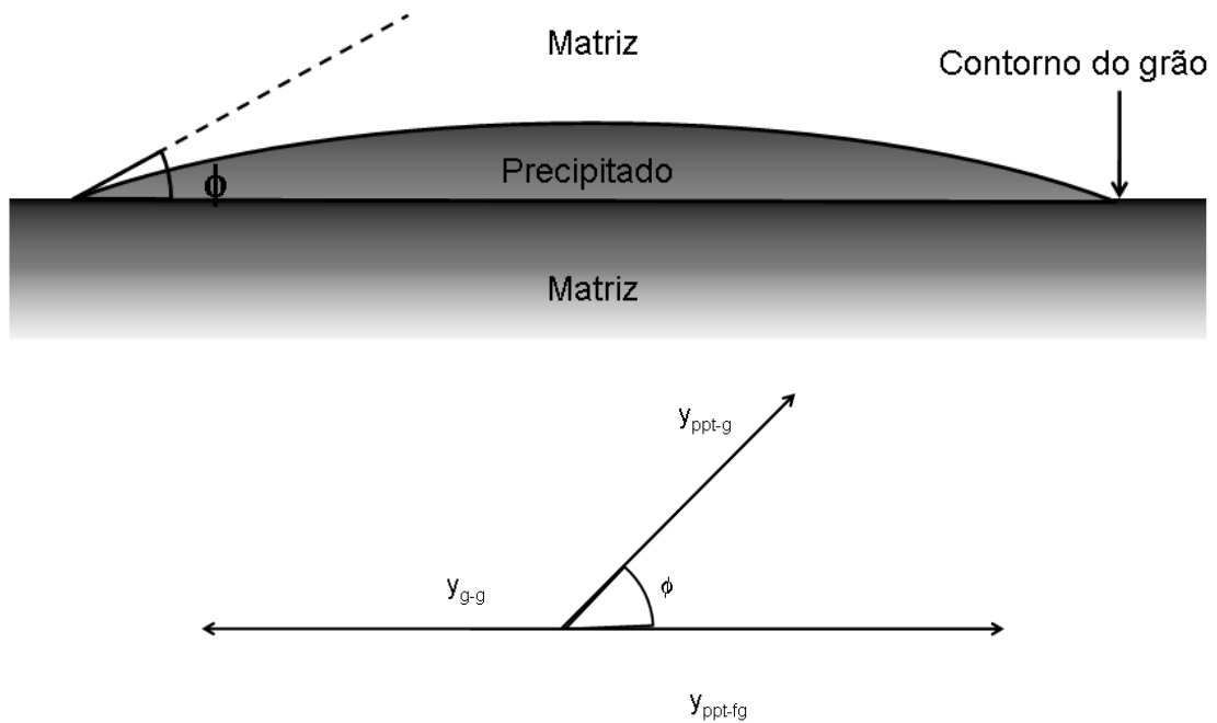
Figura 4.1 – Nucleação na fronteira de grão e representação das forças associadas (26)
