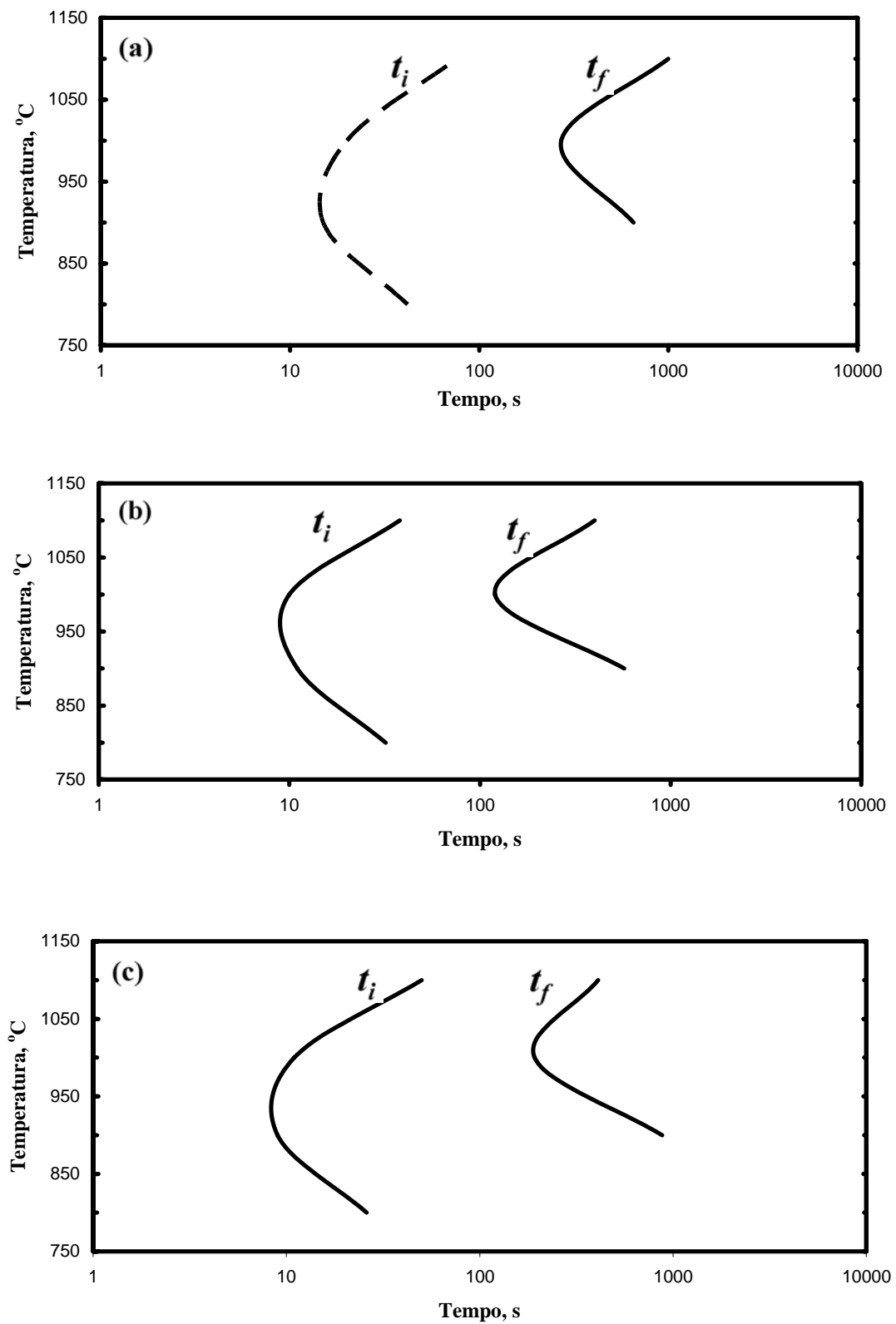
Figura 5.12 – Diagramas TTP para três aços Si: (a) aço A; (b) aço B e (c) aço C
