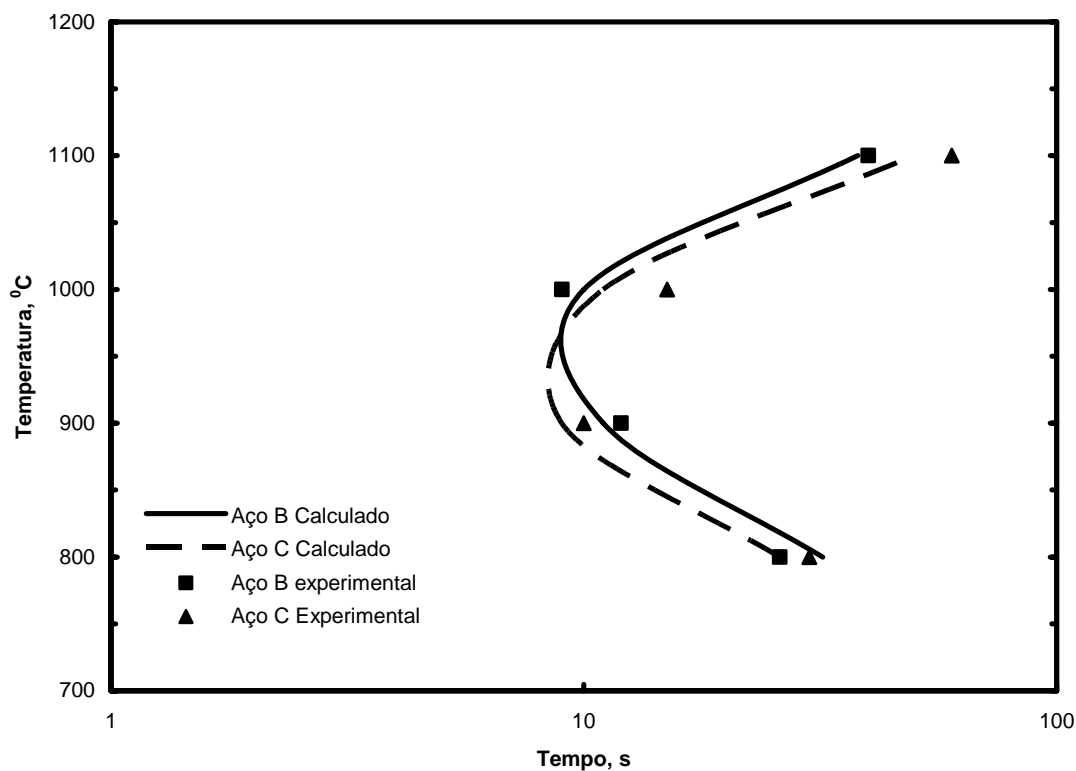
Figura 5.10 – Tempo para início de precipitação: curva calculada e pontos experimentais
