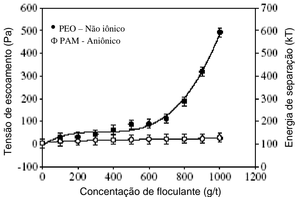
Figura 3.40: Tensão de escoamento e energia de separação de flocos (kT) em função da dosagem de flocoantes aniônico e não iônico. (Mpofu et al., 2004)
