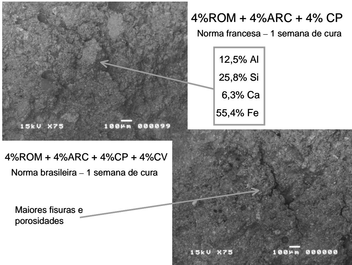
Figura 5.26 Imagens MEV obtidas via elétrons eletrospalhados; Superior: Vista geral da superfície de fratura de corpo de prova cimentado com os ligantes dos 2 metacaulins (MK) e cimento Portland (CP); Inferior: Vista geral de outra superfície de fratura que corresponde a um corpo de prova cimentado com os 4 ligantes estudados (16% do total).
