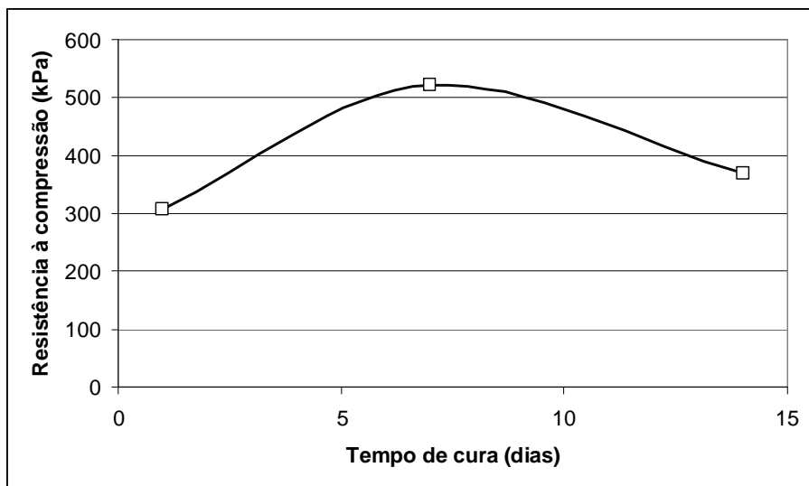
Figura 5.20: Resistências à compressão dos corpos de prova ensaiados de acordo a norma brasileira.
