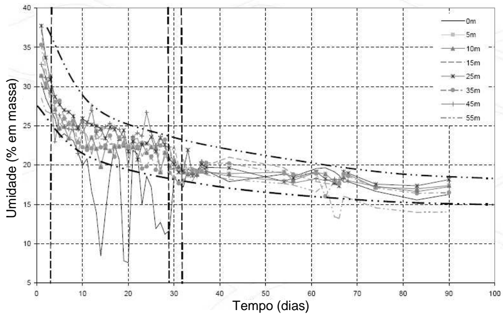
Figura 3.32: Perfil da umidade gravimétrica em função do tempo da secagem da pasta da usina Bulyanhulu. (Theron et al., 2005)
