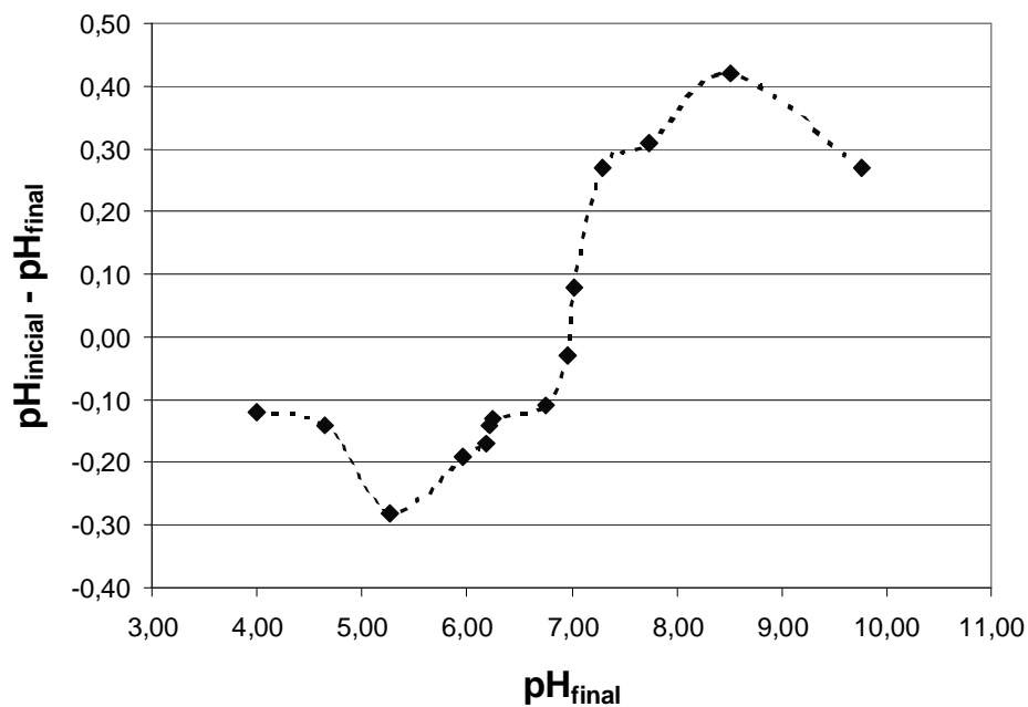
Figura 5.5: Resultado do teste de Mular e Roberts mostrando uma reversão de sinal de carga para um valor de pH de 6,98.
