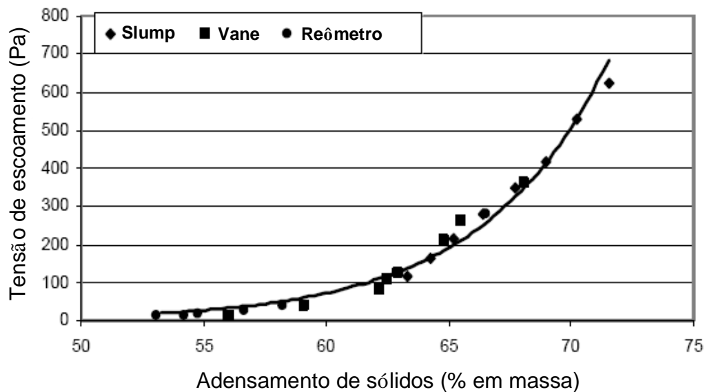
Figura 3.26: Comportamento da tensão de escoamento em função do adensamento da pasta. (Fourie, 2003)
