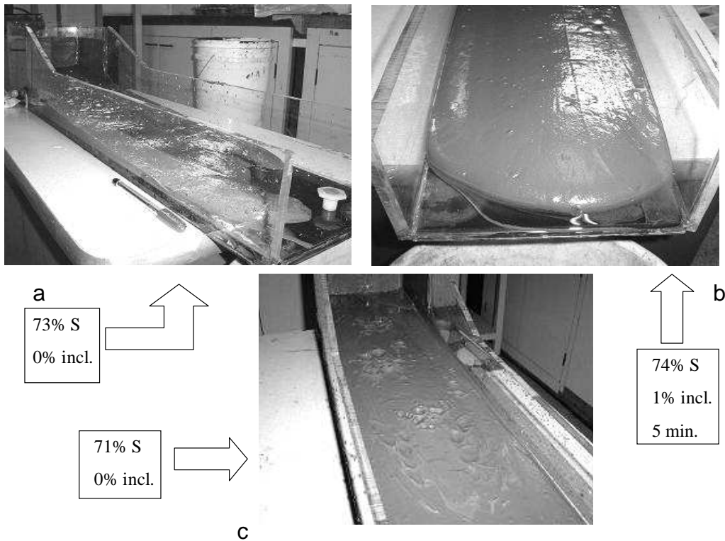
Figura 3.18: Pastas ensaiadas pelo teste de calha considerando diferentes adensamentos e inclinações de calha. (Araujo et al., 2004)
