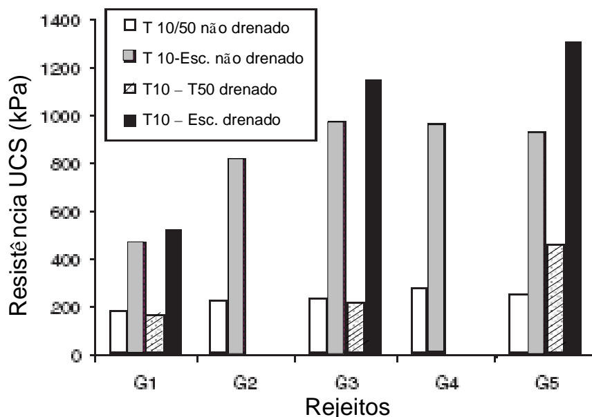
Figura 3.46: Efeito da distribuição de tamanho de partículas e da drenagem sobre a resistência mecânica de pastas cimentadas. (Benzaazoua et al., 2004)
