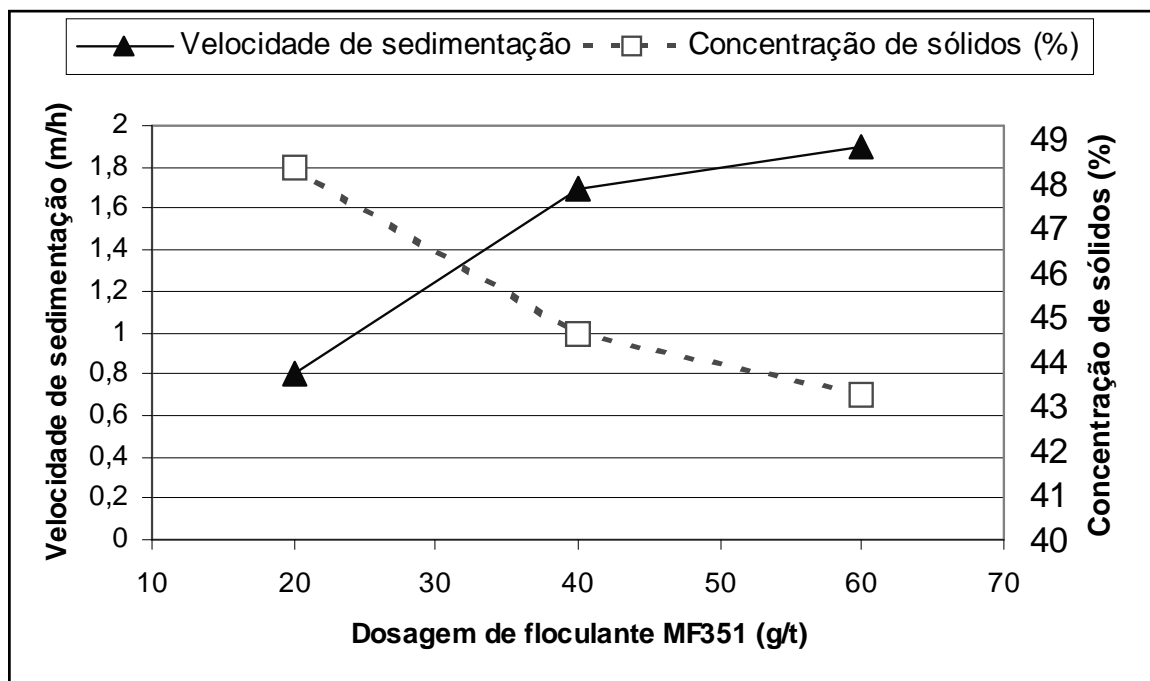
Figura 3.38: Efeito da dosagem de floculante sobre a velocidade de sedimentação e a concentração de sólidos na polpa. (Bedell et al., 2003)
