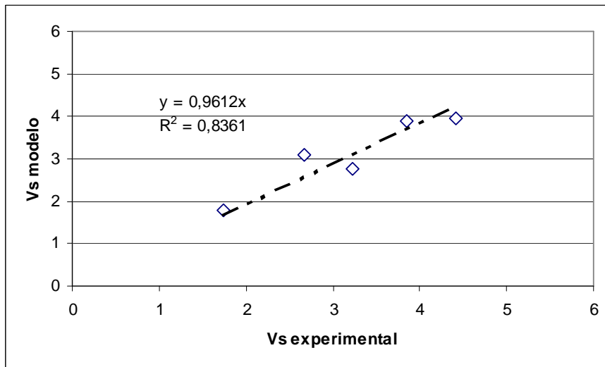
Figura 5.11: Gráfico comparativo dos valores da velocidade de sedimentação ( \times 10^4 cm/min) da pasta de 75% de sólidos obtidos experimentalmente e preditos pelo modelo.
