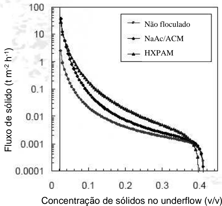
Figura 3.35: Efeito da floculação sobre o comportamento do fluxo de sólido em função da concentração de sólido na descarga do espessador. (Scales, 2003)
