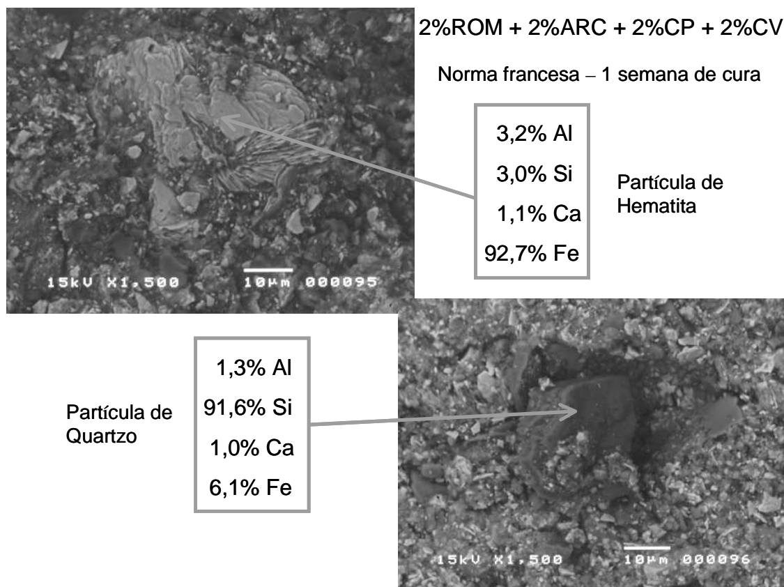
Figura 5.24: Imagens MEV obtidas via elétrons eletrospalhados; Superior: Partícula mais clara e brilhante de hematita detetada num corpo de prova cimentado com os ligantes dos 2 metacaulins (MK), cinzas volantes (CV) e cimento Portland (CP); Inferior: partícula mais escura que contém principalmente quartzo.
