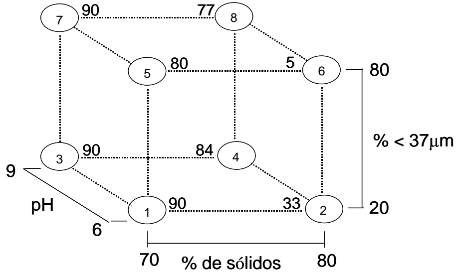
Figura 5.13: % de abatimento obtidas nas diferentes pastas estudadas.
