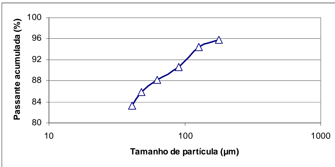
Figura 5.1: Curva granulométrica da amostra sólida obtida por peneiramento.
