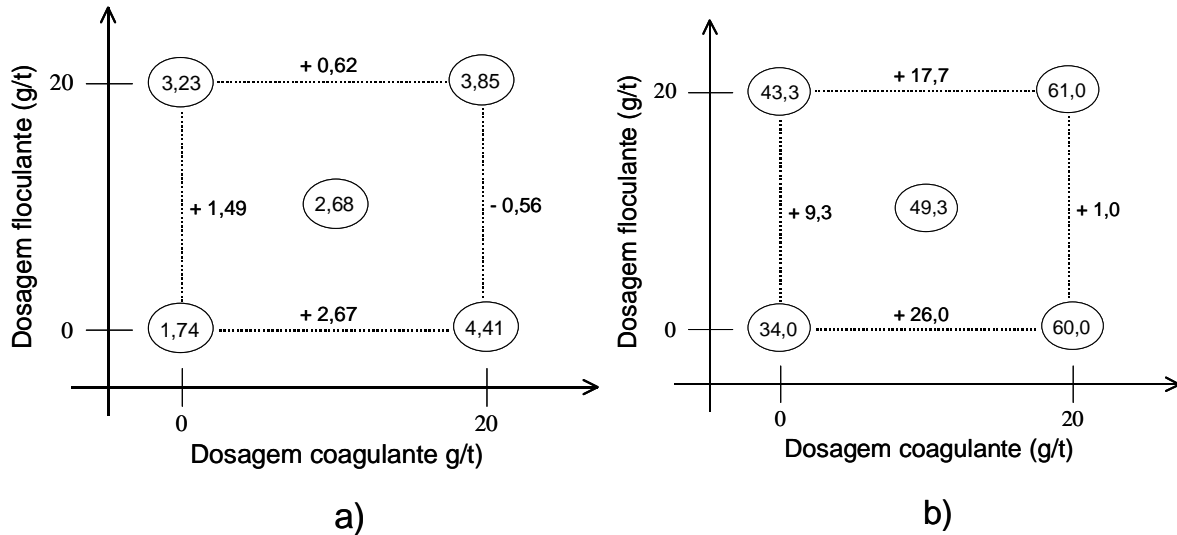
Figura 5.9: Gráficos de: a) velocidades de sedimentação ( \times 10^4 cm/min) e b) % de abatimento obtidas nas diferentes condições de agregação na pasta mineral de 75% de sólidos.
