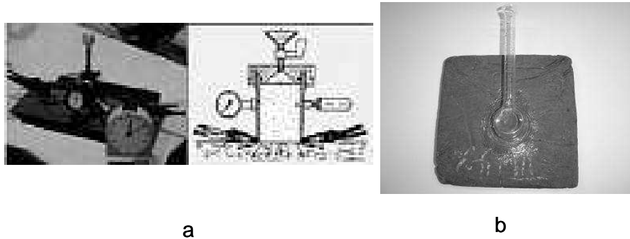
Figura 4.9: a) Permeabilímetro de Germann; b) Permeabilímetro de Karsten. (Hernández, 2005)
