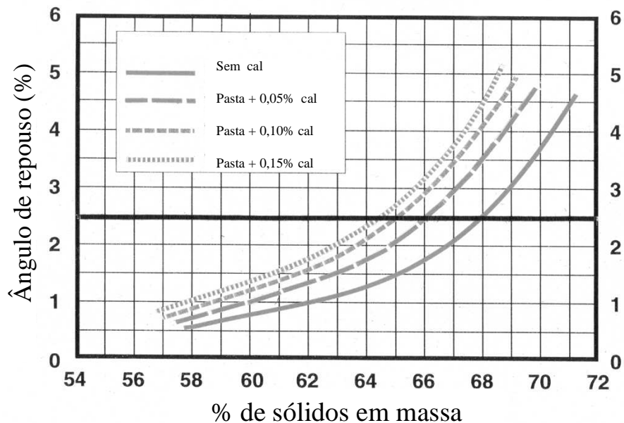
Figura 3.42: Efeito da adição de cal sobre o comportamento do ângulo de repouso em função do adensamento de sólido em massa. (Robinsky, 2002)
