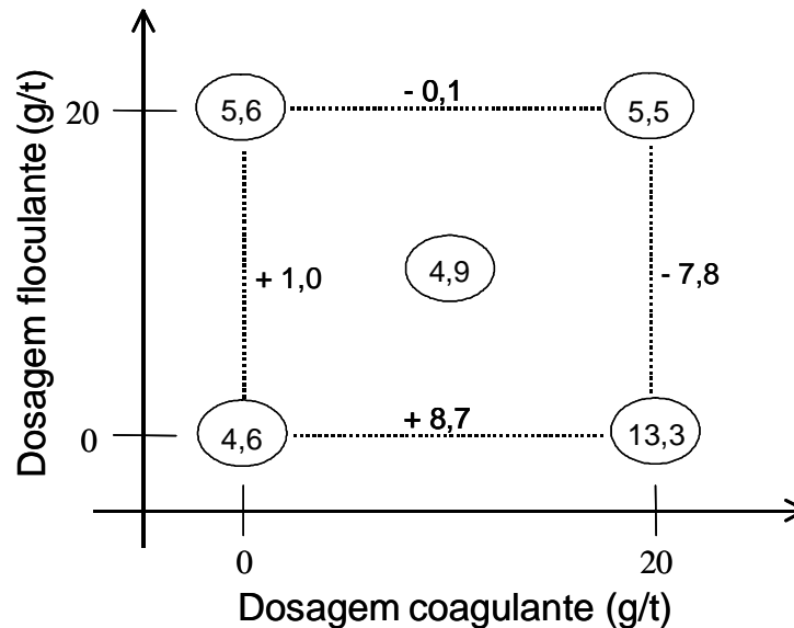
Figura 5.8: Gráfico das velocidades de sedimentação ( \times 10^3 cm/min) obtidas nas diferentes condições de adição de agregantes na polpa de 70% de sólidos.
