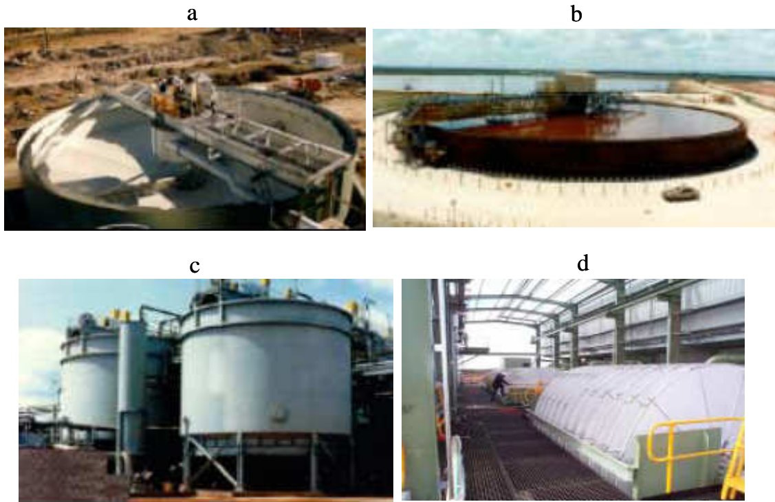
Figura 3.5: Equipamentos de desagamento utilizados na produção industrial de polpas e pastas minerais: a) espessador de alta velocidade; b) espessador de alta densidade; c) espessadores de pasta (cone profundo); d) filtros a vácuo. (GL&V, 2003)
