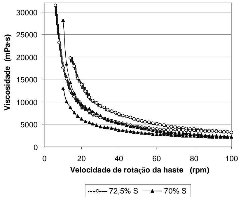
Figura 3.23: Comportamento da viscosidade de pastas adensadas com 70 e 72,5% de sólidos. (Araujo et al., 2004)
