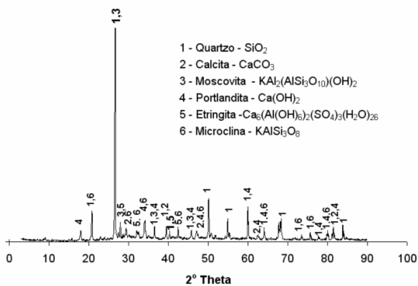
Figura 5. 26 – Espectro de DRX do concreto CONC5% na idade de 28 dias.
