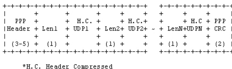
Figura 2.24: Exemplo de multiplexação em um frame PPP (PAZHYANNUR; ALI, 1999).
