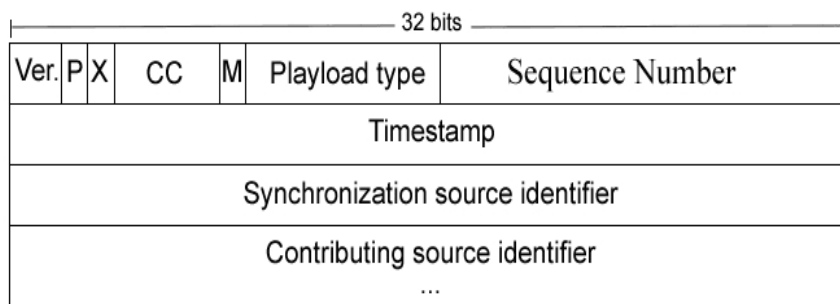
Figura 2.6: Formato do Pacote RTP (SCHULZRINNE et al., 2003).
