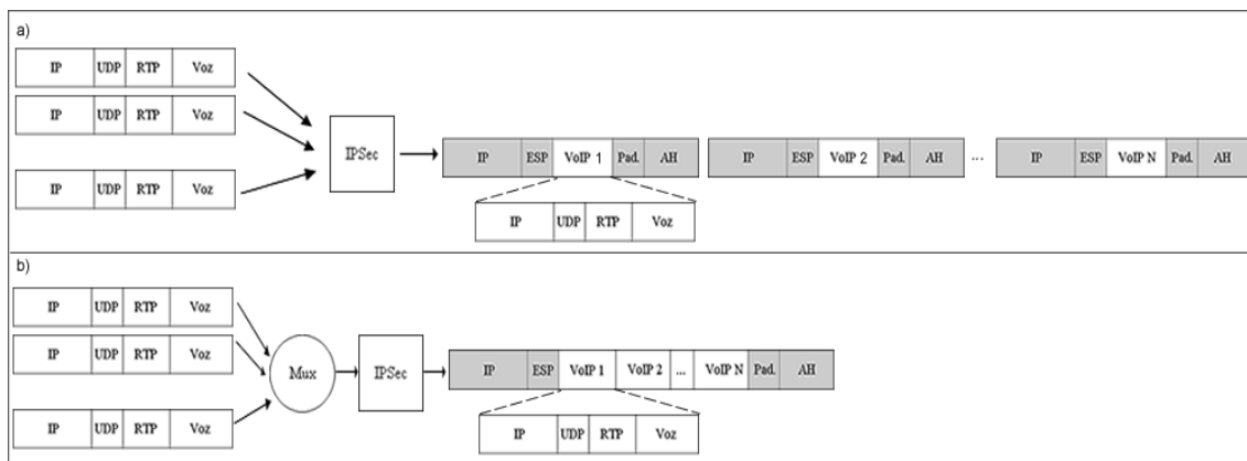
Figura 2.23: a) Fluxo convencional de ligações VoIP sobre IPsec. b) Fluxo de ligações VoIP multiplexados sobre IPsec.
