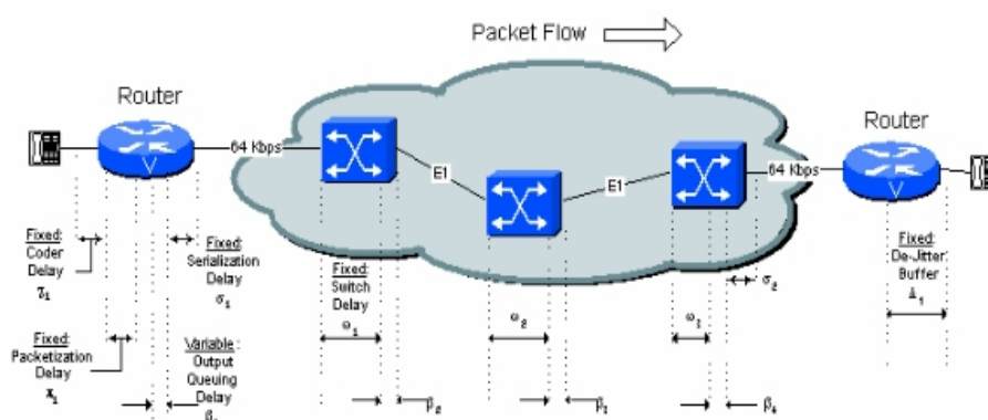
Figura 2.7: Atrasos total de fala-e-escuta (CISCO, 2007a).
