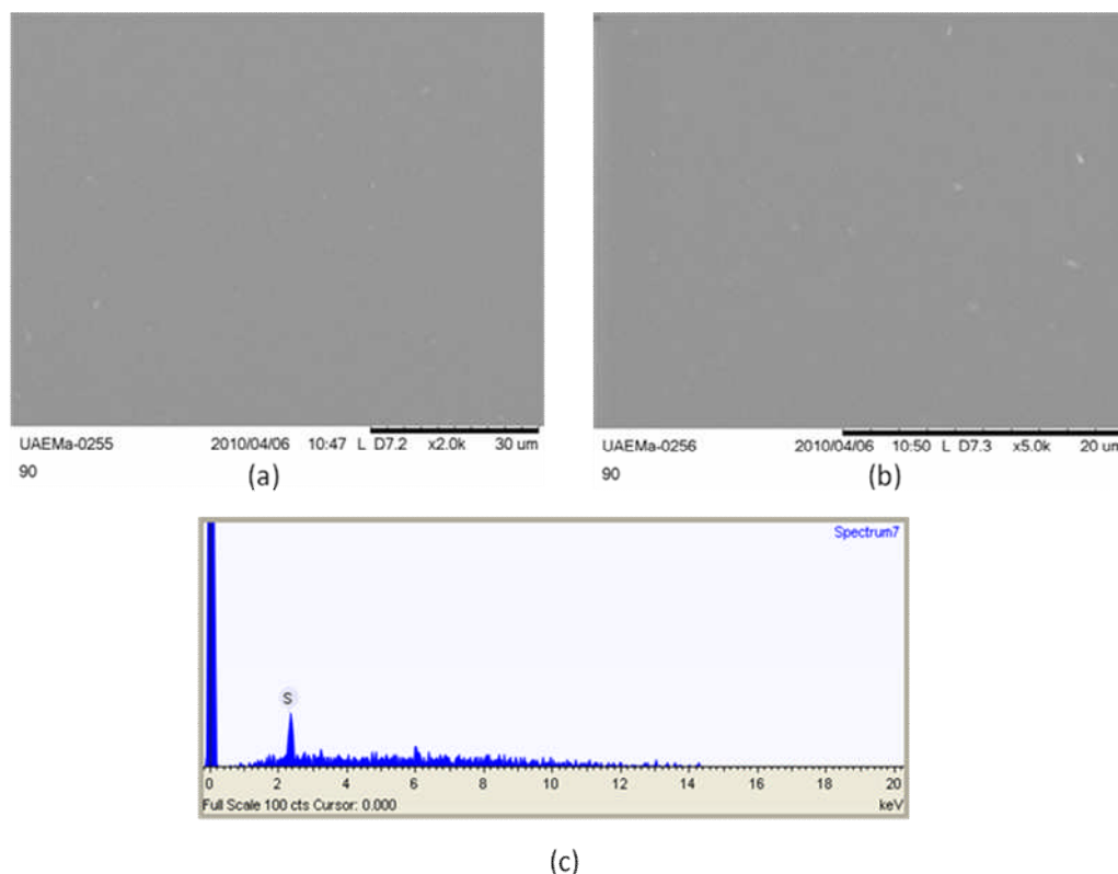
Figura 23. MEV e EDX dos filmes reticulados de quitosana com 90 minutos de reação:
