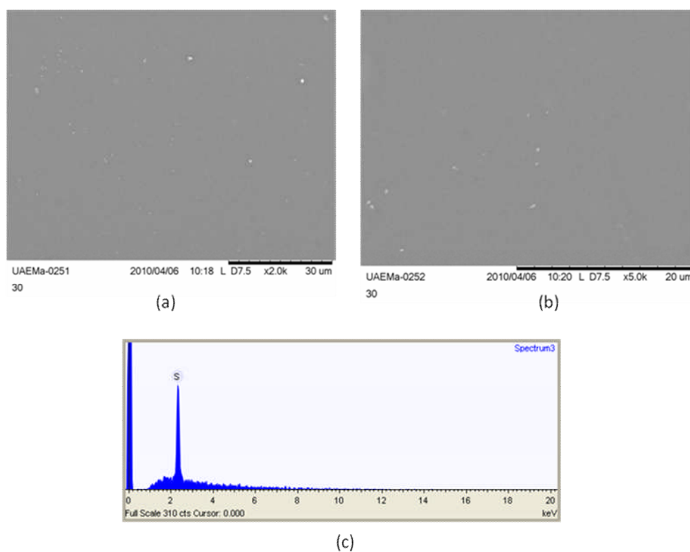
Figura 21. MEV e EDX dos filmes reticulados de quitosana com 30 minutos de reação: (a) 2000 X (b) 5000 X e (c) 2000 X.
