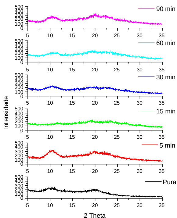
Figura 16. Difratograma de filmes de quitosana puro e reticulados.
