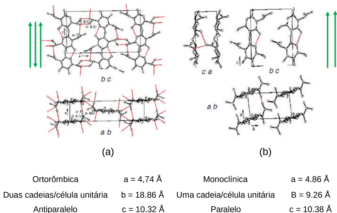
Figura 5. Estrutura cristalina para (a) \alpha -quitina e (b) \beta -quitina. Fonte: TOKURA & TAMURA, 2007
