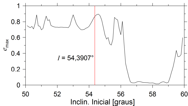
Figura 7.1. GPS Bloco IIA-10 (PRN 32). Condições iniciais: a = 27.059,74 km, e = 0,0141577 , I = 55,4704^\circ , \Omega = 295,4267^\circ , \omega = 285,2469^\circ .
