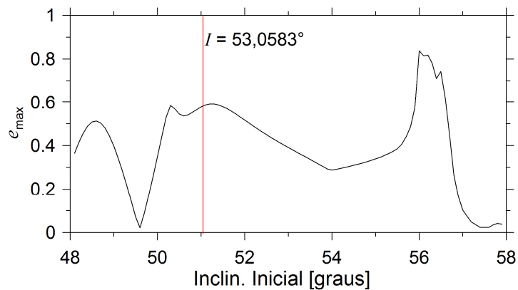
Figura 7.10. GPS Bloco IIA-25 (PRN 03). Condições iniciais: a = 27.059,74 km, e = 0,0107105 , I = 53,0583^\circ , \Omega = 164,4296^\circ , \omega = 47,0183^\circ .
