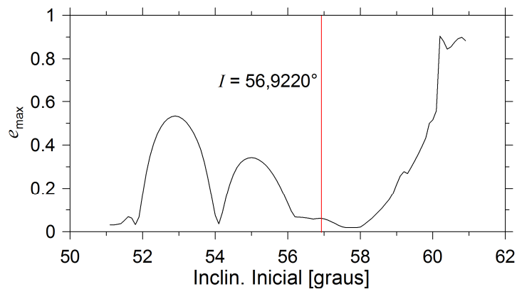
Figura 7.4. GPS Bloco IIA-14 (PRN 26). Condições iniciais: a = 27.059,74 km, e = 0,0189872 , I = 56,9220^\circ , \Omega = 353,2625^\circ , \omega = 54,0809^\circ .
