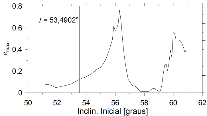
Figura 7.9. GPS Bloco IIA-24 (PRN 06). Condições iniciais: a = 27.059,74 km, e = 0,0061057 , I = 53,4902^\circ , \Omega = 168,1686^\circ , \omega = 267,4498^\circ .
