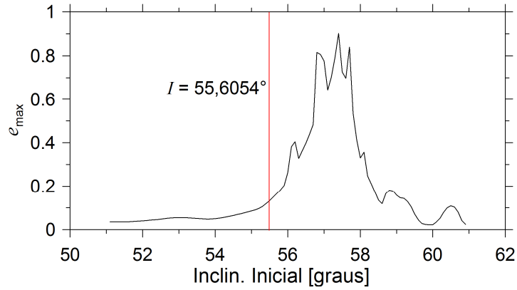
Figura 7.5. GPS Bloco IIA-15 (PRN 27). Condições iniciais: a = 27.059,74 km, e = 0,0214233 , I = 55,6054^\circ , \Omega = 47,1235^\circ , \omega = 263,1470^\circ .
