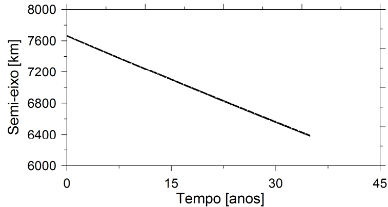
Figura 4.4. Variação do semi-eixo maior do satélite sob o efeito da força de arrasto com densidade atmosférica constante. Condições iniciais: C_d = 1,2 , a_0 = 7.653,7632 km, e = 0,00125 (Landsat 7), I = 98,67^\circ (para esta inclinação a = 7.193,968 km é o semi-eixo ressonante), \omega = 90^\circ e \Omega = 40^\circ .
