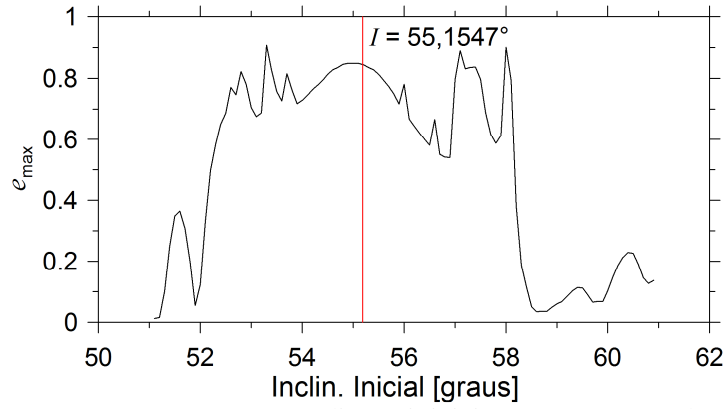
Figura 7.11. GPS Bloco IIA-26 (PRN 10). Condições iniciais: a = 27.059,74 km, e = 0,0078202 , I = 55,1547^\circ , \Omega = 292,0277^\circ , \omega = 30,8981^\circ .
