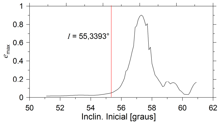
Figura 7.3. GPS Bloco IIA-12 (PRN 25). Condições iniciais: a = 27.059,74 km, e = 0,0077676 , I = 55,3393^\circ , \Omega = 45,1394^\circ , \omega = 288,2011^\circ .
