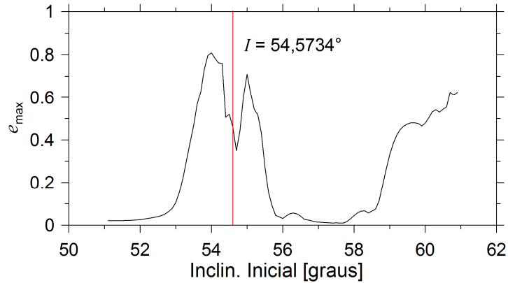
Figura 7.2. GPS Bloco IIA-11 (PRN 24). Condições iniciais: a = 27.059,74 km, e = 0,0077676 , I = 54,5734^\circ , \Omega = 233,5216^\circ , \omega = 317,5531^\circ .
