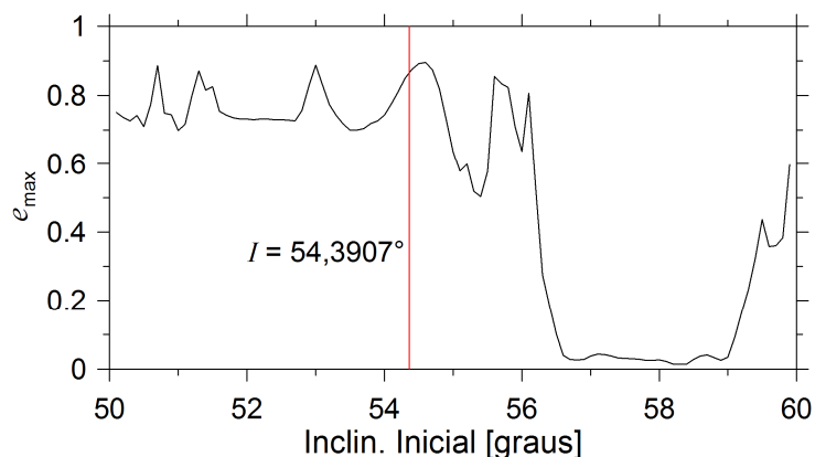
Figura 3.17. Excentricidade máxima atingida pelo satélite GPS Bloco IIA-27 (PRN 30) para uma grade de inclinações iniciais. A inclinação nominal do satélite está marcada pela linha vertical vermelha. Condições iniciais: a = 27.059,74 km, e = 0.0106654 , I = 54.3907 , \Omega = 108.2529^\circ , \omega = 79.3795^\circ (CelesTrak, 12/08/08); I_L = 18.28^\circ .
