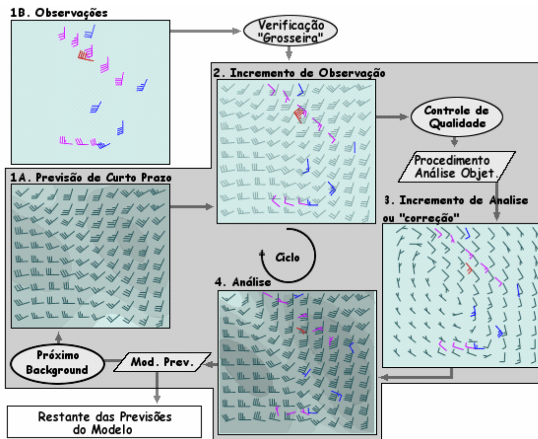
Figura B.1: Diagrama esquemático do Ciclo de Assimilação de Dados.
