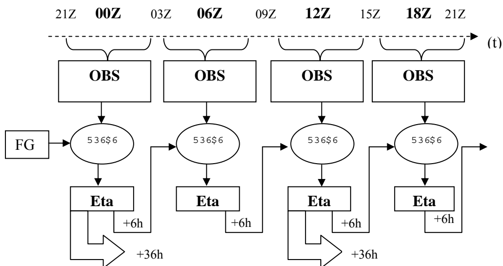
Figura 3.1 - Representação esquemática simplificada do ciclo de assimilação de dados.
