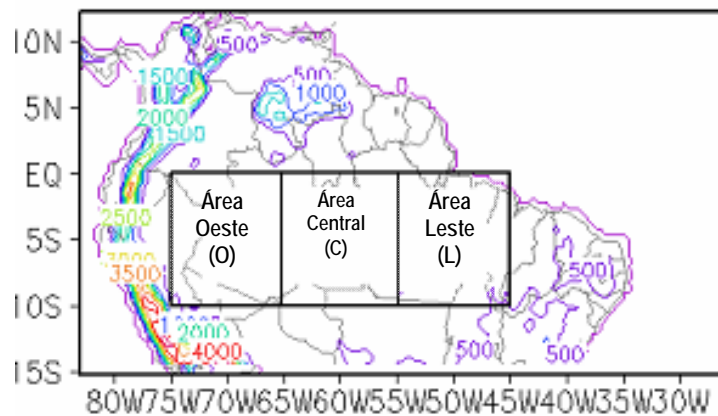
Figura 3.2 - Representação esquemática das áreas geográficas definidas para o estudo.
