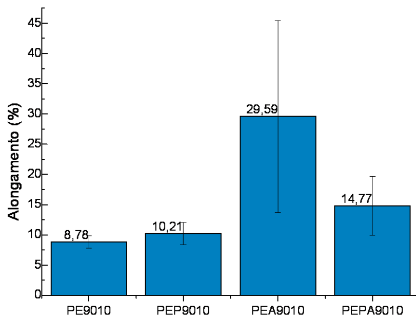
Figura 5.13. Alongamento dos híbridos e das misturas na proporção 90:10
