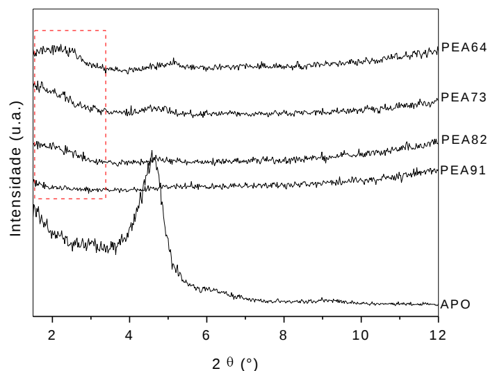
Figura 5.6. Difratomogramas dos híbridos PP/EPDM/APO com razões de PP para EPDM correspondentes a 90:10; 80:20; 70:30 e 60:40 e quantidade de APO de 1 pcr (PEA91, PEA82, PEA73 e PEA64, respectivamente).
