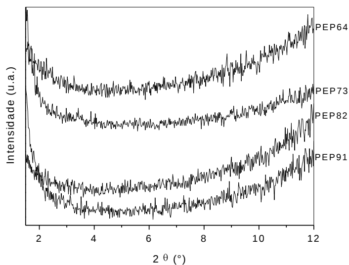
Figura 5.5. Difratogramas das misturas PP/EPDM/PP-g-MA com razões de PP para EPDM e PP-g-MA correspondentes a 90:10; 80:20; 70:30 e 60:40 (PEP91, PEP82, PEP73 e PEP64, respectivamente).
