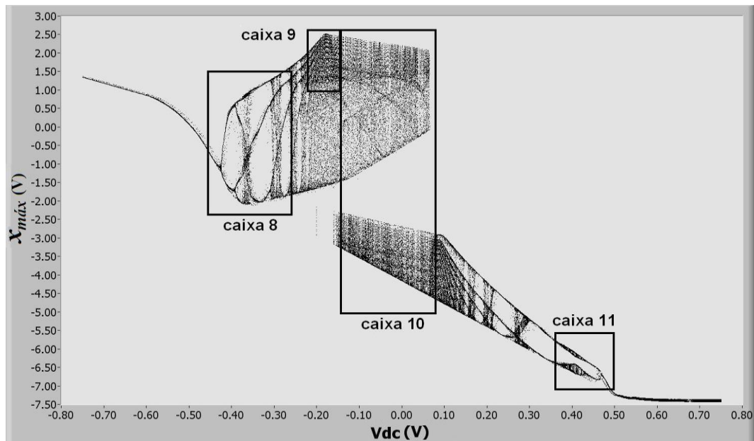
Figura 4.17: Diagrama de bifurcação R = 1680,00 \Omega , V_{DC} entre -0,7500 \text{ V} e +0,7500 \text{ V} .
