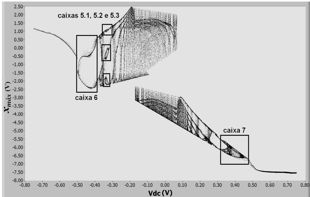
Figura 4.16: Diagrama de bifurcação R = 1668,00 \Omega , V_{DC} entre -0,7500 \text{ V} e +0,7500 \text{ V} .
