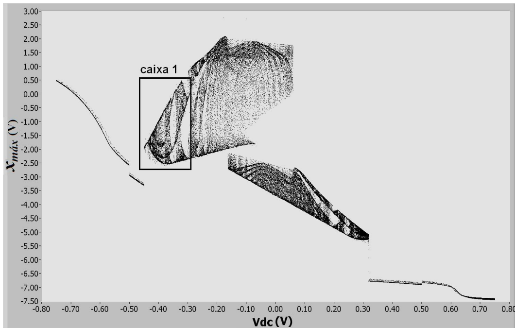
Figura 4.14: Diagrama de bifurcação R = 1600,00 \Omega , V_{DC} entre -0,7500 V e +0,7500 V.
