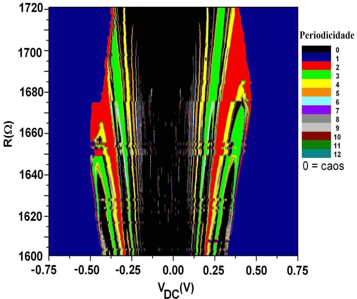
Figura 4.24: Espaço de Parâmetros da Periodicidade para R entre 160,00 \Omega e 1720,00 \Omega e V_{DC} entre -0,7500 V e +0,7500 V. Escala de 13 cores, uma cor para cada valor da periodicidade P da série temporal, sendo que para as séries caóticas ou de periodicidade acima de 12, foi definida a mesma cor, preta.
