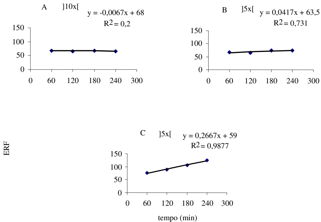
Figura 6.8. Atividade de cisteína-proteases (Catepsina L) da saliva de Dichelops melacanthus (A); Euschistus heros (B); e Nezara viridula (C). Insetos em jejum, diluição da saliva em colchetes abertos. ERF = Emissão Relativa de Fluorescência.
