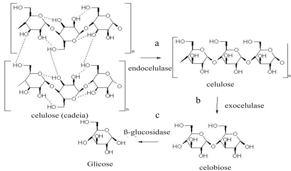
Figura 6.1. Mecanismo da digestão da celulose. Quebra das ligações não-covalentes presentes na estrutura cristalina da celulose pela endocelulase (a); hidrólise da cadeia polissacarídica em dissacarídeos pela exocelulase (b); hidrólise dos dissacarídeos em glicose pela \beta -glucosidase (c) (baseado em Nation 2002).
