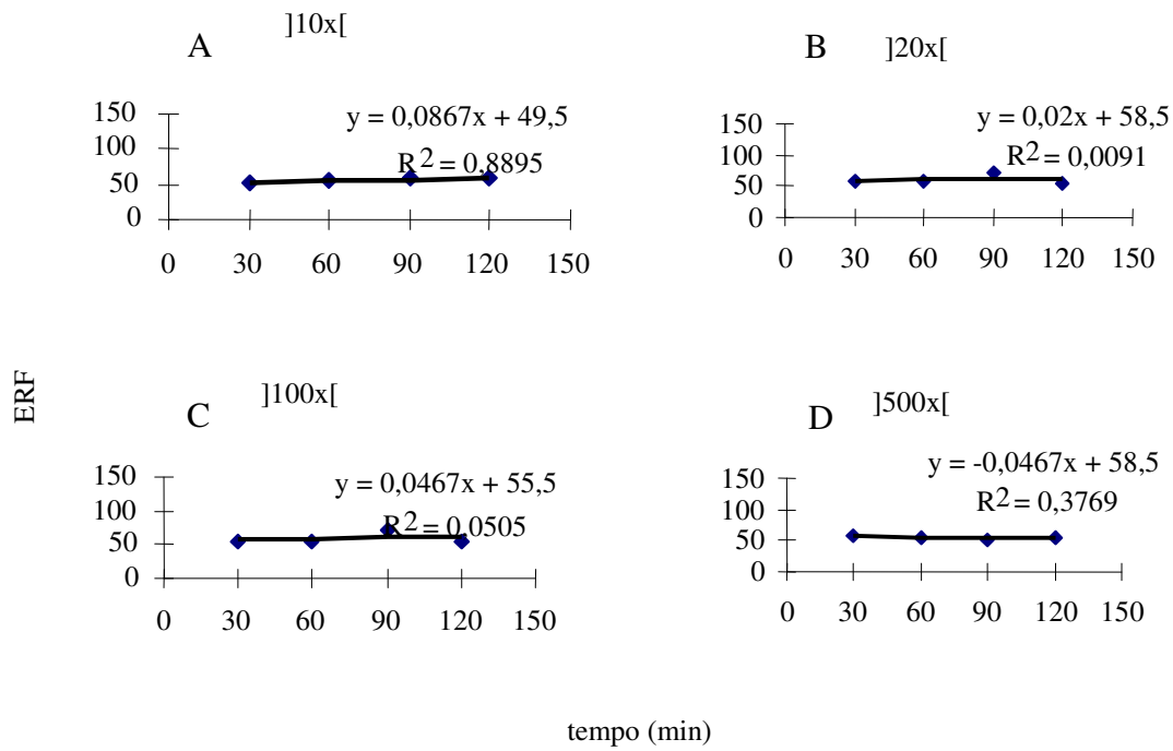
Figura 6.7. Atividade de cisteína-proteases (Cathepsina L) da saliva de Nezara viridula em diferentes diluições. A = 10x; B = 20x; C = 100 x; D = 500x. Insetos alimentados. ERF = Emissão Relativa de Fluorescência.
