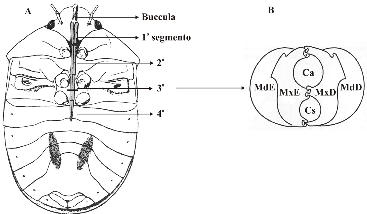
Figura 3.2. Diagrama geral da estrutura do aparelho bucal de um pentatomídeo (A), e secção transversal dos estiletos no 3º segmento do lábio (B). Ca = canal de alimento; Cs = canal de saliva; MdE = mandíbula esquerda; MdD = mandíbula direita; MxE = maxila esquerda; MxD
