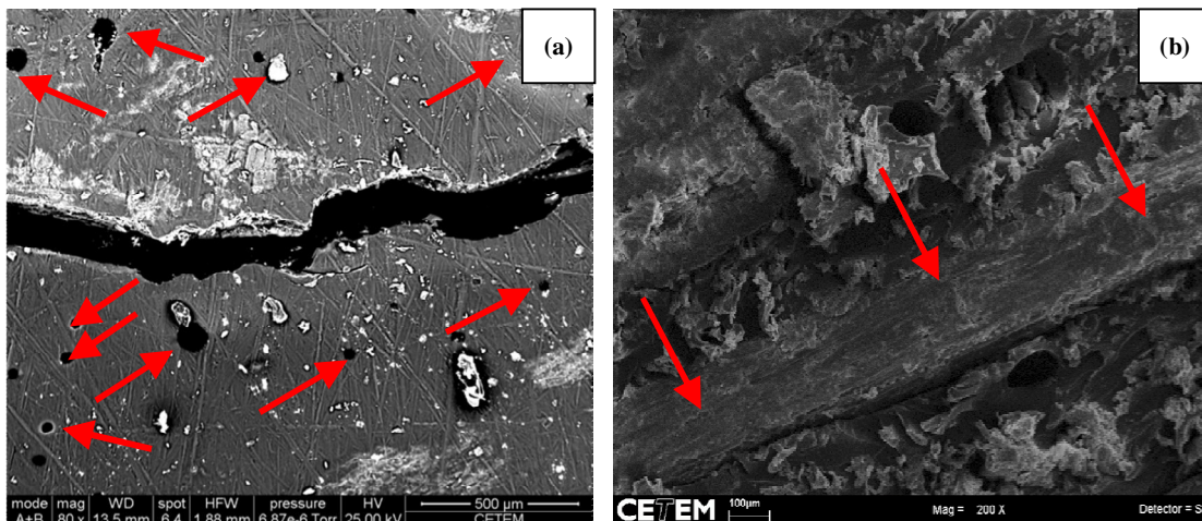
Figura 4.14– Imagem de MEV de: (a) trincamento da matriz e (b) região onde ocorreu o desacoplamento
