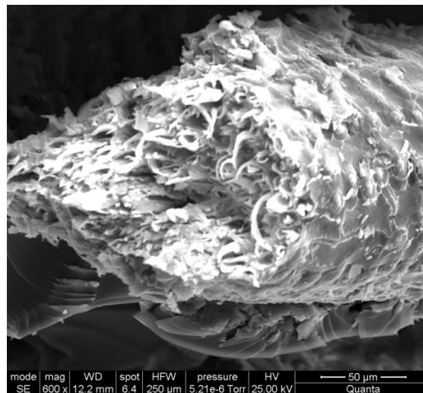
Figura 4.13 – Região da fratura da fibra de coco
