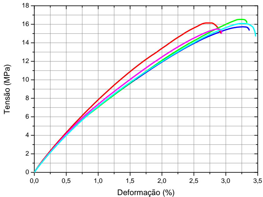
Figura 4.3 – Ensaio de Tração versus Deformação da Resina Epóxi reforçada com 20% de fibra de coco
