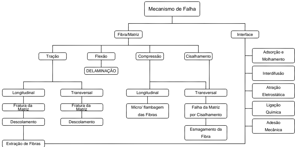
2.8 – Figura Fluxograma da relação entre os mecanismos de falhas (DA SILVA, J. L. G., 1996).
