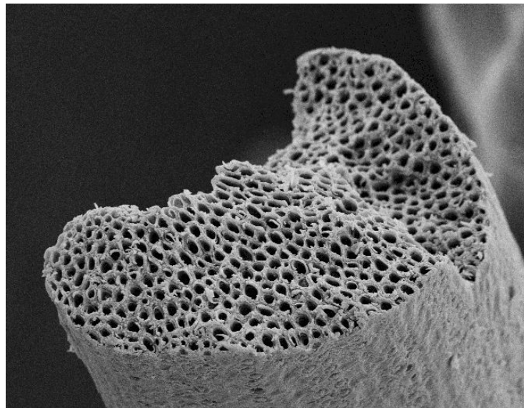
Figura 2.6 – Imagem obtida por MEV de um corte transversal da fibra do coco.
