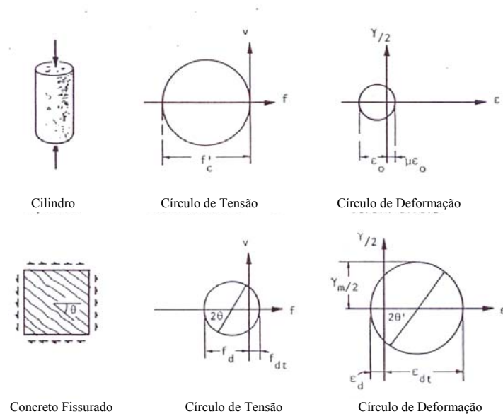
Figura 13: comparação de condições de tensões e deformações para um cilindro de teste e para um painel de concreto fissurado (VECCHIO, 1981, p. 33)
