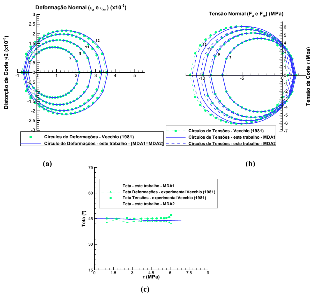
Figura 55: curvas do painel PV22: (a) Círculos de Mohr de Deformações; (b) Círculos de Mohr de Tensões; (c) variação do ângulo das tensões e deformações
