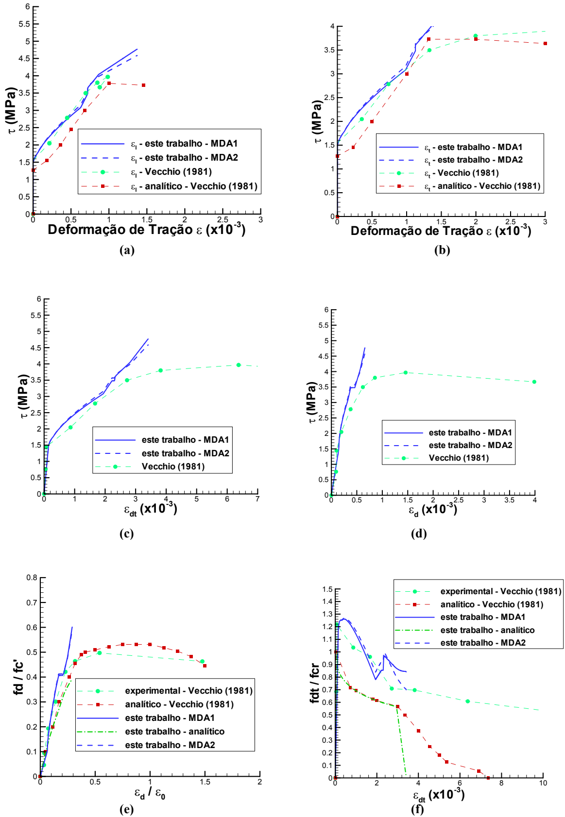
Figura 69: curvas do painel PV10 de (a) \epsilon_t \times \tau ; (b) \epsilon_t \times \tau (c) \epsilon_{dt} \times \tau ; (d) \epsilon_d \times \tau ; (e) deformações x tensões de compressão; (f) deformações x tensões de tração
