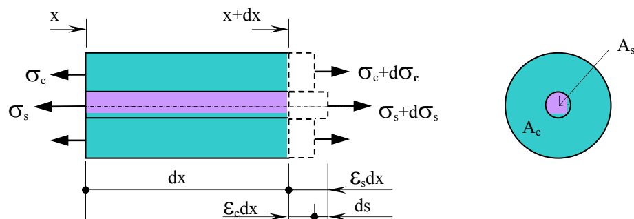
Figura 27: tensões e deformações na barra de aço e na camada de concreto adjacente
