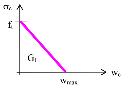
Figura 15: amolecimento linear
