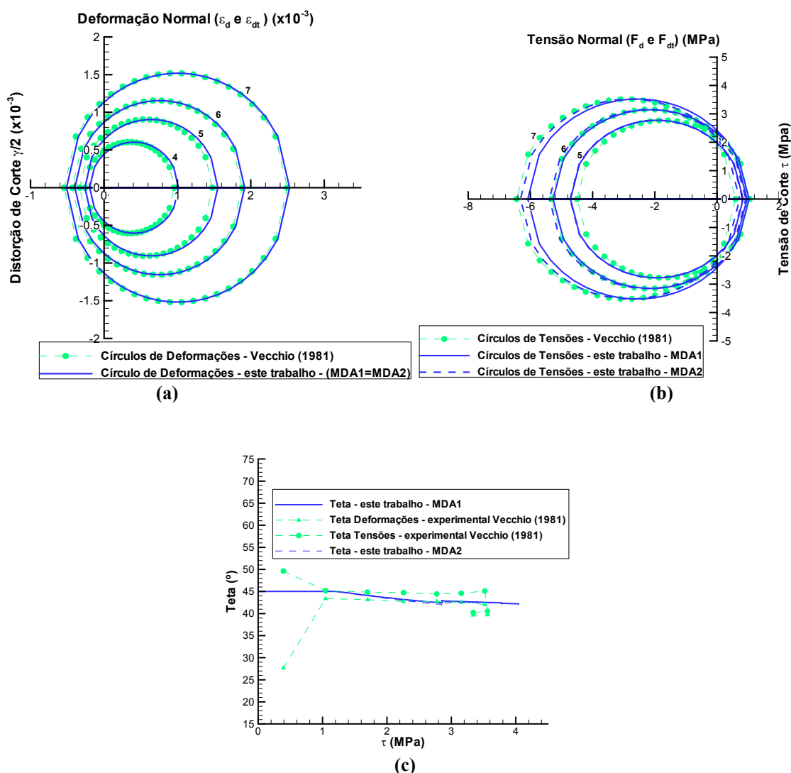
Figura 61: curvas do painel PV11: (a) Círculos de Mohr de Deformações; (b) Círculos de Mohr de Tensões; (c) variação do ângulo das tensões e deformações
