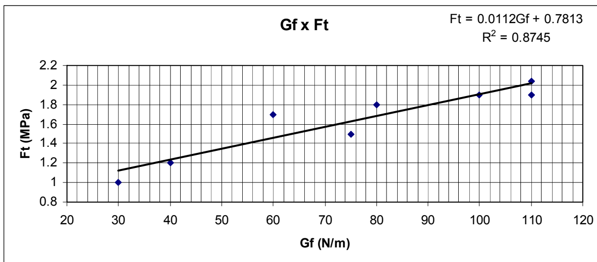
Figura 77: relação entre a resistência à tração do concreto e a energia de fratura
