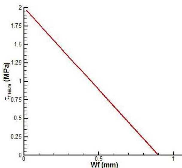
Figura 45: curva de amolecimento do painel de concreto simples
