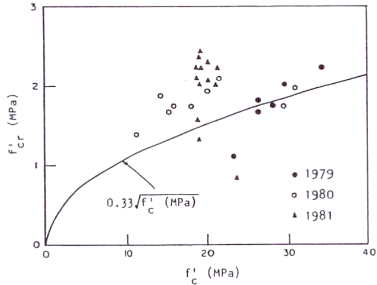
Figura 7: tensões de fissuração x resistência do cilindro (VECCHIO, 1981, p. 91)
