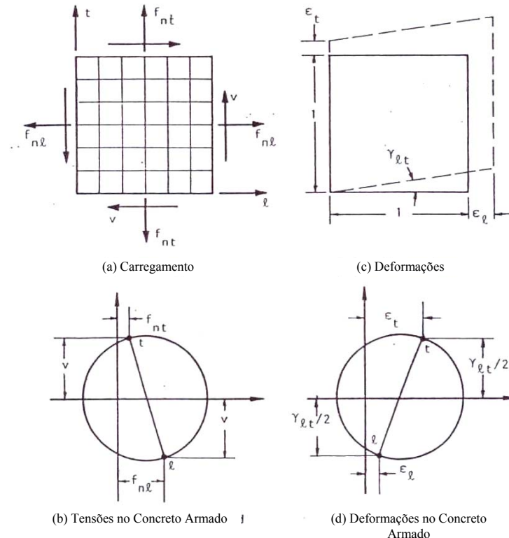
Figura 9: condições de tensão e deformação para o painel (VECCHIO, 1981, p. 19)
