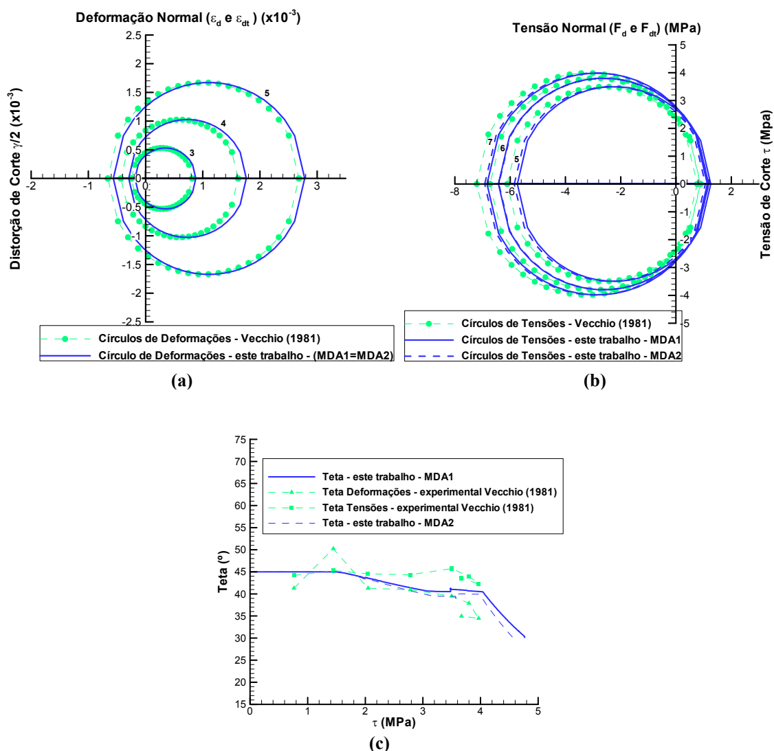
Figura 70: curvas do painel PV10: (a) Círculos de Mohr de Deformações; (b) Círculos de Mohr de Tensões; (c) variação do ângulo das tensões e deformações
