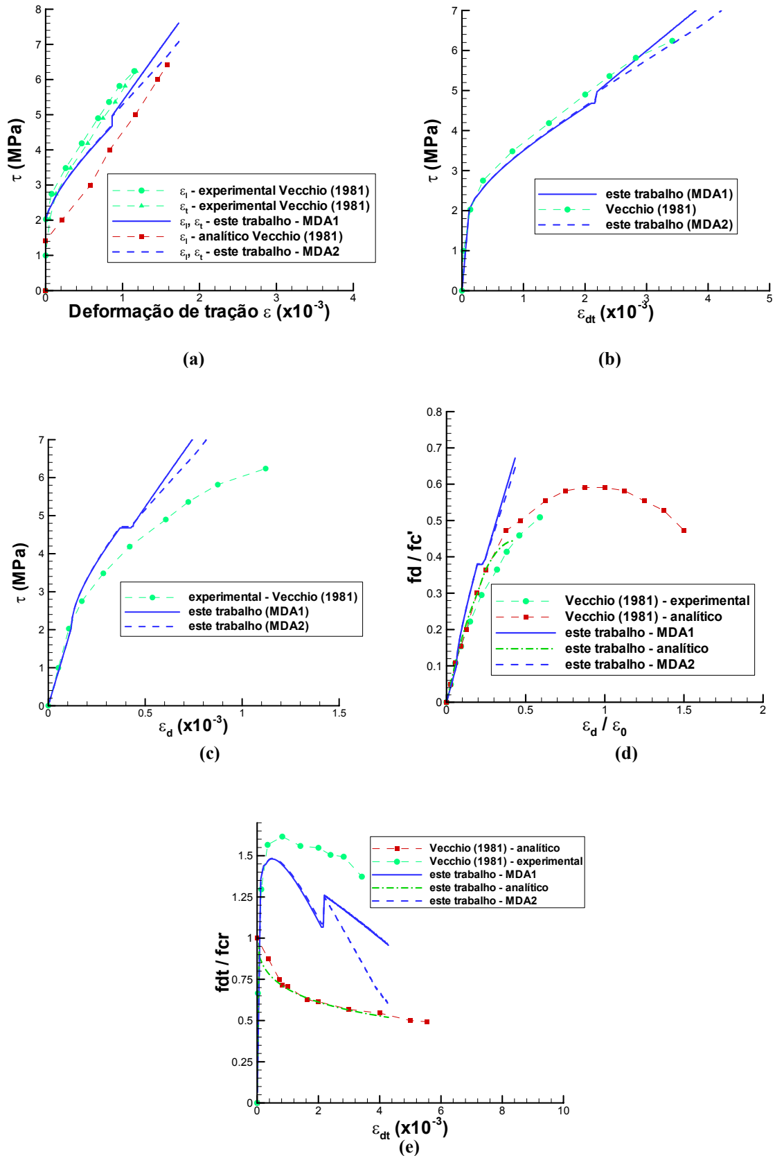
Figura 50: curvas do painel PV27 de (a) \varepsilon_l = \varepsilon_t \times \tau ; (b) \varepsilon_{dt} \times \tau ; (c) \varepsilon_d \times \tau ; (d) deformações x tensões de compressão; (e) deformações x tensões de tração
