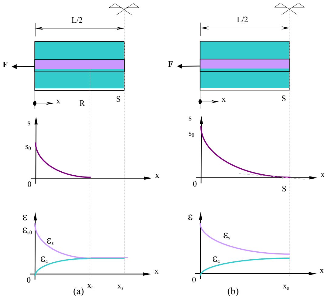
Figura 29: distribuição do escorregamento e das deformações no concreto e no aço:
