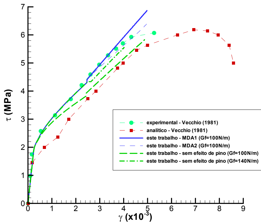
Figura 75: influência do efeito de pino na curva tensão tangencial x distorção para o painel PV22
