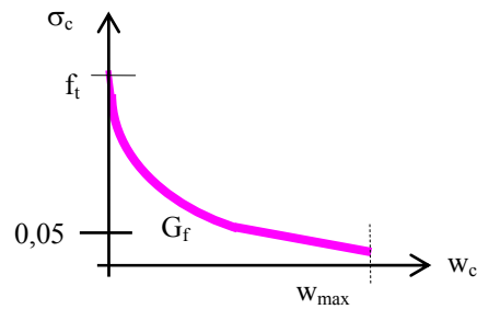
Figura 16: amolecimento exponencial
