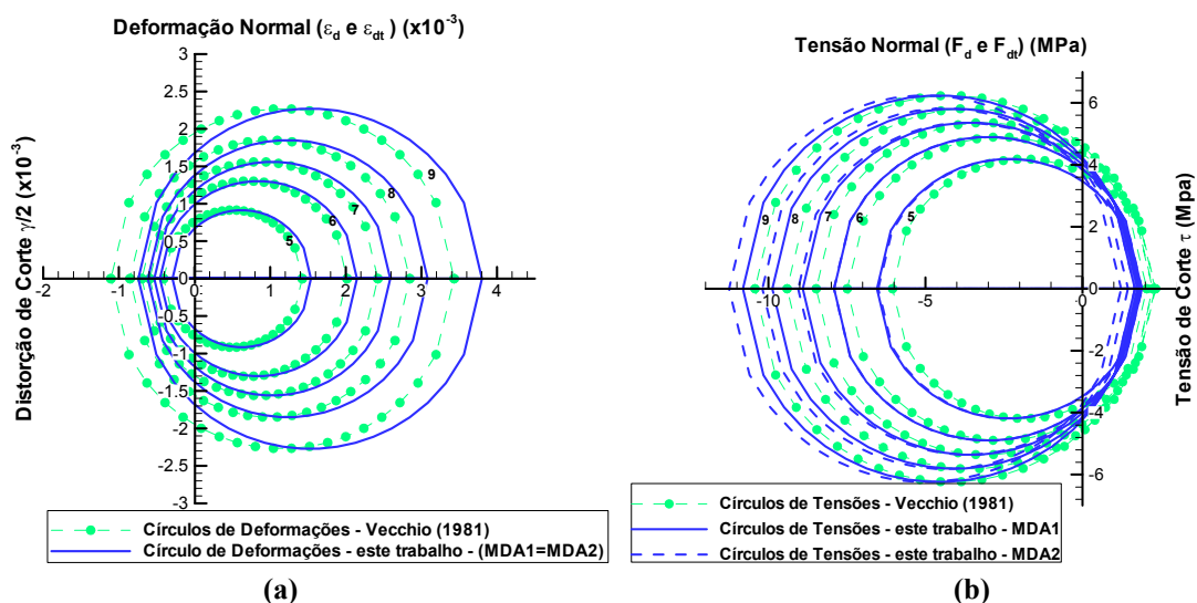
Figura 51: curvas do painel PV27: (a) Círculos de Mohr de Deformações; (b) Círculos de Mohr de Tensões
