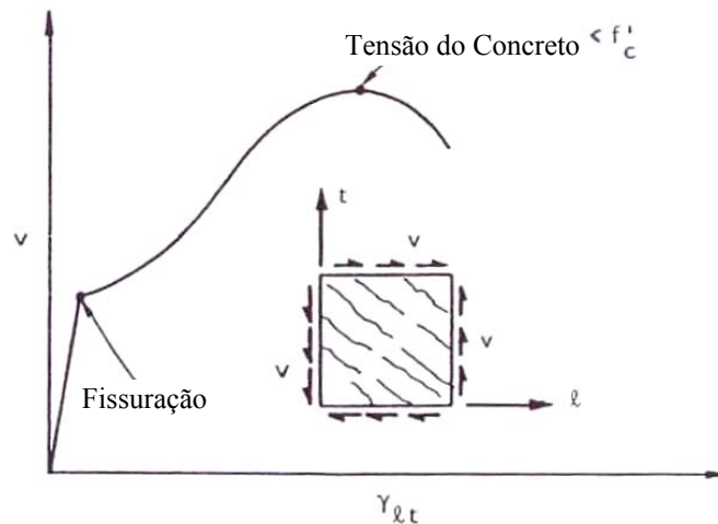
Figura 8: painel carregado em corte puro (VECCHIO, 1981, p. 5)
