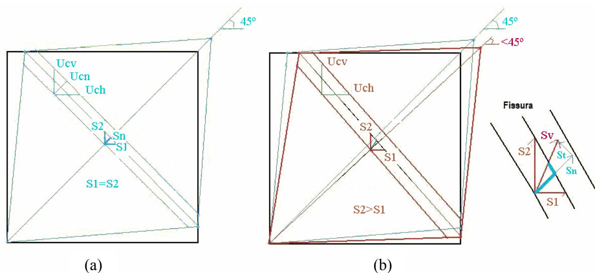
Figura 42: comparação da determinação dos escorregamentos e aberturas de fissura para: (a) painéis com mesma taxa de armadura e (b) painéis com taxas diferentes
