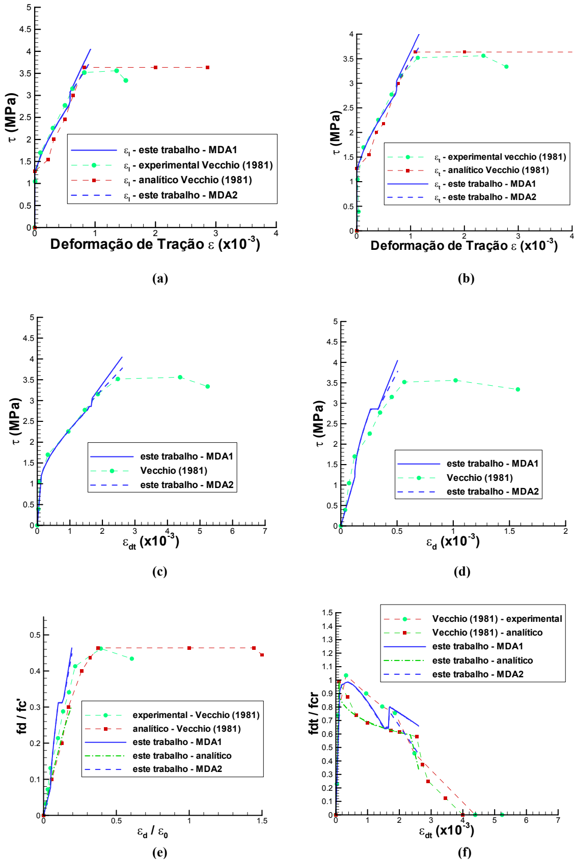
Figura 60: curvas do painel PV11 de (a) \epsilon_l \times \tau ; (b) \epsilon_l \times \tau (c) \epsilon_{dt} \times \tau ; (d) \epsilon_d \times \tau ; (e) deformações x tensões de compressão; (f) deformações x tensões de tração
