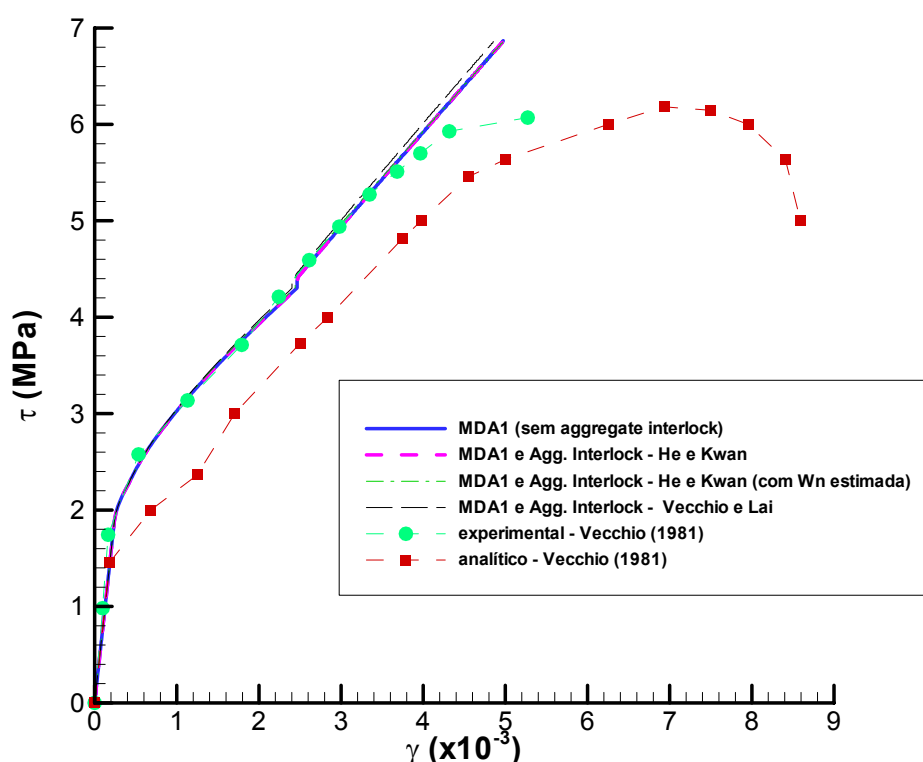
Figura 76: comparação dos modelos de engrenamento dos agregados
