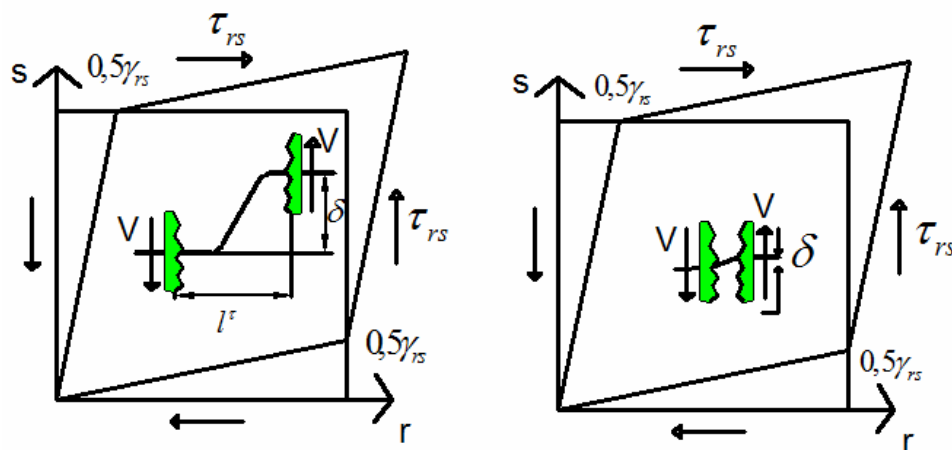
Figura 19: efeito de pino (a) devido à flexão da barra na abertura de fissura e (b) devido ao corte direto da barra (baseada em OLIVER et al., 2008, p. 337)
