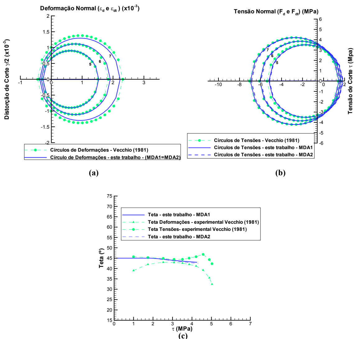
Figura 67: curvas do painel PV21: (a) Círculos de Mohr de Deformações; (b) Círculos de Mohr de Tensões; (c) variação do ângulo das tensões e deformações
