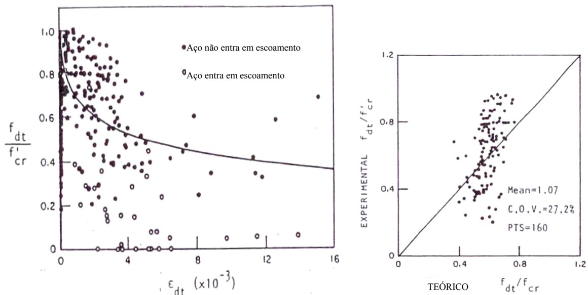
Figura 6: (a) dados obtidos de tensão-deformação de tração e (b) comparação entre valores experimentais e previstos de tensões de tração (VECCHIO, 1981, p. 86 e 89)
