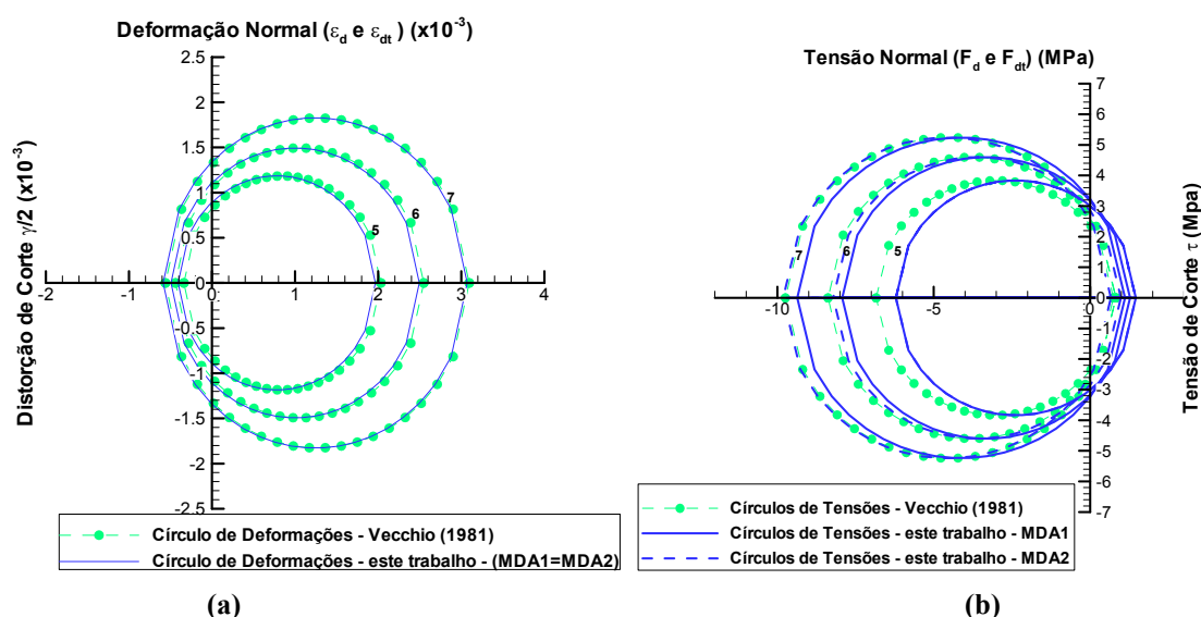
Figura 73: curvas do painel PV14: (a) Círculos de Mohr de Deformações; (b) Círculos de Mohr de Tensões
