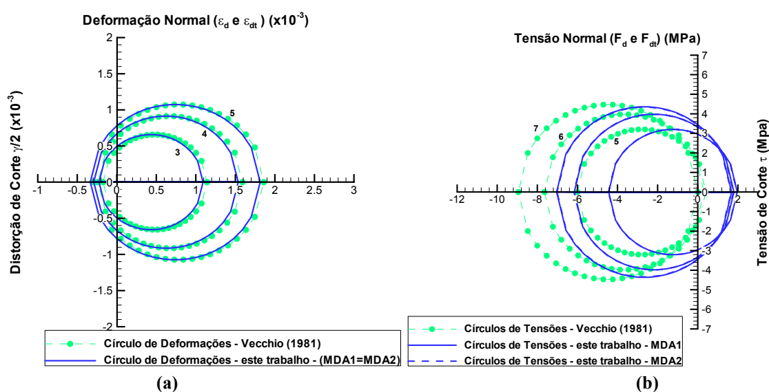
Figura 64: curvas do painel PV6: (a) Círculos de Mohr de Deformações; (b) Círculos de Mohr de Tensões
