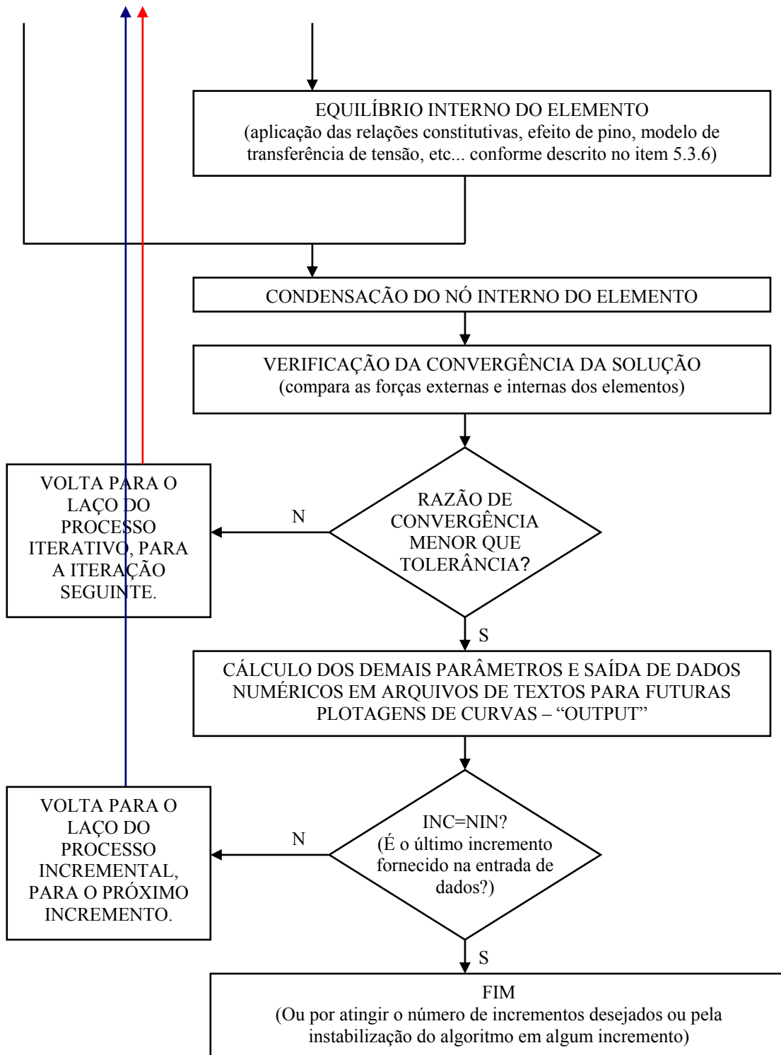
Figura A2: organograma do algoritmo do presente trabalho (parte 2)
