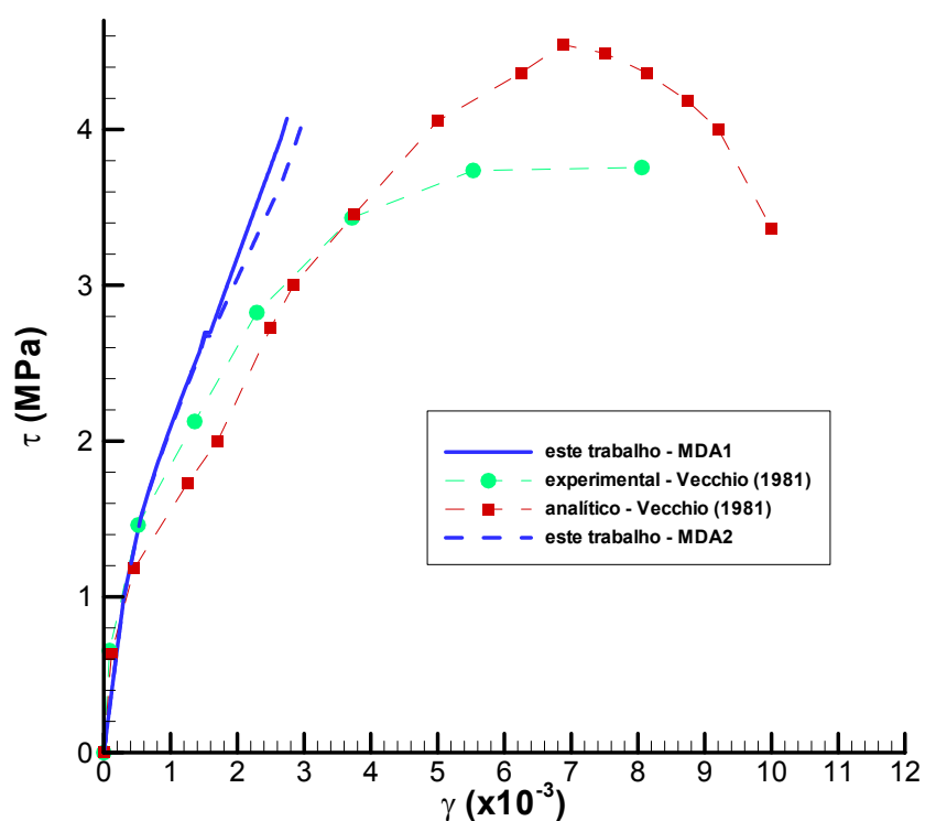
Figura 56: curva tensão x distorção do painel PV9
