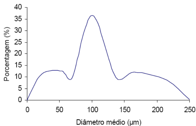
Figura 25 – Distribuição por frequência de tamanho das partículas de ferro usadas nos corpos de prova (JESUS, 2005).
