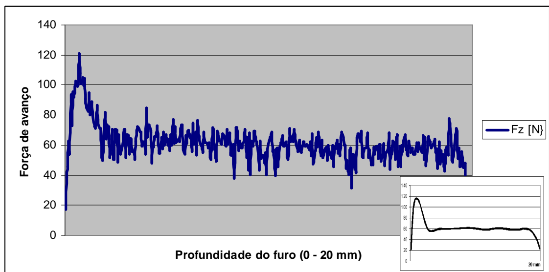
Figura 107 – Força de avanço para resina com 30% de carga e velocidade de corte igual a 100 m/min.
