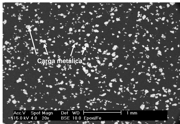
Figura 43 – Distribuição da carga metálica – partículas de ferro – em um corte horizontal no centro da espessura do corpo de prova de resina epóxi com 10% de carga metálica (MEV – BSE)
