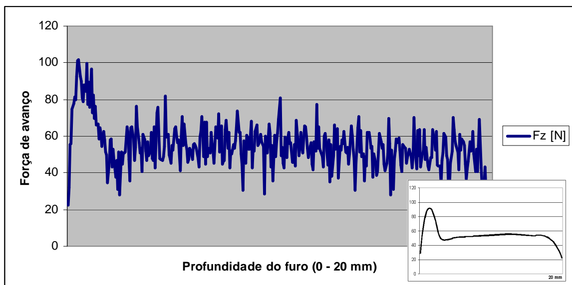
Figura 103 – Força de avanço para resina com 10% de carga e velocidade de corte igual a 100 m/min.
