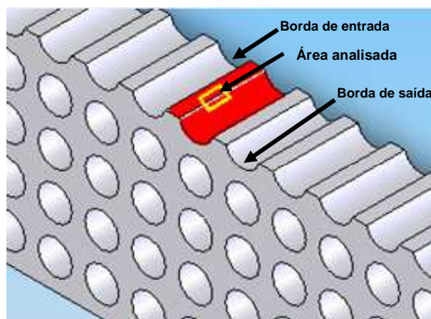
Figura 45 – Corte do corpo de prova para analisar a integridade da superfície do furo.
