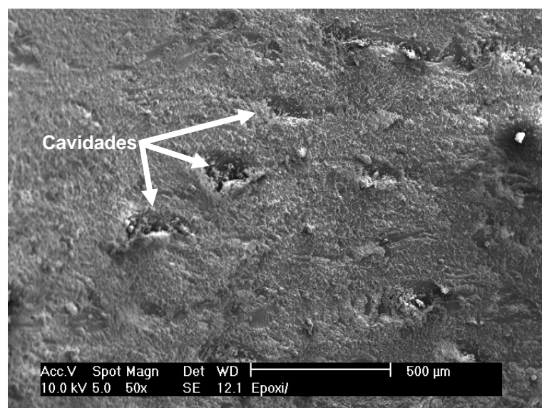
Figura 51 - Micrografia da resina epóxi na metade do furo com aumento de 50x. Resina sem carga metálica e v_c 50 m/min.
