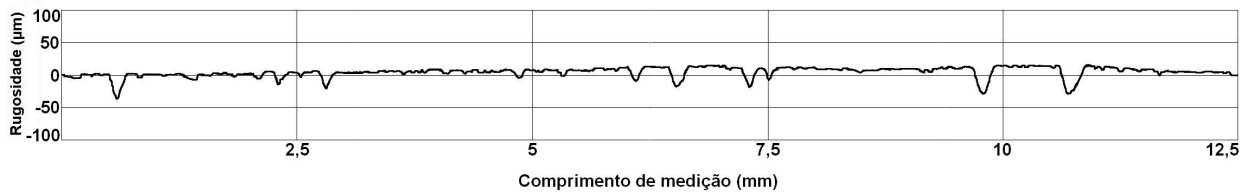
Figura 59 – Perfil de rugosidade da superfície da parede do furo, após ensaio de furação, da resina epóxi com 0% de carga metálica e v_c de 100 m/min.
