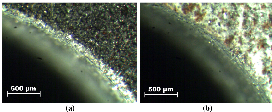
Figura 89 – Resina epóxi com 30% de carga de pó de ferro, v_c 50 m/min. (a) entrada do furo, (b) saída do furo.
