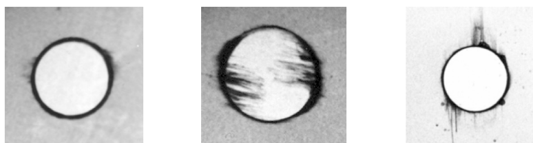
Figura 19 – Radiografia de peças furadas com: a) broca helicoidal; b) broca Dagger ; c) broca com ponta em W (DURÃO et al. 2006).
