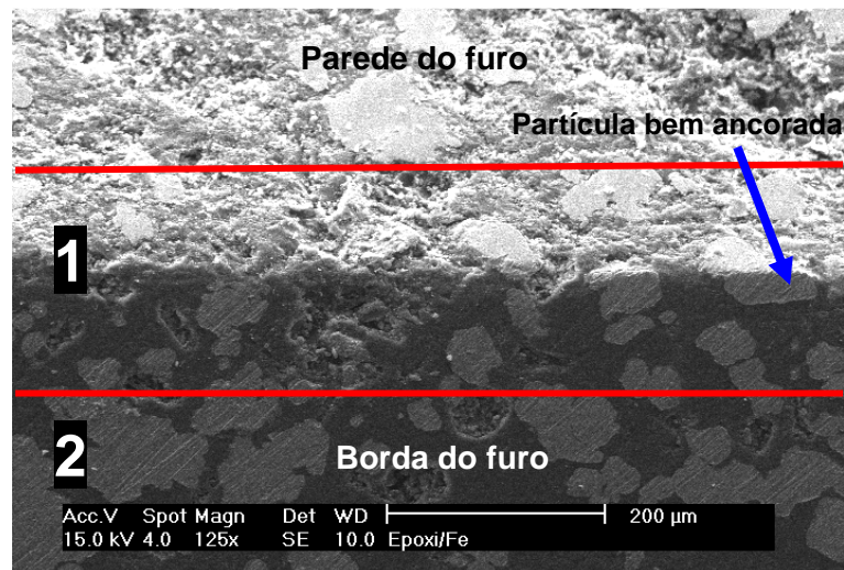
Figura 47 – Amostra do corpo de prova com 30% de carga metálica. A integridade da superfície não foi afetada durante a furação.
