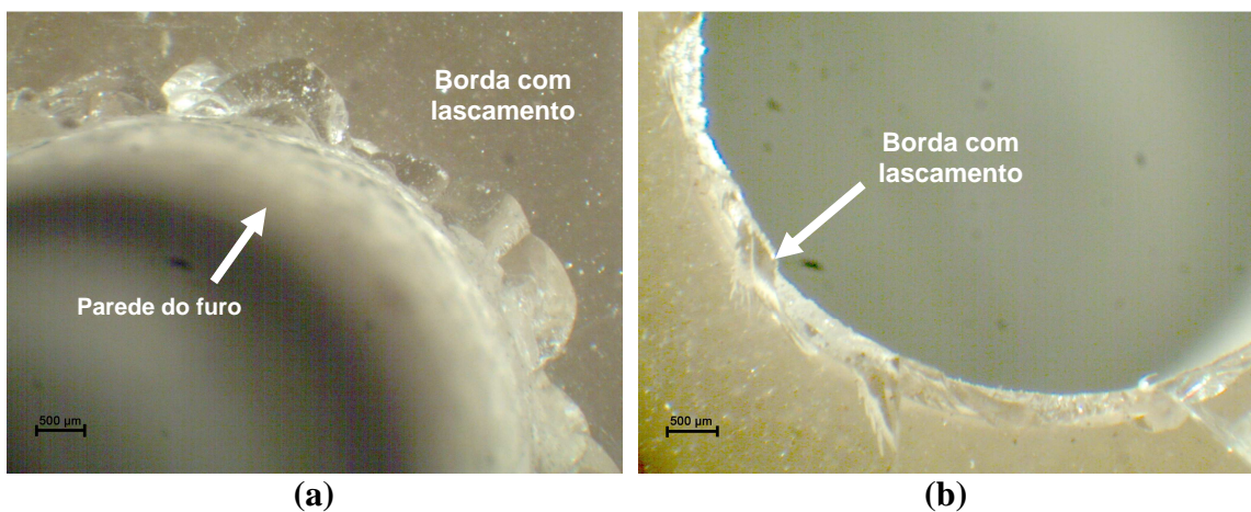
Figura 68 – Resina epóxi com 0% de carga de pó de ferro, v_c 50 m/min. (a) entrada do furo, (b) saída do furo.
