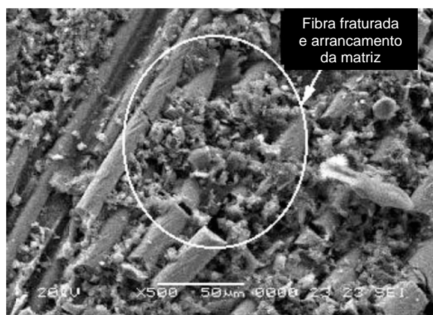
Figura 22 – Imagem feita por um microscópio eletrônico por varredura mostrando o arrancamento e quebra das fibras de um material compósito após a usinagem (PALANIKUMAR, 2006).
