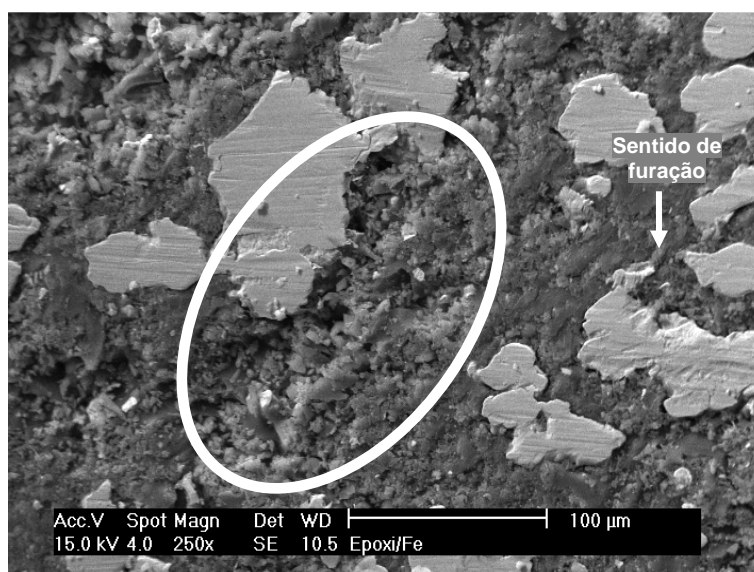
Figura 91 - Microestrutura da resina epóxi/Fe na metade do furo com aumento de 250x. Resina com 30% de carga metálica e v_c 100 m/min.
