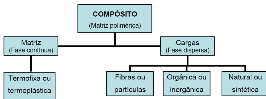
Figura 1 – Esquema de formação de um material compósito [17].
