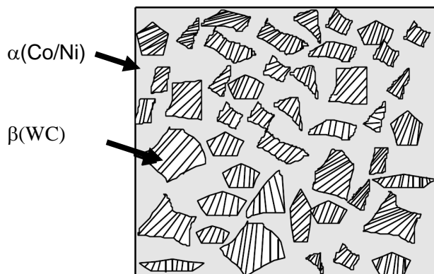
Figura 8 - Constituintes presentes na estrutura do metal-duro em duas fases, alfa e beta (SANDVIK, 2000).
