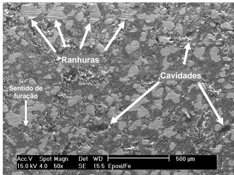
Figura 83 - Micrografia da resina epóxi/Fe na metade do furo com aumento de 50x. Resina com 30% de carga metálica e v_c 50 m/min.
