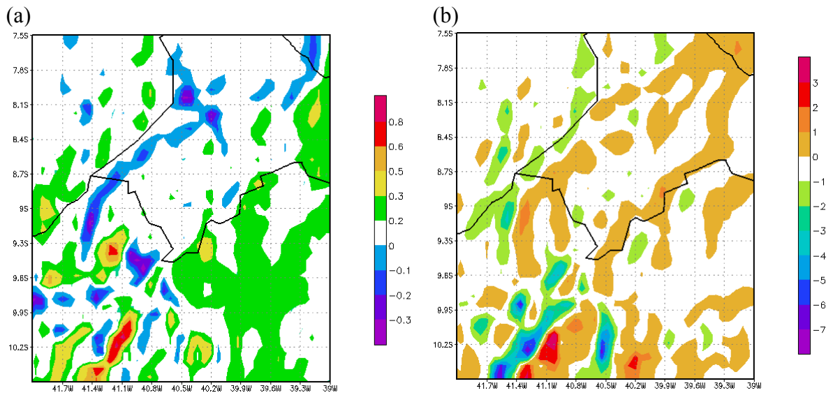
Figura 26 – Advecção média na Grade 2 às 15:00UTC para o período de 08 a 12 de novembro de 2004 de: a)advecção de umidade ( \text{g.kg}^{-1}.\text{h}^{-1} ) b) advecção de temperatura ( ^{\circ}\text{C}.\text{h}^{-1} )
