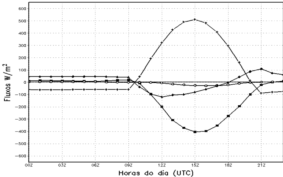
Figura 22 – Média dos Fluxos de Calor Latente (círculo aberto), Calor Sensível (retângulo), Calor no Solo (losango), saldo de radiação (cruz) do período de 17 a 21 de julho de 2004 para o ponto de latitude 9°S e longitude 40°30'W em Wm^{-2}
