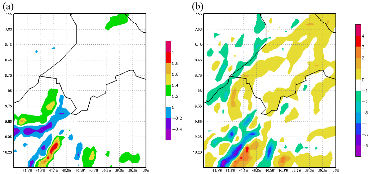
Figura 25 – Advecção média na Grade 2 às 15:00UTC para o período de 17 a 21 de julho de 2004 de: a)advecção de umidade ( \text{g.kg}^{-1}.\text{h}^{-1} ) b) advecção de temperatura ( ^{\circ}\text{C}.\text{h}^{-1} )
