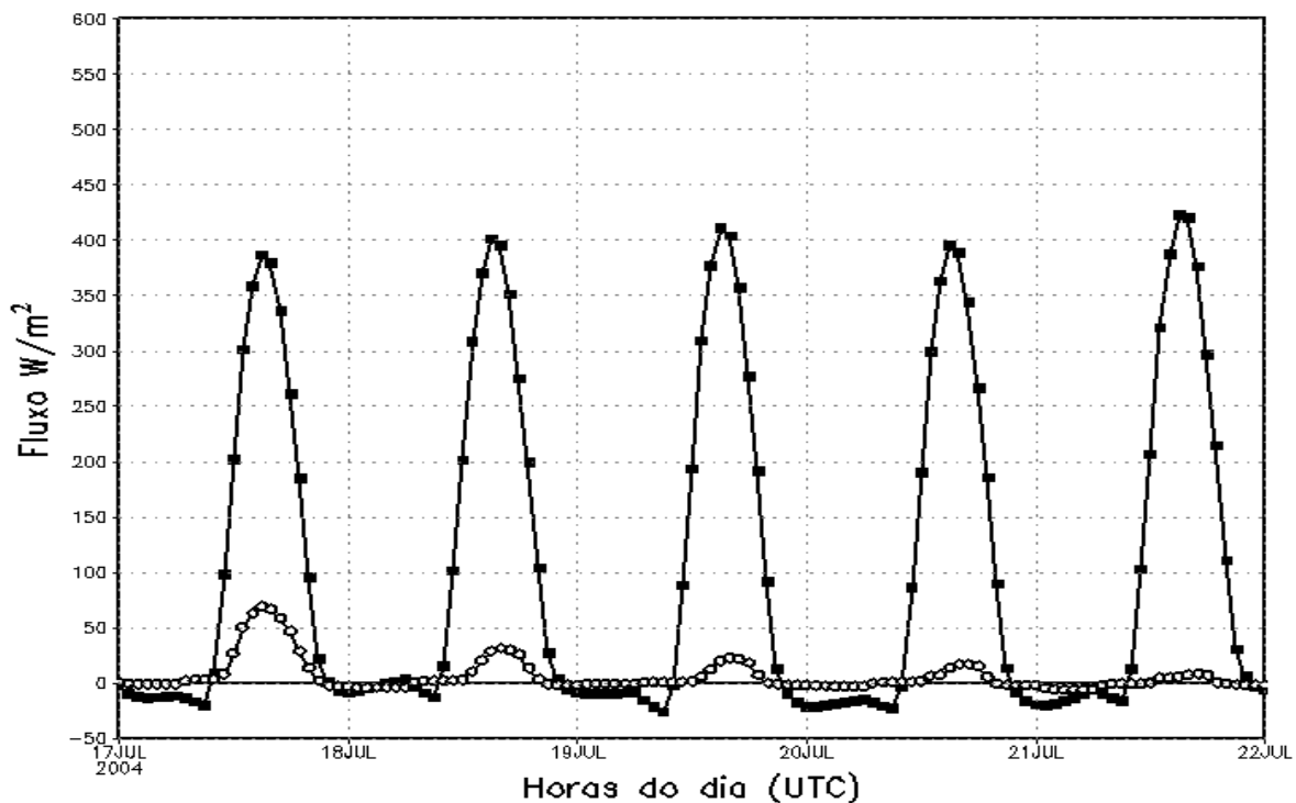
Figura 14 – Fluxos de Calor Latente (circulo aberto), Calor Sensível (quadrado) simulado para o período de 17 a 21 de julho de 2004 para o ponto de latitude 9^{\circ}S e longitude 40^{\circ}30'W em Wm^{-2}
