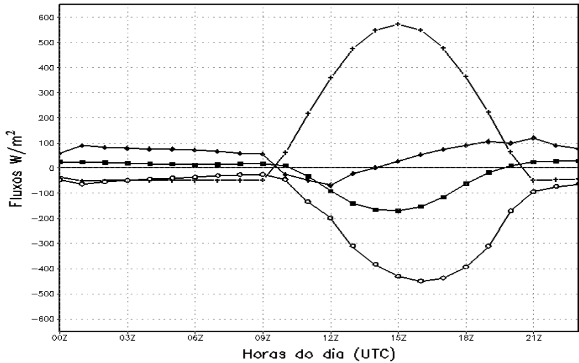
Figura 21 – Média dos Fluxos de Calor Latente (círculo aberto), Calor Sensível (retângulo), Calor no Solo (losango), saldo de radiação (cruz) do período de 18 a 22 de julho de 1999 para o ponto de latitude 9°S e longitude 40°30'W em Wm^{-2}
