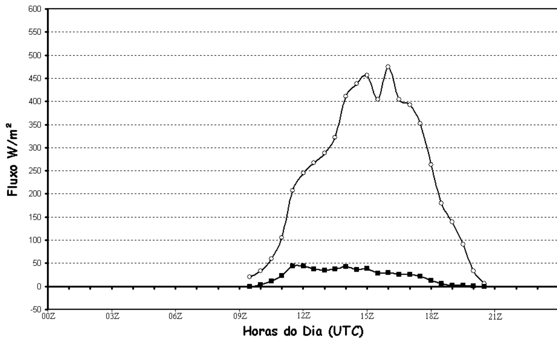
Figura 7 – Média dos Fluxos de Calor Latente (circulo aberto) e Calor Sensível (quadrado fechado) do período de 18 a 22 de julho de 1999 em Wm^{-2}
