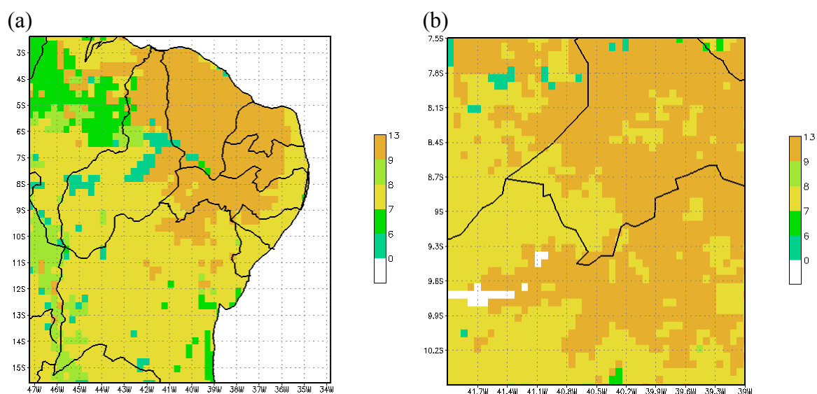
Figura 4 – Tipo de cobertura do solo para a região segundo o modelo: (a)Na Grade 1, (b)Na Grade 2
