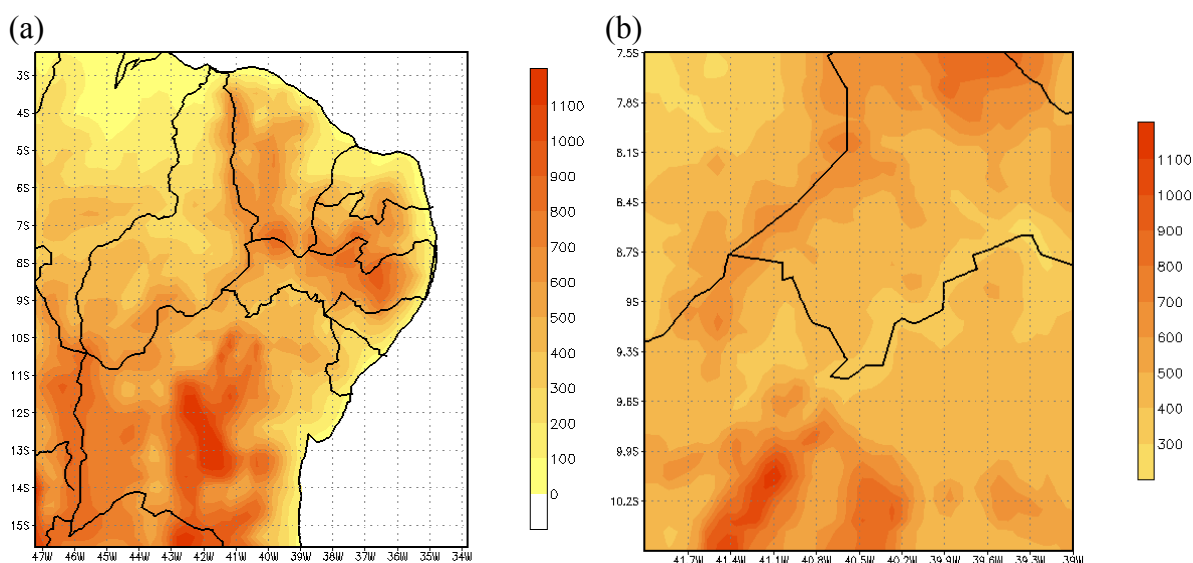
Figura 5 – Topografia para a região segundo o modelo: (a)Na Grade 1, (b)Na Grade 2
