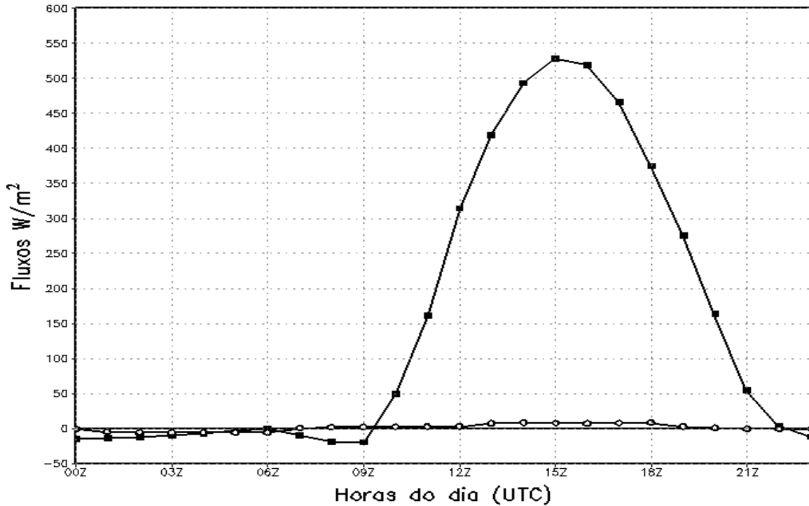
Figura 17 – Média dos Fluxos de Calor Latente (circulo aberto), Calor Sensível (quadrado) do período de 08 a 12 de novembro para o ponto de latitude 9°S e longitude 40°30' W em Wm^{-2}
