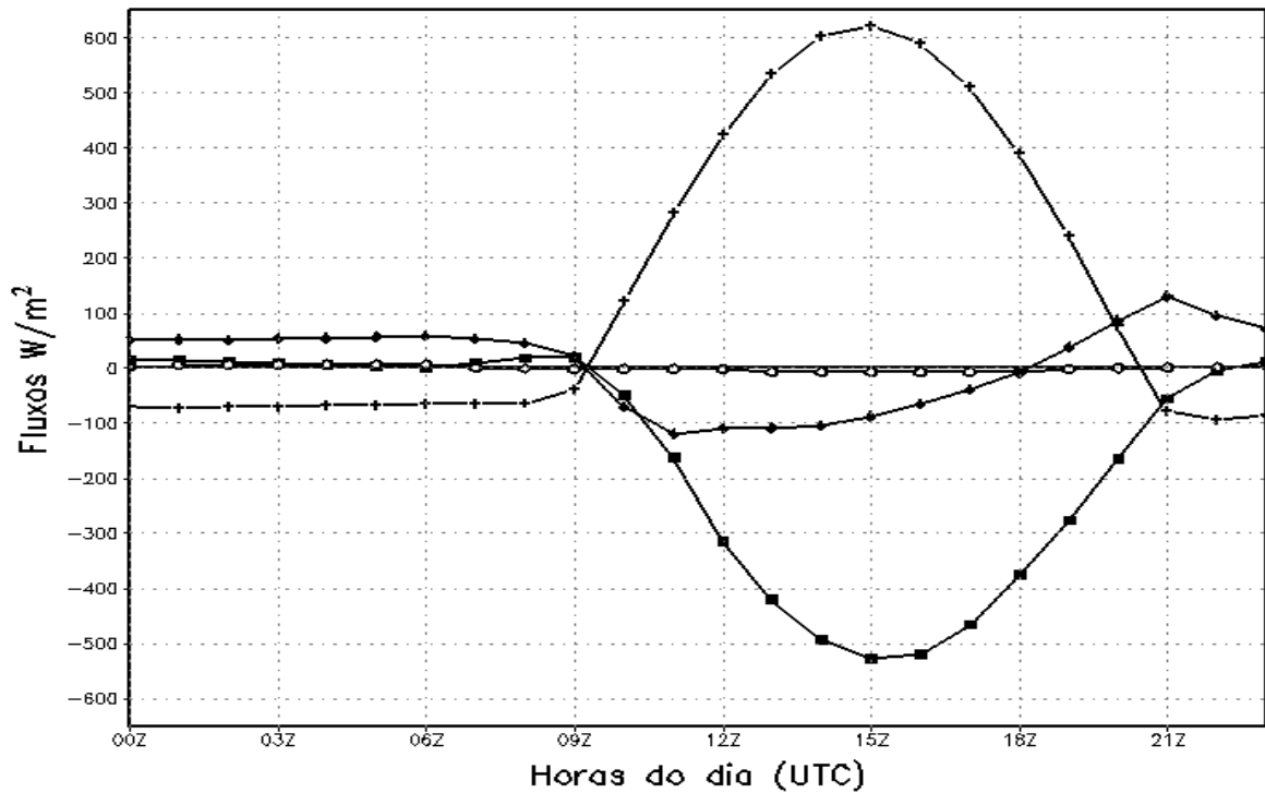
Figura 23 – Média dos Fluxos de Calor Latente (círculo aberto), Calor Sensível (retângulo), Calor no Solo (losango), saldo de radiação (cruz) do período de 08 a 12 de novembro de 2004 para o ponto de latitude 9°S e longitude 40°30' W em Wm^{-2}
