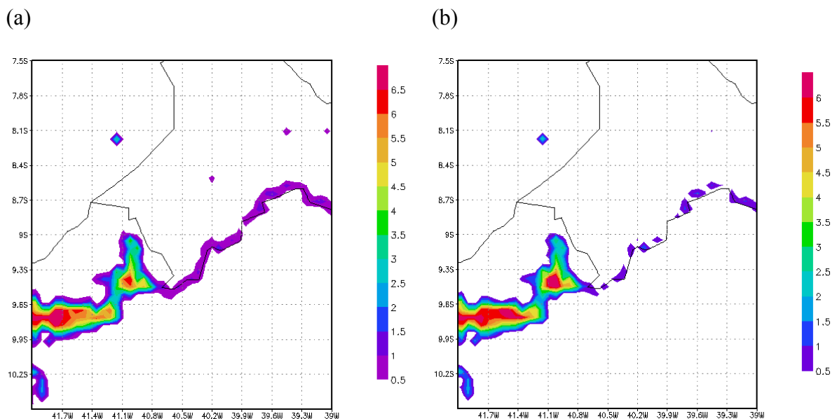
Figura 24 – Evapotranspiração (mm/dia) média na Grade 2 a) para o período de 17 a 21 de julho de 2004 e b) para o período de 08 a 12 de novembro de 2004
