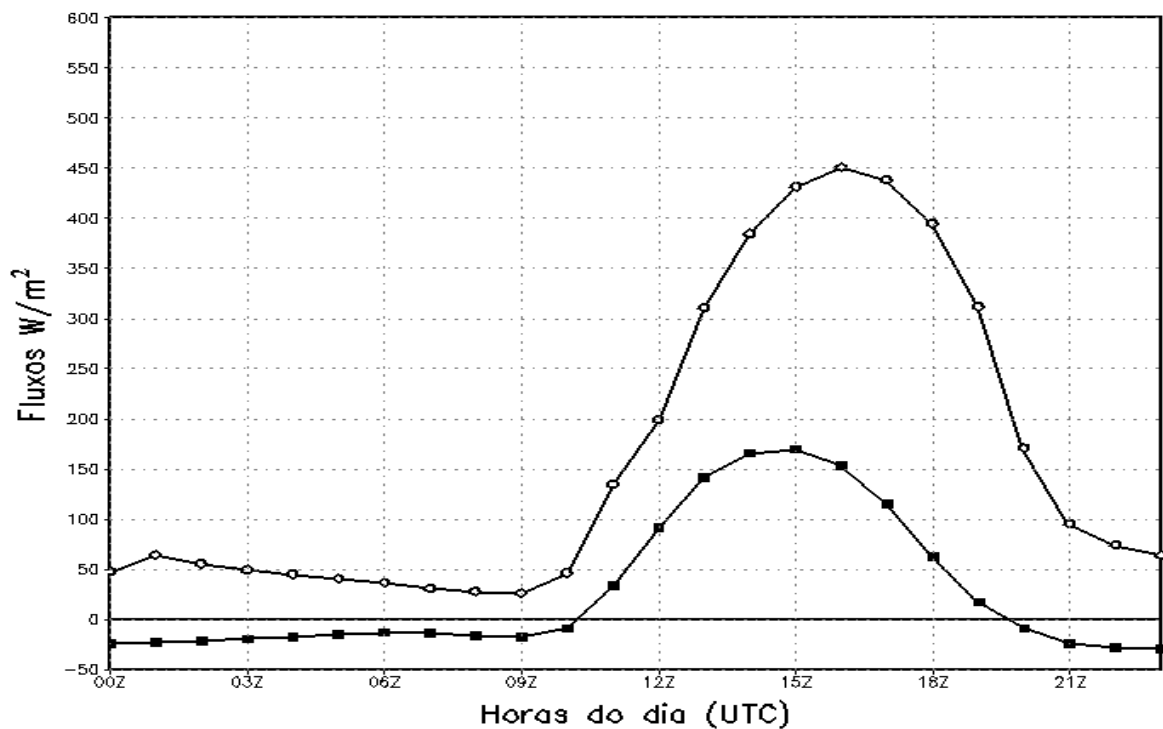
Figura 13 – Média dos Fluxos de Calor Latente (circulo aberto), Calor Sensível (quadrado) do período de 18 a 22 de julho de 1999 para o ponto de latitude 9°S e longitude 40°30'W em Wm -2
