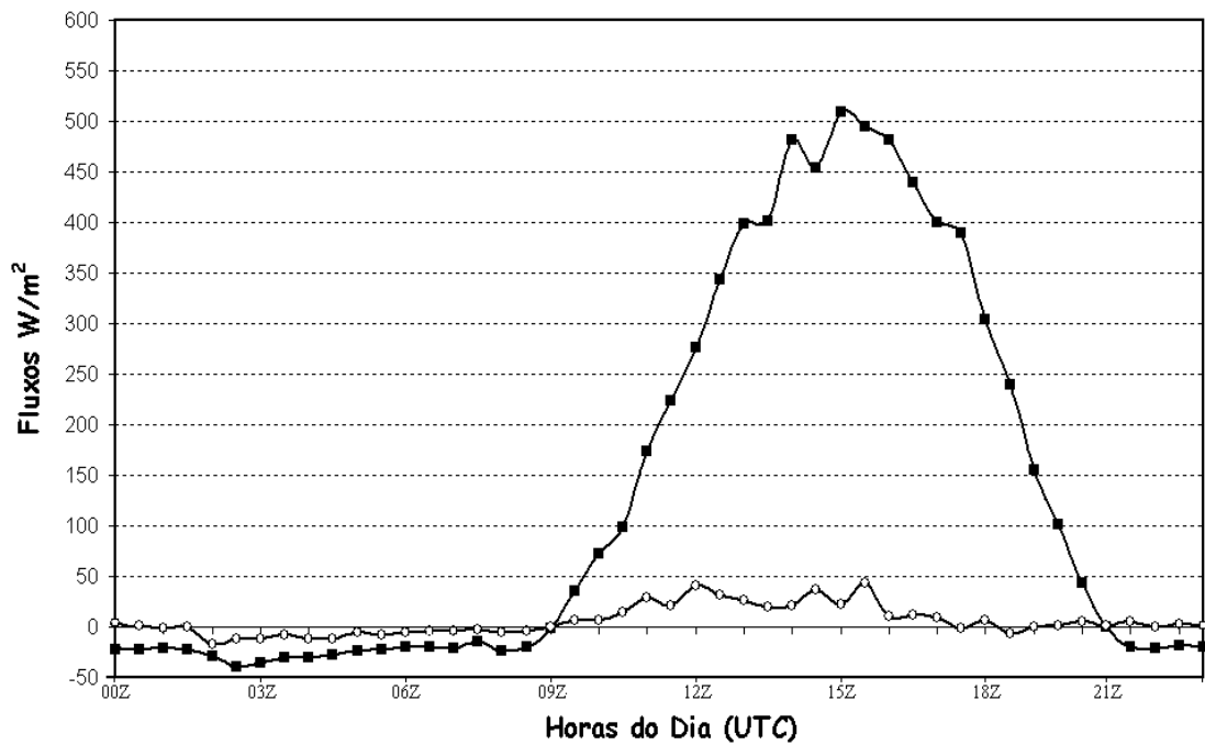
Figura 11 – Média dos Fluxos de Calor Latente (circulo aberto) e Calor Sensível (quadrado fechado) do período de 08 a 12 de novembro de 2004 em Wm^{-2}
