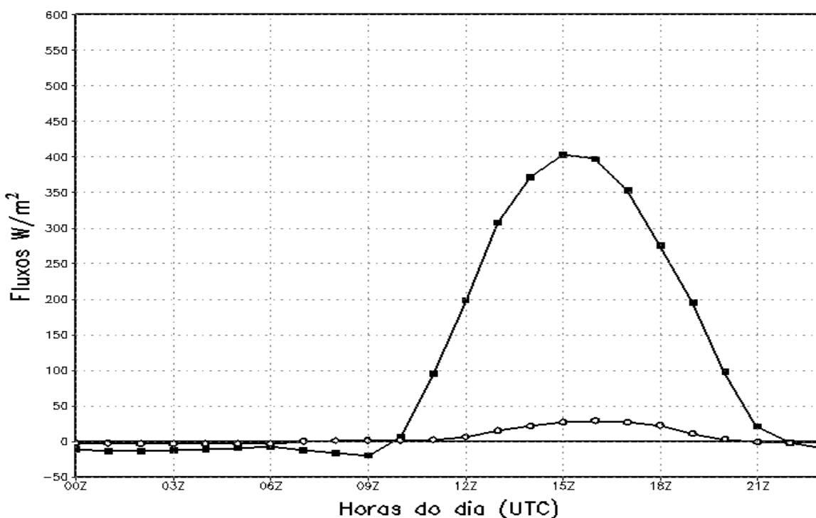
Figura 15 – Média dos Fluxos de Calor Latente (circulo aberto), Calor Sensível (quadrado) do período de 17 a 21 de julho de 2004 para o ponto de latitude 9^{\circ}S e longitude 40^{\circ}30'W em Wm^{-2}
