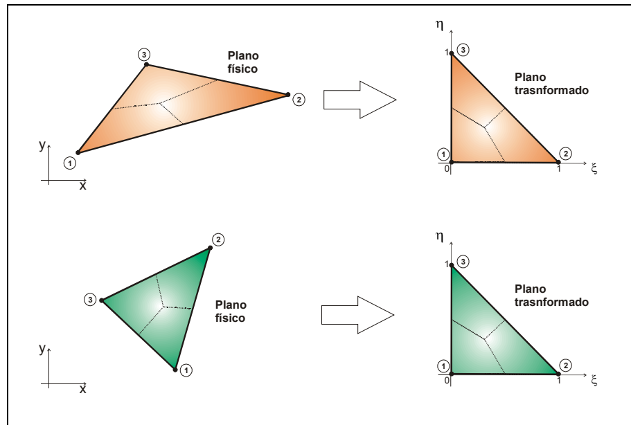
Figura 3.2 - Representação de elementos triangulares nos planos físico e transformado. Fonte: Schubert (2006).
