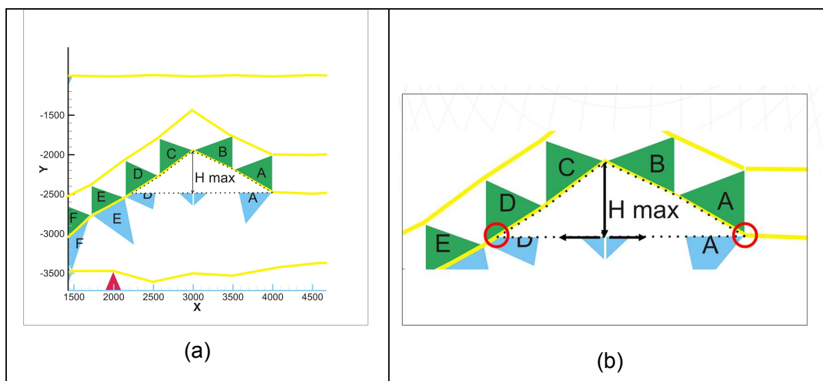
Figura 3.9 – (a) Capacidade máxima que pode ser armazenada na área de drenagem determinada pelo H_{m\acute{a}x} . (b) Determinação das coordenadas limítrofes do reservatório.
