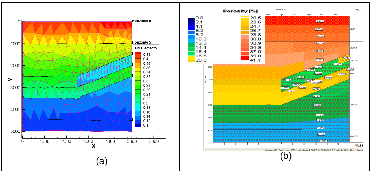
Figura 5.25 - Porosidade
