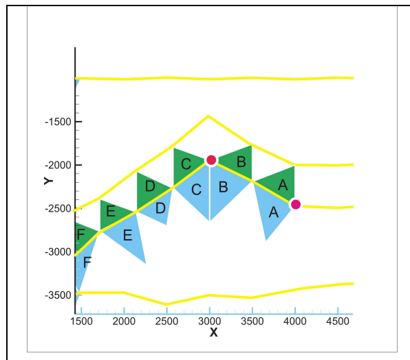
Figura 3.24 – Definição de uma área de drenagem, ponto em vermelho marcando ponto mais alto, ponto cor magenta representando ponto de derramamento, as letras representam os pares de elementos que formam os segmentos das interfaces.
