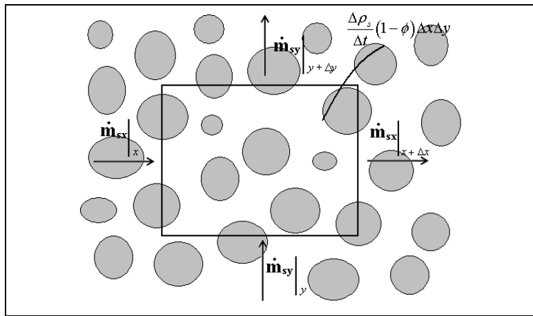
Figura 2.13 – Balanço de massa em um volume de controle para um meio poroso
