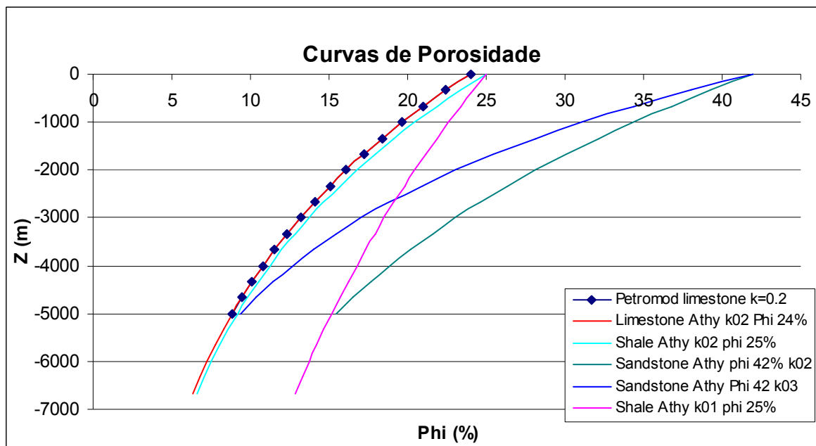
Figura 2.9 – Curva da Variação da Porosidade com a profundidade. As densidades dos materiais Sandstone , Shale e Limestone são respectivamente: 2660 kg/m 3 , 2680 kg/m 3 e 2710 kg/m 3 . Curva em vermelho sobrepõe a curva de losangos azuis escuros mostrando a similaridade entre curvas do software PETROMOD e SiBa 2008.
