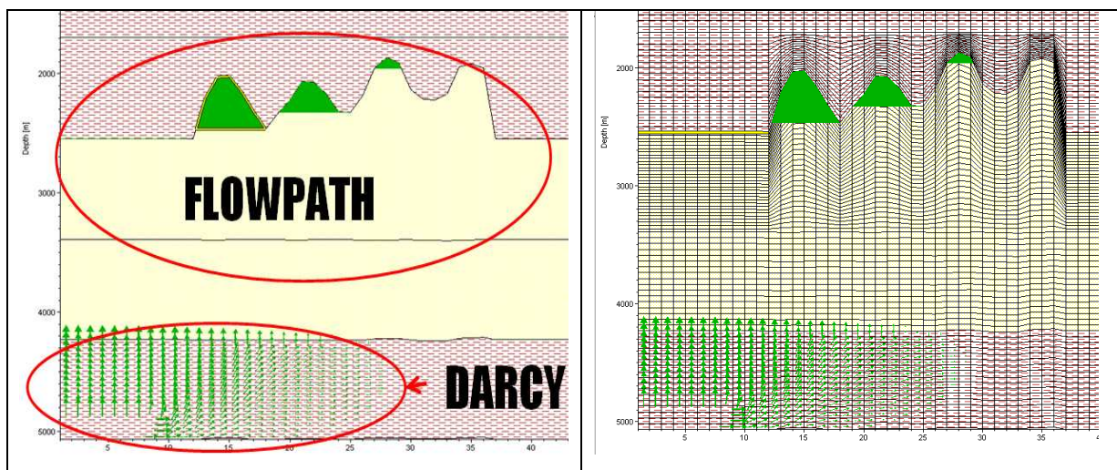
Figura 3.5 - Método Híbrido.
