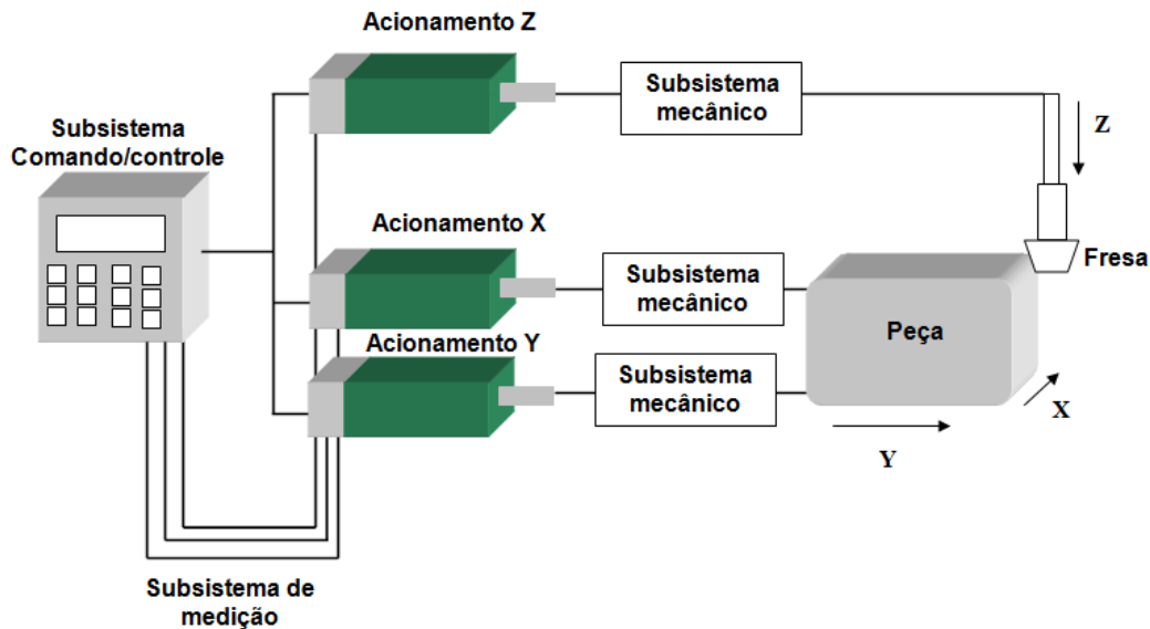
Figura 4.4 - Esquematização de uma idéia de uma máquina automatizada (fresadora).
