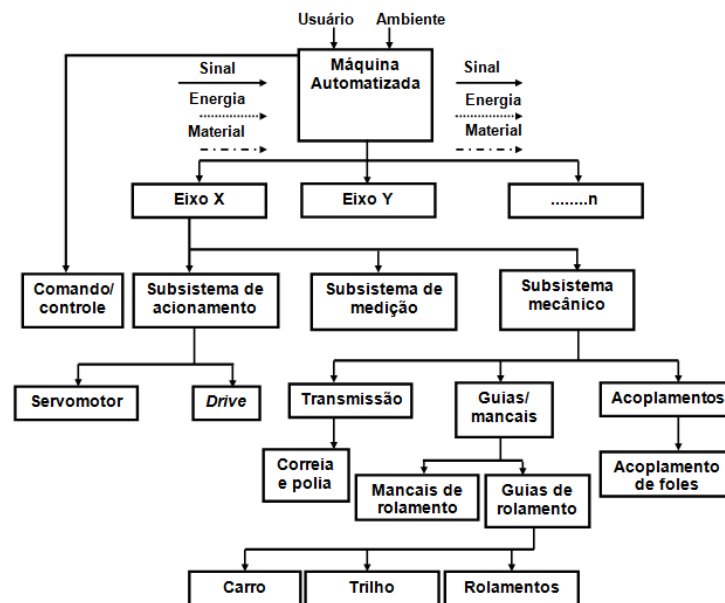
Figura 4.14 - Desdobramento de uma máquina automatizada.
