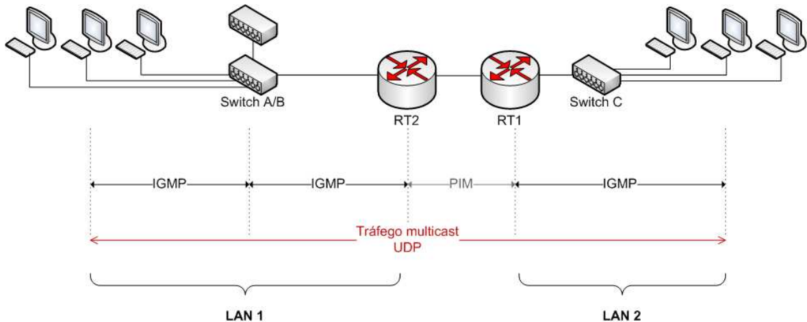
Figura 5.1: Configuração da rede para os experimentos.
