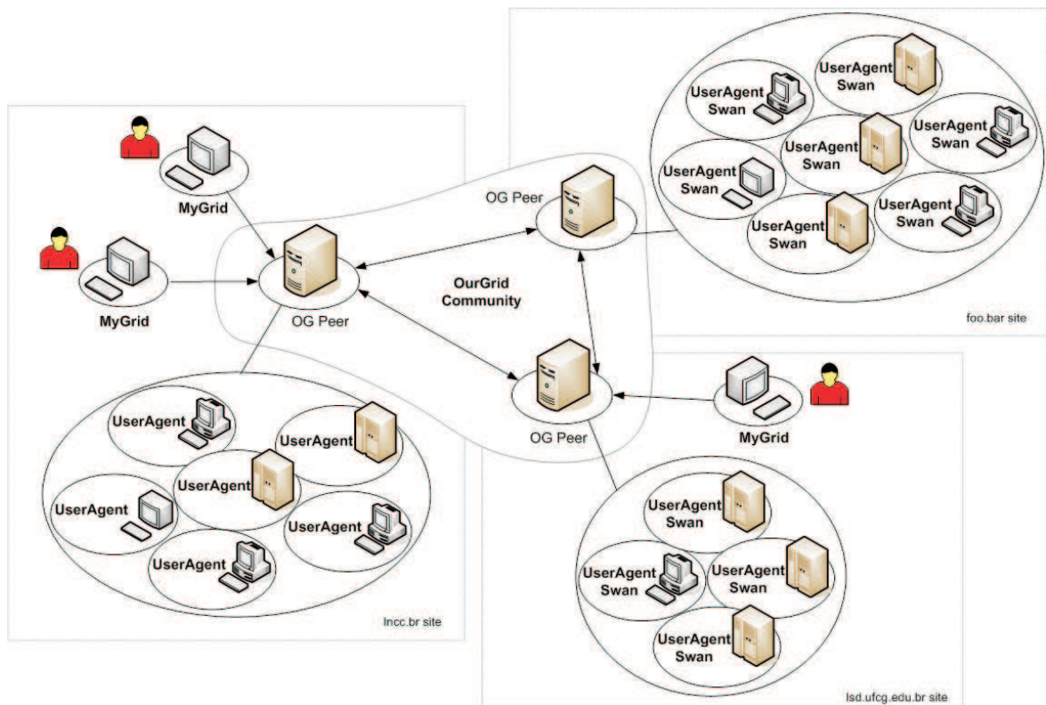
Figura 3.1: Arquitetura do OurGrid (Cirne et al. [21]).
