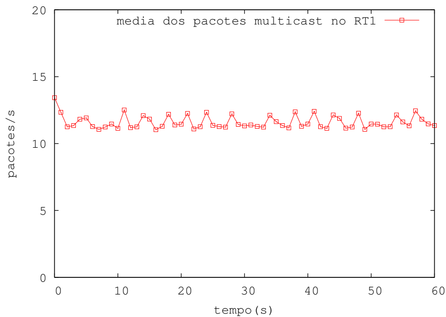
Figura 5.3: Fluxo gerado pela troca de mensagens multicast no roteador RT1.
