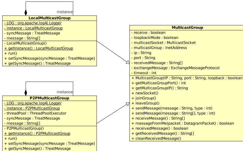
Figura 4.3: Diagrama das classes responsáveis pela formação dos Grupos multicast .
