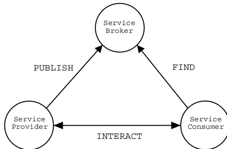
Figura 6.2: Arquitetura orientada a serviço do ICENI Grid Middleware (Furmento et al. [30]).
