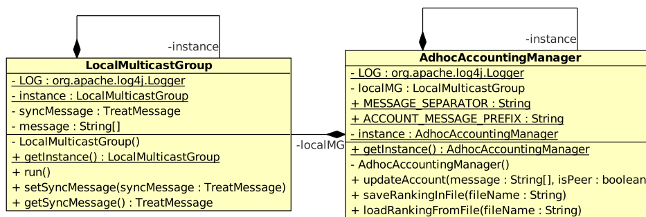
Figura 4.5: Diagrama das classes responsáveis por manter a NoF.
