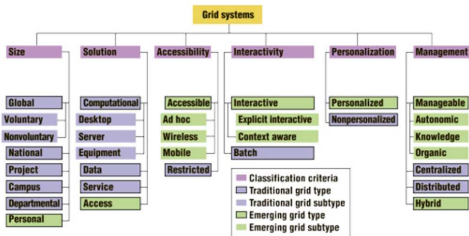
Figura 2.1: Classificação de grades tradicionais e emergentes (Kurdi [41]).
