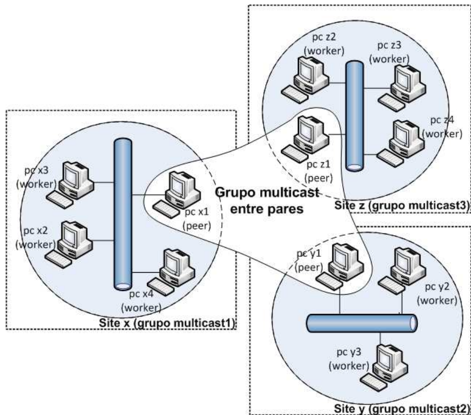
Figura 4.1: Exemplo de uma comunidade no ad hoc Grid
