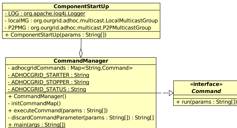
Figura 4.6: Diagrama das classes responsáveis pela inicialização do ad hoc Grid.
