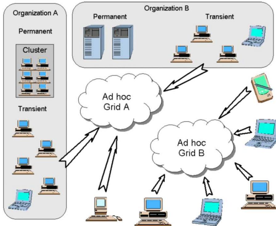
Figura 2.2: Arquitetura de uma grade ad hoc (Smith [51]).
