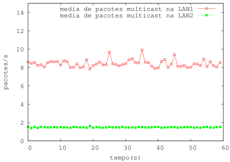
Figura 5.4: Fluxo gerado pela troca de mensagens multicast na LAN1 \times LAN2.
