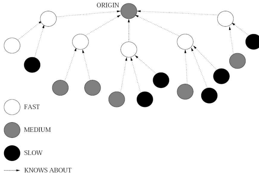
Figura 6.1: Configuração exemplo de uma árvore do Organic Grid (Chakravarti et al. [19]).
