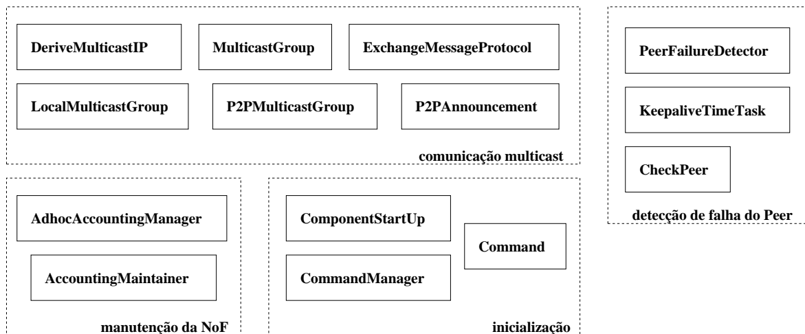
Figura 4.2: Estrutura do ad hoc Grid.
