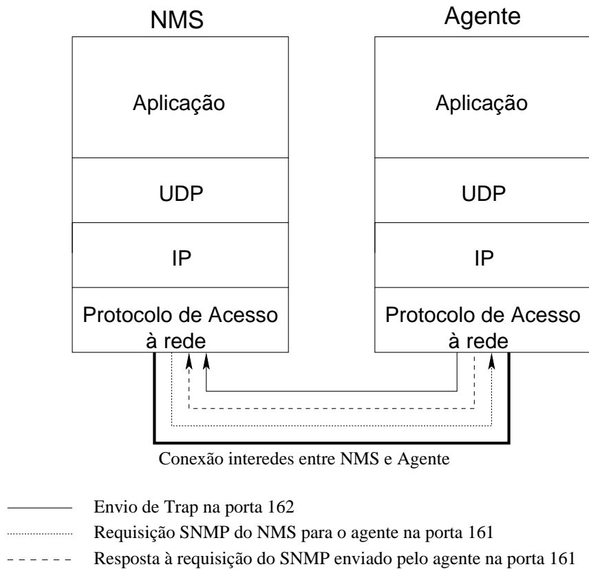
Figura 5.2: Comunicação entre NMS e agente (Adaptado de Douglas et al. [42]).
