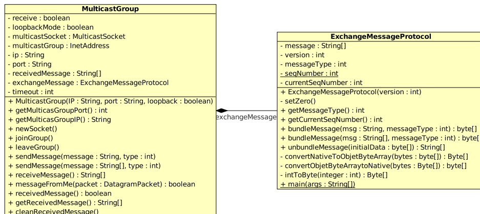
Figura 4.4: Diagrama das classes responsáveis pela troca de mensagens multicast .
