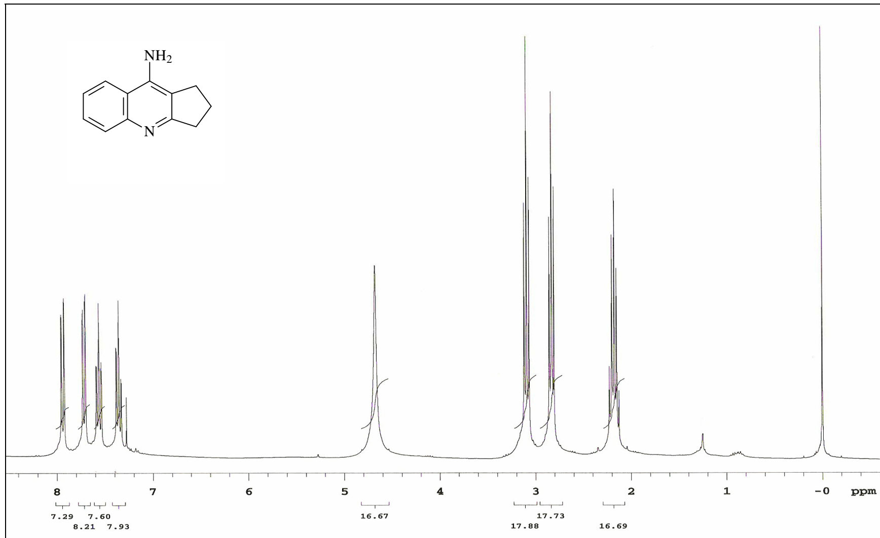
Anexo 4. Espectro de RMN de ^1\text{H} ( \text{CDCl}_3 , 300 MHz) da 9-amino-2,3-di-idro-1H-ciclopenta[1,2- b ]quinolina ( 58 ).
