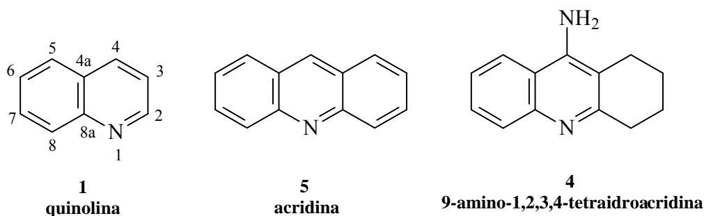
Figura 2. Quinolina ( 1 ), acridina ( 5 ) e 9-amino-1,2,3,4-tetraidroacridina ( 4 ).
