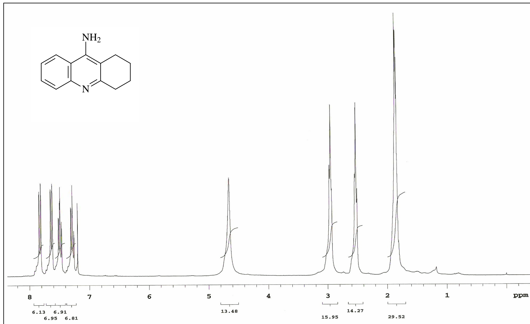
Anexo 1. Espectro de RMN de ^1\text{H} ( \text{CDCl}_3 , 300 MHz) da 9-amino-1,2,3,4-tetraidroacridina ( 4 ).
