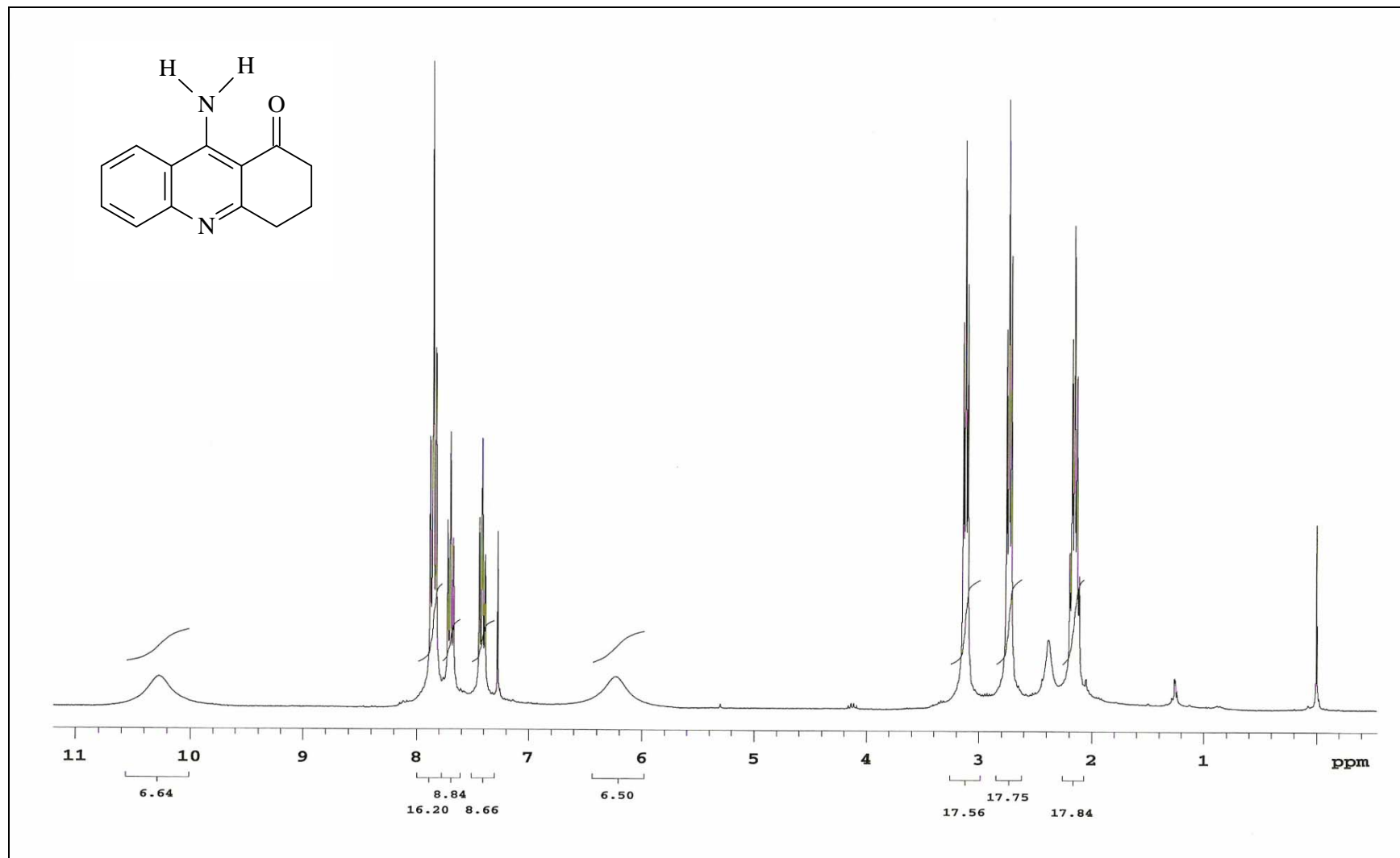
Anexo 10. Espectro de RMN de ^1\text{H} ( \text{CDCl}_3 , 300 MHz) da 9-amino-3,4-di-idroacridin-1(2H)-ona ( 60 ).
