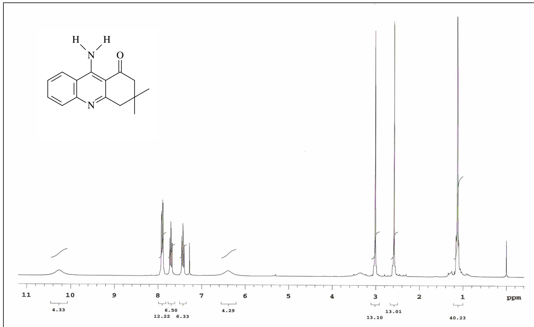
Anexo 13. Espectro de RMN de ^1\text{H} ( \text{CDCl}_3 , 300 MHz) da 9-amino-3,4-di-idro-3,3-dimetilacridin-1(2H)-ona ( 61 ).
