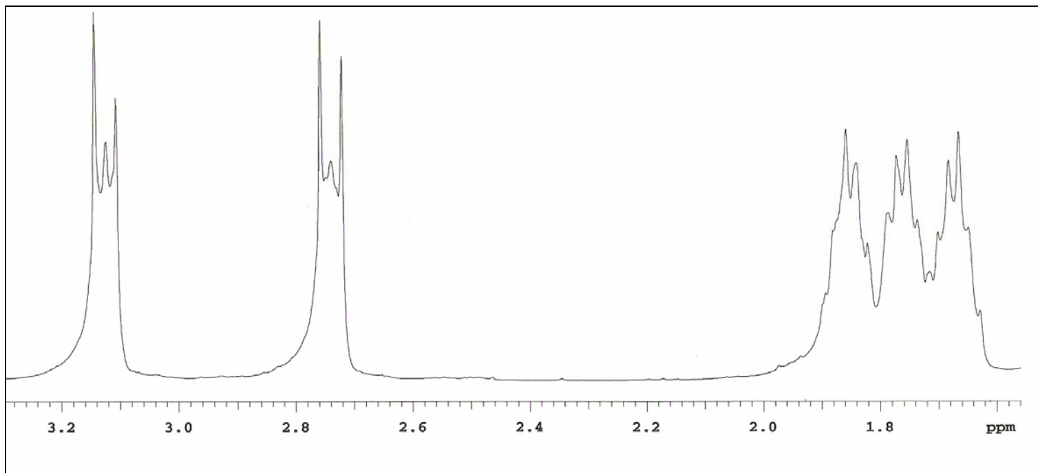
Anexo 8. Ampliação da faixa de 1,6 a 3,2 ppm do espectro de RMN de ^1\text{H} ( \text{CDCl}_3 , 300 MHz) da 11-amino-2,3,4,5-tetraidro-1 H -cicloepa[1,2- b ]quinolina ( 59 ).
