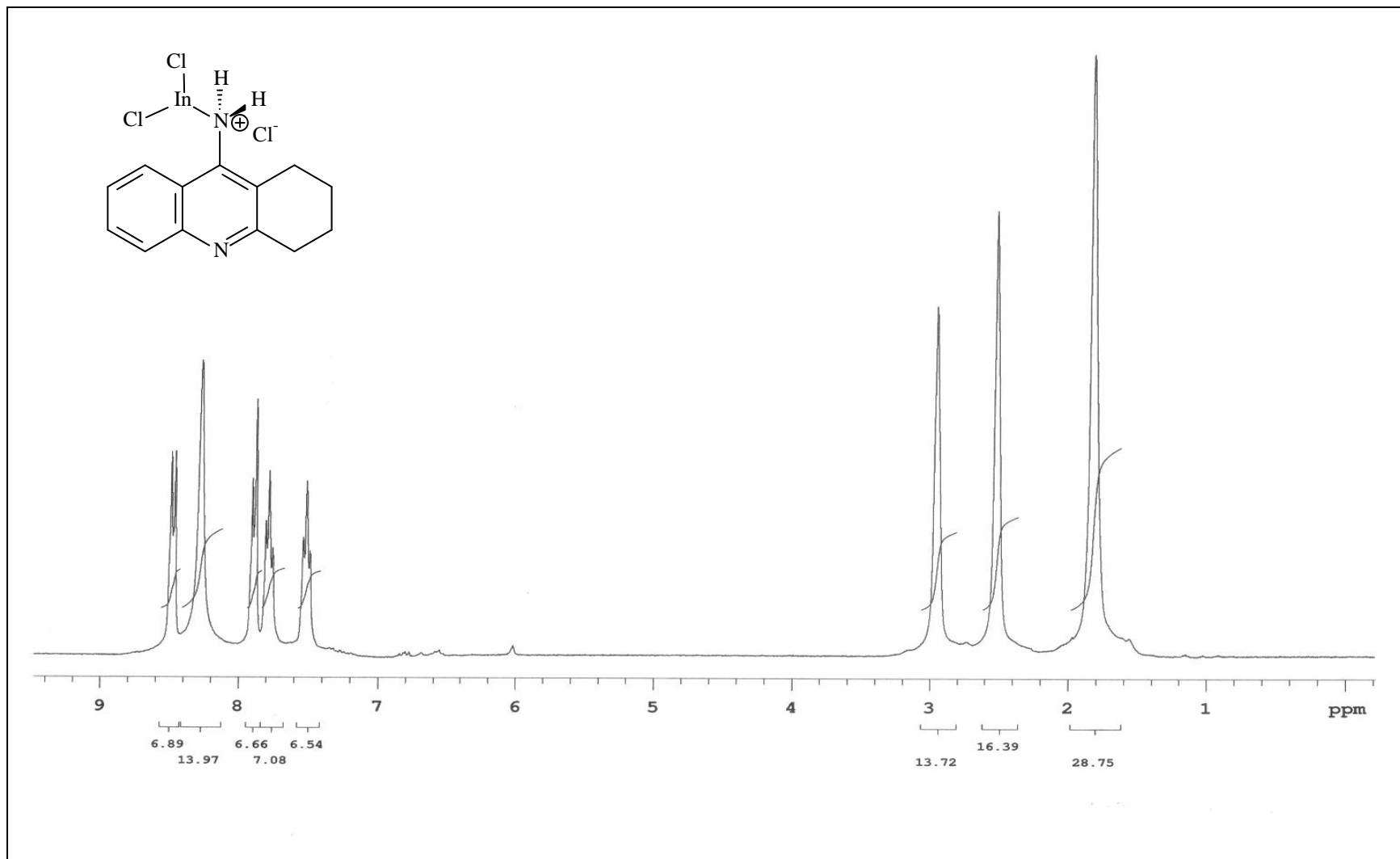
Anexo 20. Espectro de RMN de ^1\text{H} (DMSO- d_6 , 300 MHz) do complexo aminoacridínico 69 .
