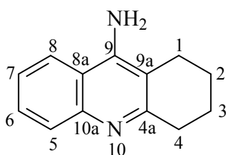
Figura 6. Tacrina ( 4 ).
