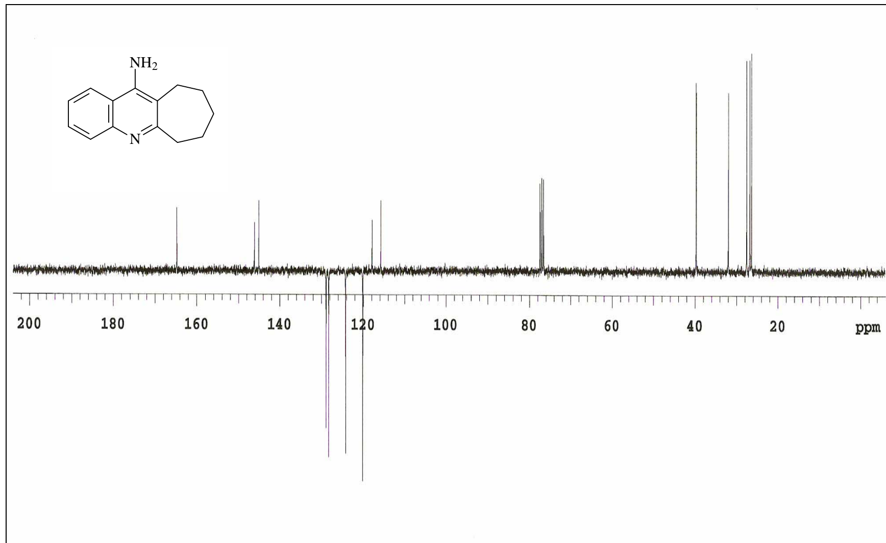
Anexo 9. Espectro de RMN de ^{13}\text{C} (APT) ( \text{CDCl}_3 , 75 MHz) da 11-amino-2,3,4,5-tetraidro-1H-cicloepa[1,2-b]quinolina ( 59 ).
