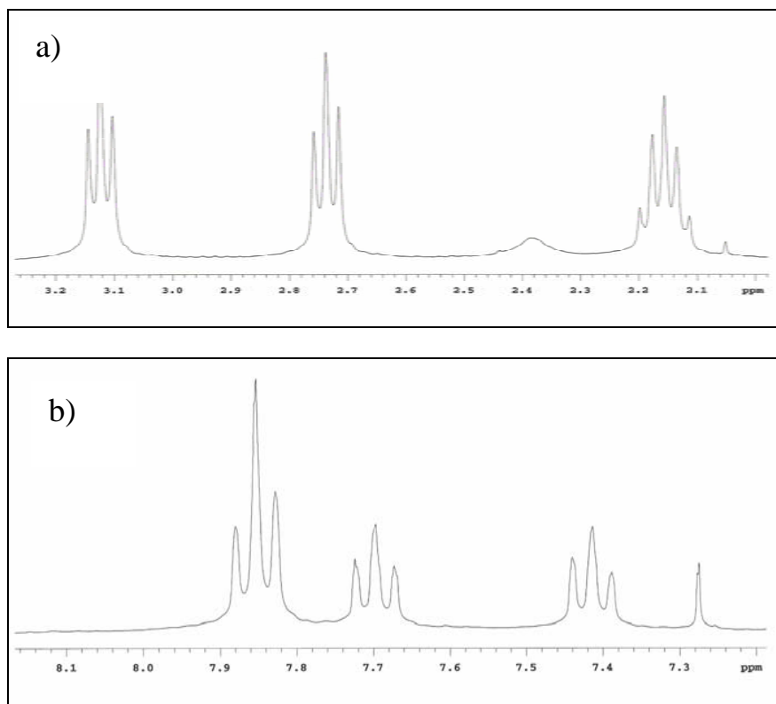
Anexo 11. Ampliações do espectro de RMN de ^1\text{H} ( \text{CDCl}_3 , 300 MHz) da 9-amino-3,4-di-idroacridin-1(2 H )-ona ( 60 ) (a) 2,1 – 3,2 ppm; (b) 7,2 – 7,9 ppm.
