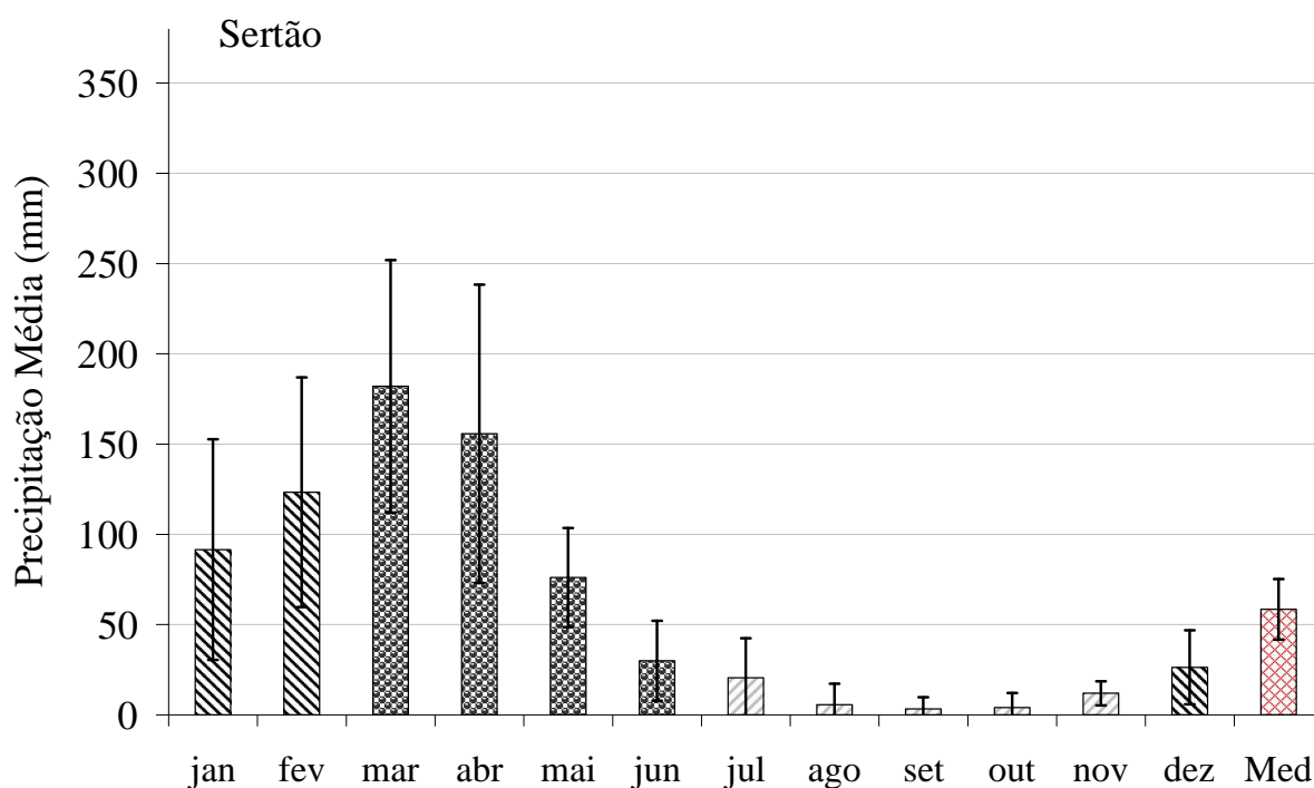
Figura 16. Precipitação média mensal (mm) para a microrregião do Sertão do estado da Paraíba no período de 1975 a 2005, com destaque para pré-estação chuvosa (dez-fev) e estação chuvosa (mar-jun).
