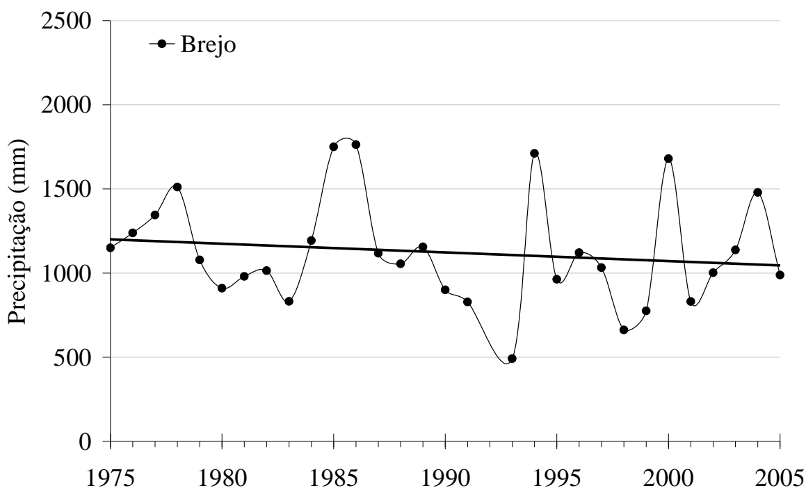
Figura 11. Variabilidade anual da precipitação (mm) para a microrregião do Brejo do estado da Paraíba, e a linha tendência, no período de 1975 a 2005.
