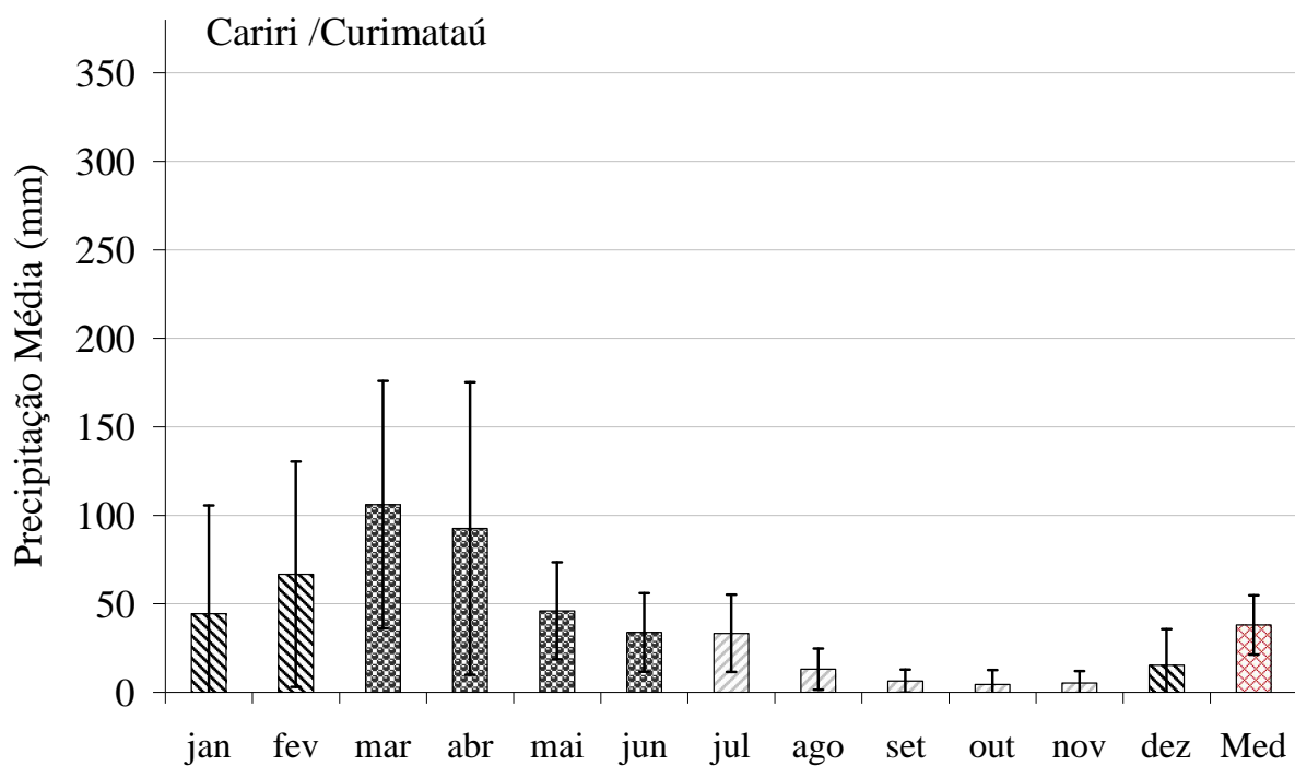
Figura 14. Precipitação média mensal (mm) para a microrregião do Cariri/Curimataú do estado da Paraíba no período de 1975 a 2005, com destaque para pré-estação chuvosa (dez-fev) e estação chuvosa (mar-jun).
