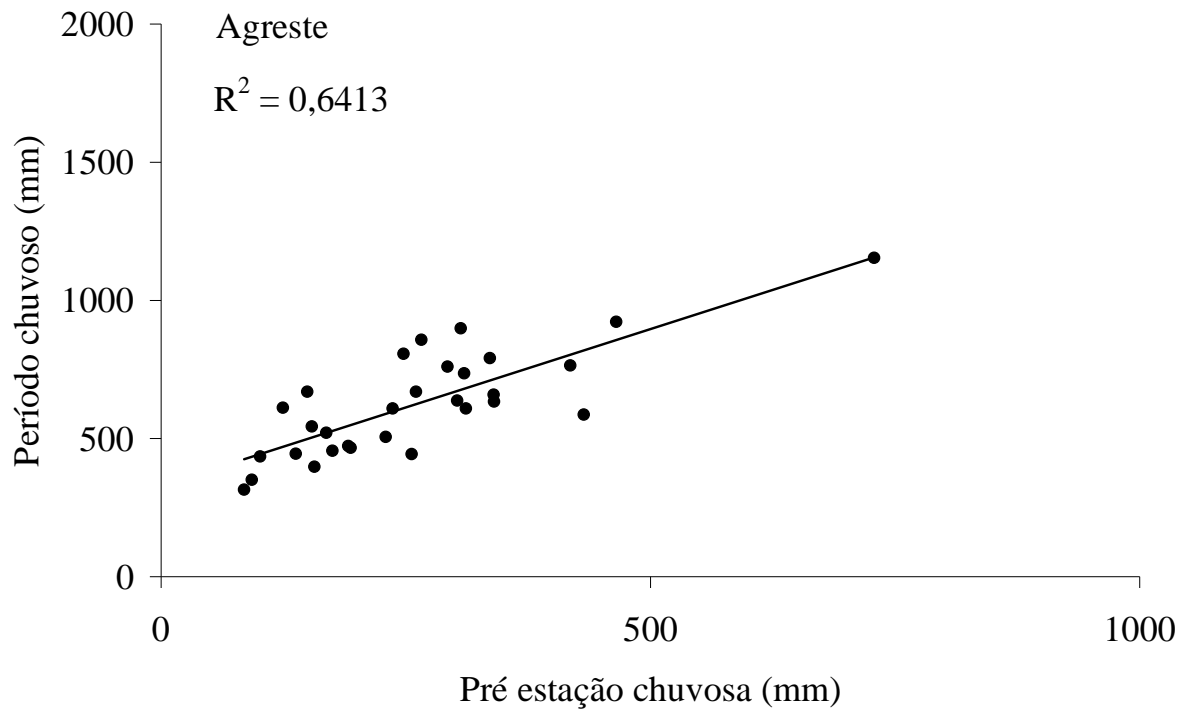
Figura 22. Relação linear entre as precipitações (mm) da pré-estação com a do período chuvoso para a microrregião do Agreste paraibano, no período de 1975 a 2005.
