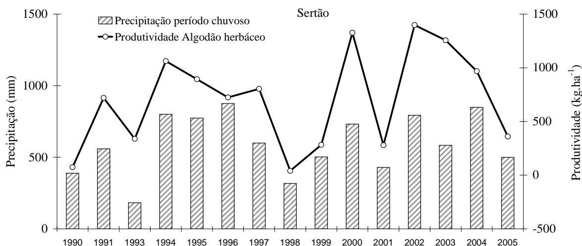
Figura 35. Produtividade anual de Algodão herbáceo (kg ha -1 ) na microrregião do Sertão do estado da Paraíba, no período de 1990 a 2005, e a precipitação pluvial (mm) durante o período chuvoso (Fontes: IBGE e AESA)
