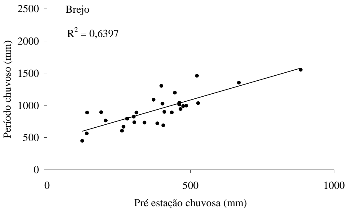
Figura 21. Relação linear entre as precipitações (mm) da pré-estação com a do período chuvoso para a microrregião do Brejo paraibano, no período de 1975 a 2005.
