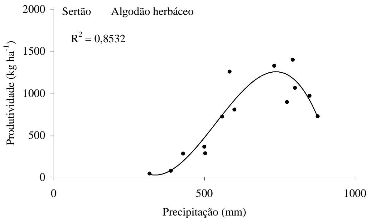
Figura 36. Correlação da precipitação pluvial (milímetro) durante a estação chuvosa com a produtividade do Algodão herbáceo (kg ha -1 ) da microrregião do Sertão do estado da Paraíba, no período de 1990 a 2005
