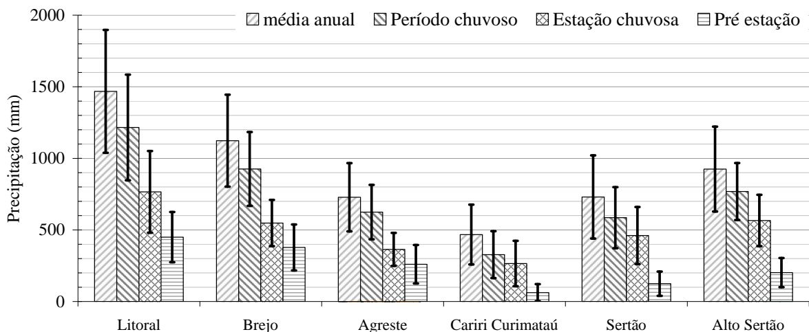
Figura 7. Médias das precipitações (mm) anual, período chuvoso (7 meses), estação chuvosa (4 meses) e pré-estação (3 meses) para as seis microrregiões pluviometricamente homogêneas da Paraíba, no período de 1975 a 2005 e seus respectivos desvios-padrão.
