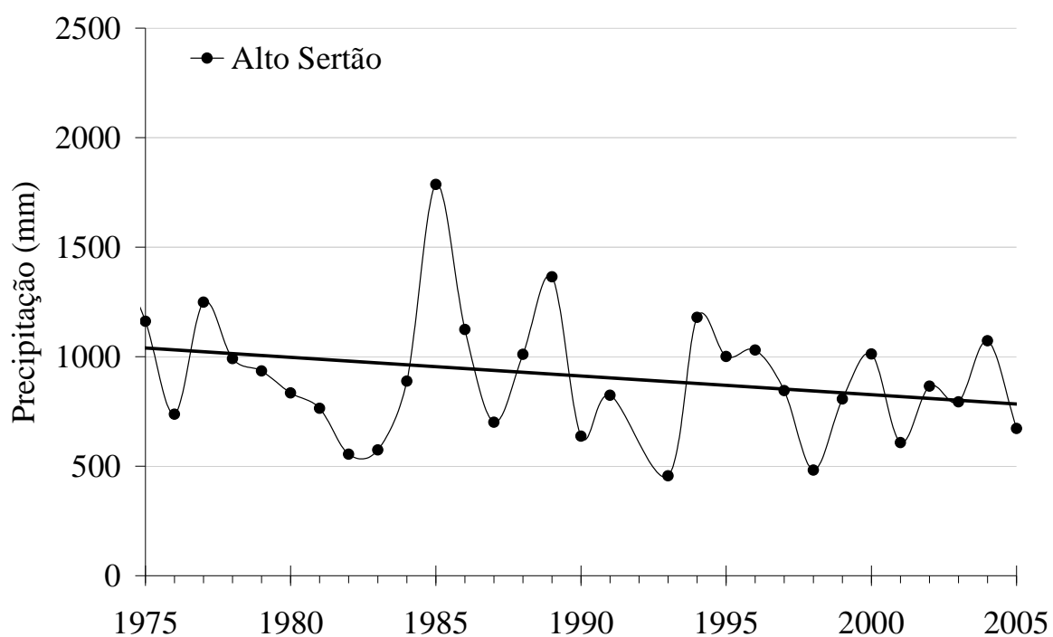
Figura 19. Variabilidade anual da precipitação (mm) para a microrregião do Alto Sertão do estado da Paraíba, e a linha tendência, no período de 1975 a 2005.
