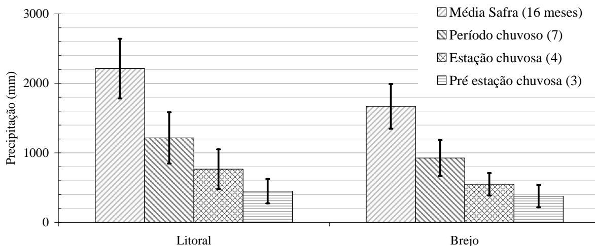
Figura 26. Precipitações médias (mm) da safra (16 meses), período chuvoso (7 meses), estação chuvosa (4 meses) e pré-estação (3 meses), para as microrregiões do Litoral e Brejo da Paraíba, médias de 1975 a 2005. As linhas verticais são os desvios-padrão
