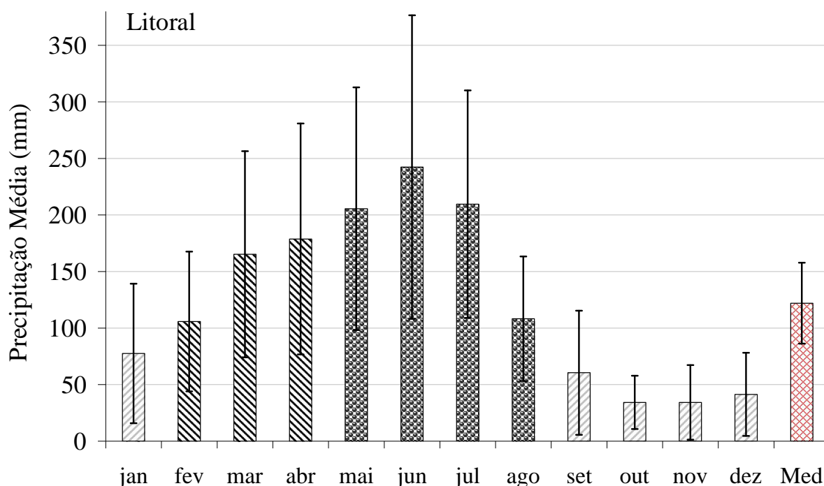
Figura 8. Precipitação média mensal (mm) para a microrregião do Litoral do estado da Paraíba no período de 1975 a 2005, com destaque para pré-estação chuvosa (fev-abr) e estação chuvosa (mai-ago).
