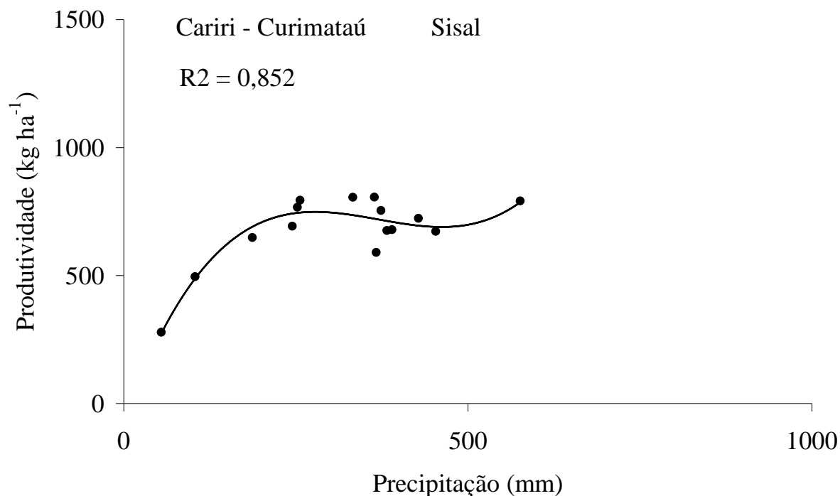
Figura 39. Correlação da precipitação pluvial (milímetro) durante o período chuvoso com a produtividade do Sisal (kg ha -1 ) da microrregião do Cariri/Curimataú do estado da Paraíba, no período de 1990 a 2005.
