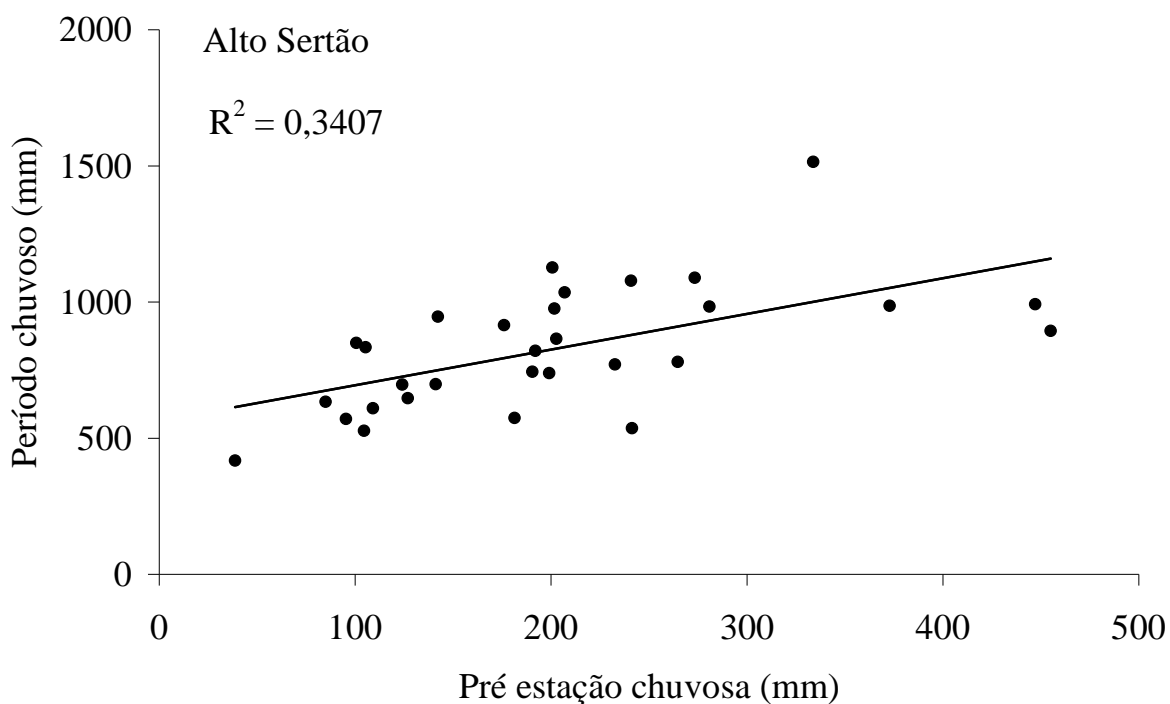
Figura 25. Relação linear entre as precipitações (mm) da pré-estação com a do período chuvoso para a microrregião do Alto Sertão paraibano, no período de 1975 a 2005.
