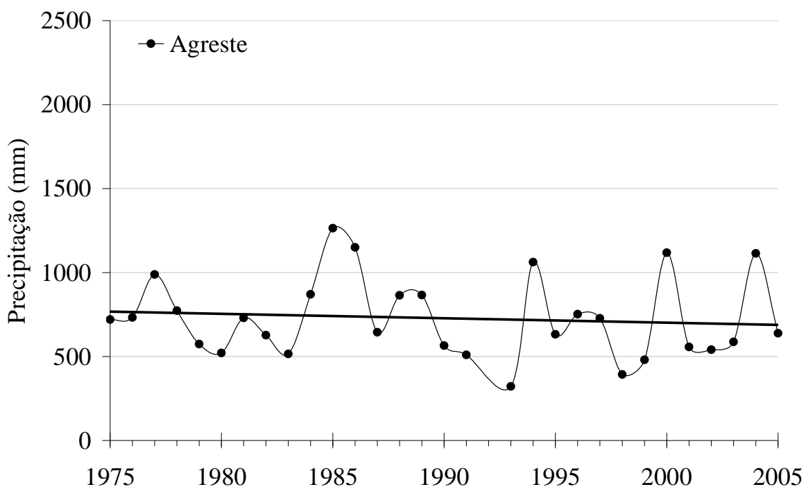
Figura 13. Variabilidade anual da precipitação (mm) para a microrregião do Agreste do estado da Paraíba, e a linha tendência, no período de 1975 a 2005.
