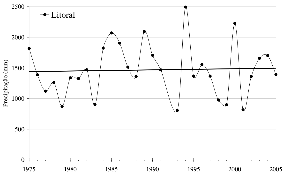
Figura 9. Variabilidade anual da precipitação (mm) para a microrregião do Litoral do estado da Paraíba, e a linha tendência, no período de 1975 a 2005.
