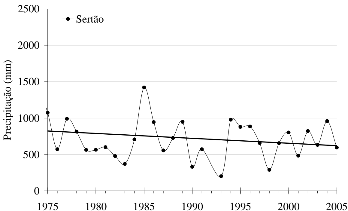
Figura 17. Variabilidade anual da precipitação (mm) para a microrregião do Sertão do estado da Paraíba, e a linha tendência, no período de 1975 a 2005.
