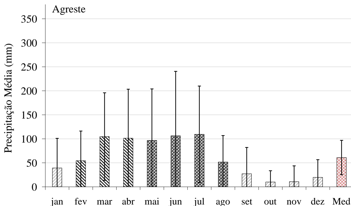
Figura 12. Precipitação média mensal (mm) para a microrregião do Agreste do estado da Paraíba no período de 1975 a 2005, com destaque para pré-estação chuvosa (fev-abr) e estação chuvosa (mai-ago).
