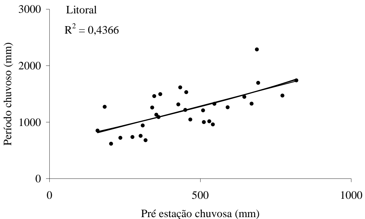
Figura 20. Relação linear entre as precipitações (mm) da pré-estação com a do período chuvoso para a microrregião do Litoral paraibano, no período de 1975 a 2005.
