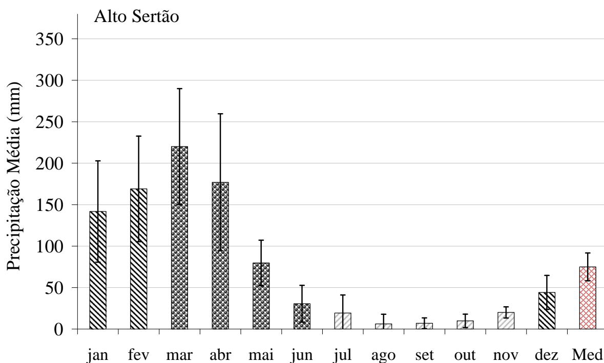
Figura 18. Precipitação média mensal (mm) para a microrregião do Alto Sertão do estado da Paraíba no período de 1975 a 2005, com destaque para pré-estação chuvosa (dez-fev) e estação chuvosa (mar-jun).
