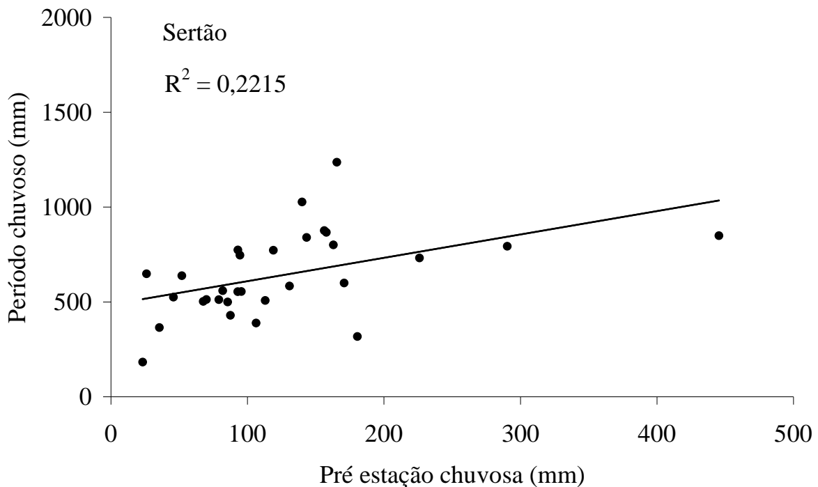
Figura 24. Relação linear entre as precipitações (mm) da pré-estação com a do período chuvoso para a microrregião do Sertão paraibano, no período de 1975 a 2005.
