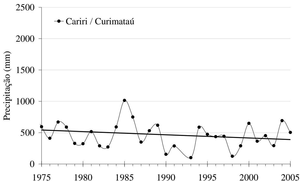
Figura 15. Variabilidade anual da precipitação (mm) para a microrregião do Cariri/Curimataú do estado da Paraíba, e a linha tendência, no período de 1975 a 2005.
