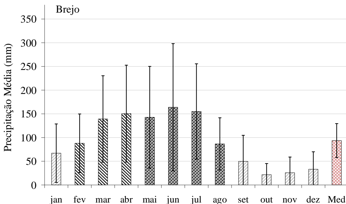
Figura 10. Precipitação média mensal (mm) para a microrregião do Brejo do estado da Paraíba no período de 1975 a 2005, com destaque para pré-estação chuvosa (fev-abr) e estação chuvosa (mai-ago).
