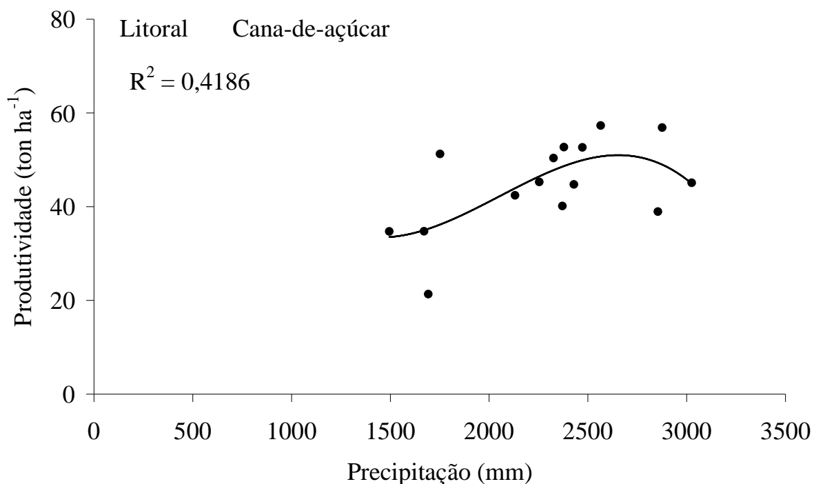
Figura 30. Correlação polinomial da precipitação pluvial (mm) durante o ciclo da cana-de-açúcar com a produtividade (ton.ha-1) da microrregião do Litoral da Paraíba, no período de 1990 a 2005
