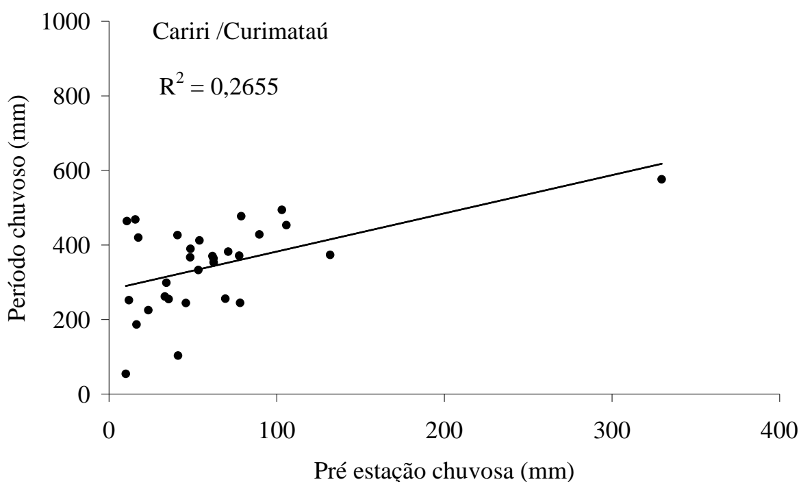
Figura 23. Relação linear entre as precipitações (mm) da pré-estação com a do período chuvoso para a microrregião do Cariri/Curimataú paraibano, no período de 1975 a 2005.
