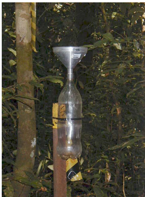
Figura 10. Pluviômetro utilizado para quantificar a precipitação interna
