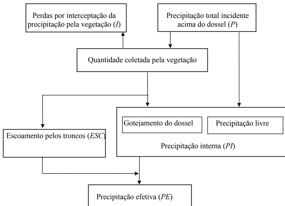
Figura 13. Fluxograma conceitual do processo de interceptação da precipitação pela vegetação e a precipitação que efetivamente chega ao solo. Adaptado de Valente et al. (1997)
