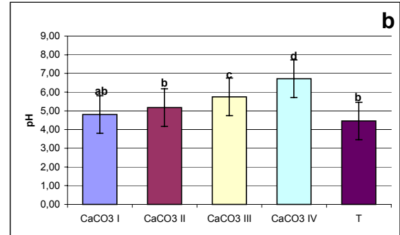
FIGURA 4 - TESTE DE TUKEY 5% PARA AS MÉDIAS DE pH DO SOLO DE CONTENDA. SENDO (a) pH EM H 2 O, (b) pH CaCl 2 e (c) pH SMP
