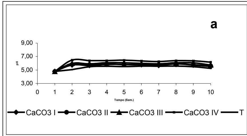
FIGURA 3 - CURVAS DE NEUTRALIZAÇÃO DO SOLO DE PALMEIRA EM FUNÇÃO DAS DOSES DE CARBONATO DE CÁLCIO APLICADAS. SENDO (a) pH EM ÁGUA, (b) pH CaCl 2 e (c) pH SMP
