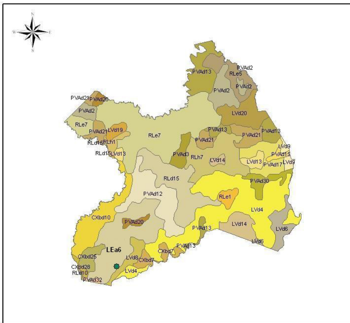
FIGURA 1 - MAPA DE SOLO DE ARAPOTI COM DESTAQUE DO PONTO DE AMOSTRAGEM
