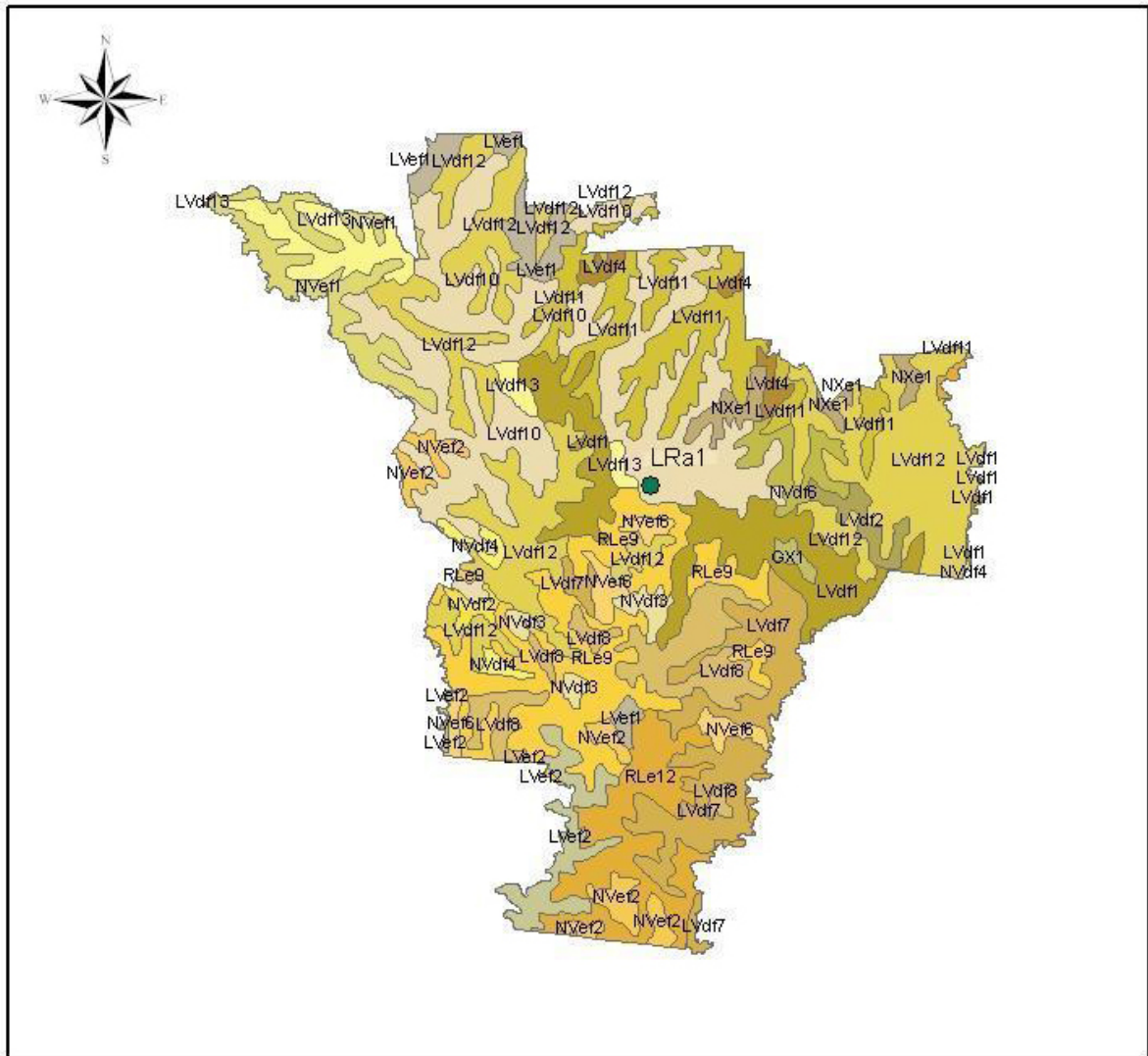
FIGURA 5 - MAPA DE SOLO DE CASCAVEL COM DESTAQUE DO PONTO DE AMOSTRAGEM
