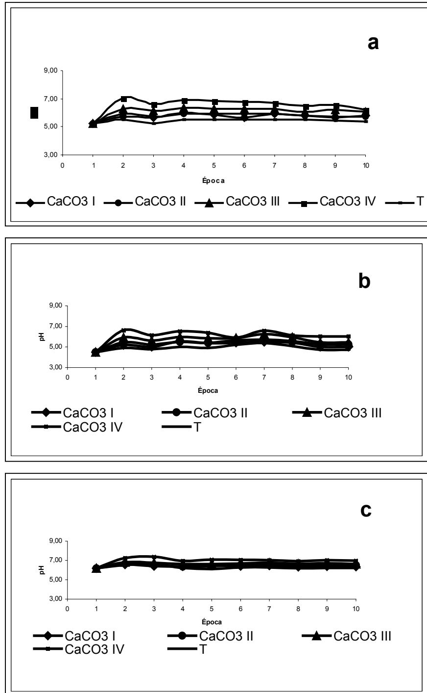
FIGURA 2 - CURVAS DE NEUTRALIZAÇÃO DO SOLO DE PONTA GROSSA EM FUNÇÃO DAS DOSES DE CARBONATO DE CÁLCIO APLICADAS. SENDO (a) pH EM ÁGUA, (b) pH CaCl 2 e (c) pH SMP
