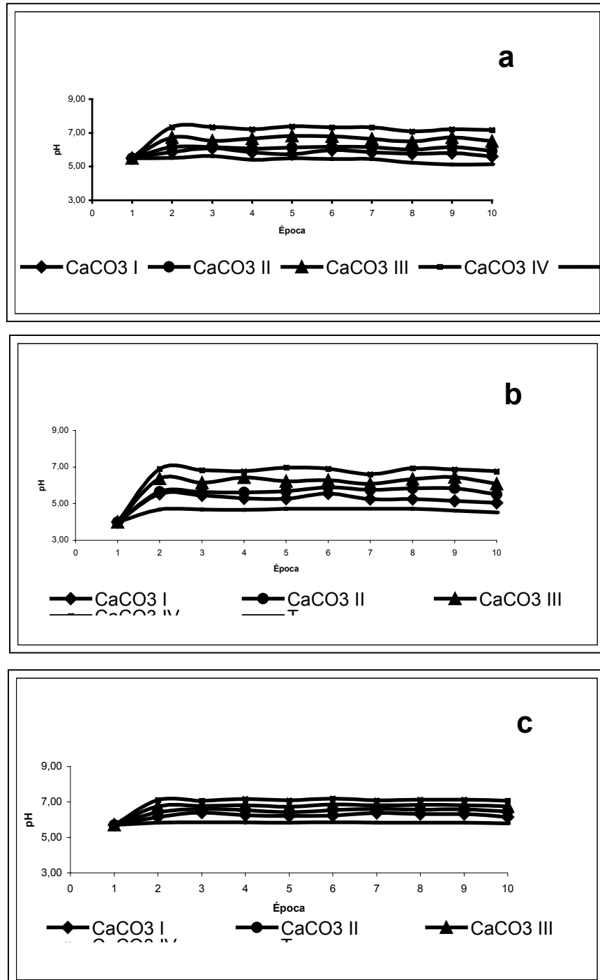
FIGURA 1 - CURVAS DE NEUTRALIZAÇÃO DO SOLO DE ARAPOTI EM FUNÇÃO DAS DOSES DE CARBONATO DE CÁLCIO APLICADAS. SENDO (a) pH EM ÁGUA, (b) pH CaCl 2 e (c) pH SMP
