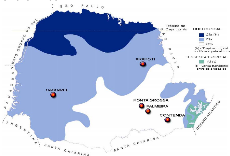
FIGURA 03 – MAPA DOS CLIMAS DO PARANÁ E LOCALIZAÇÃO DOS MUNICÍPIOS ESTUDADOS
