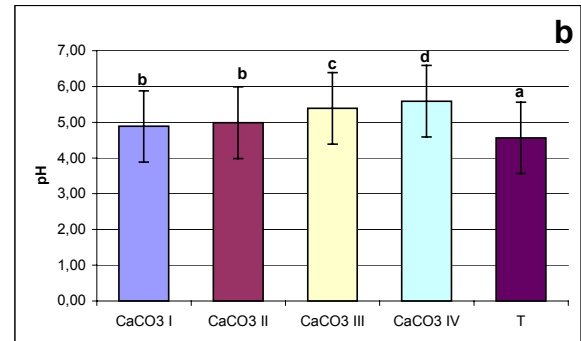
FIGURA 3 - TESTE DE TUKEY 5% PARA AS MÉDIAS DE pH DO SOLO DE PALMEIRA. SENDO (a) pH EM H 2 O, (b) pH CaCl 2 e (c) pH SMP
