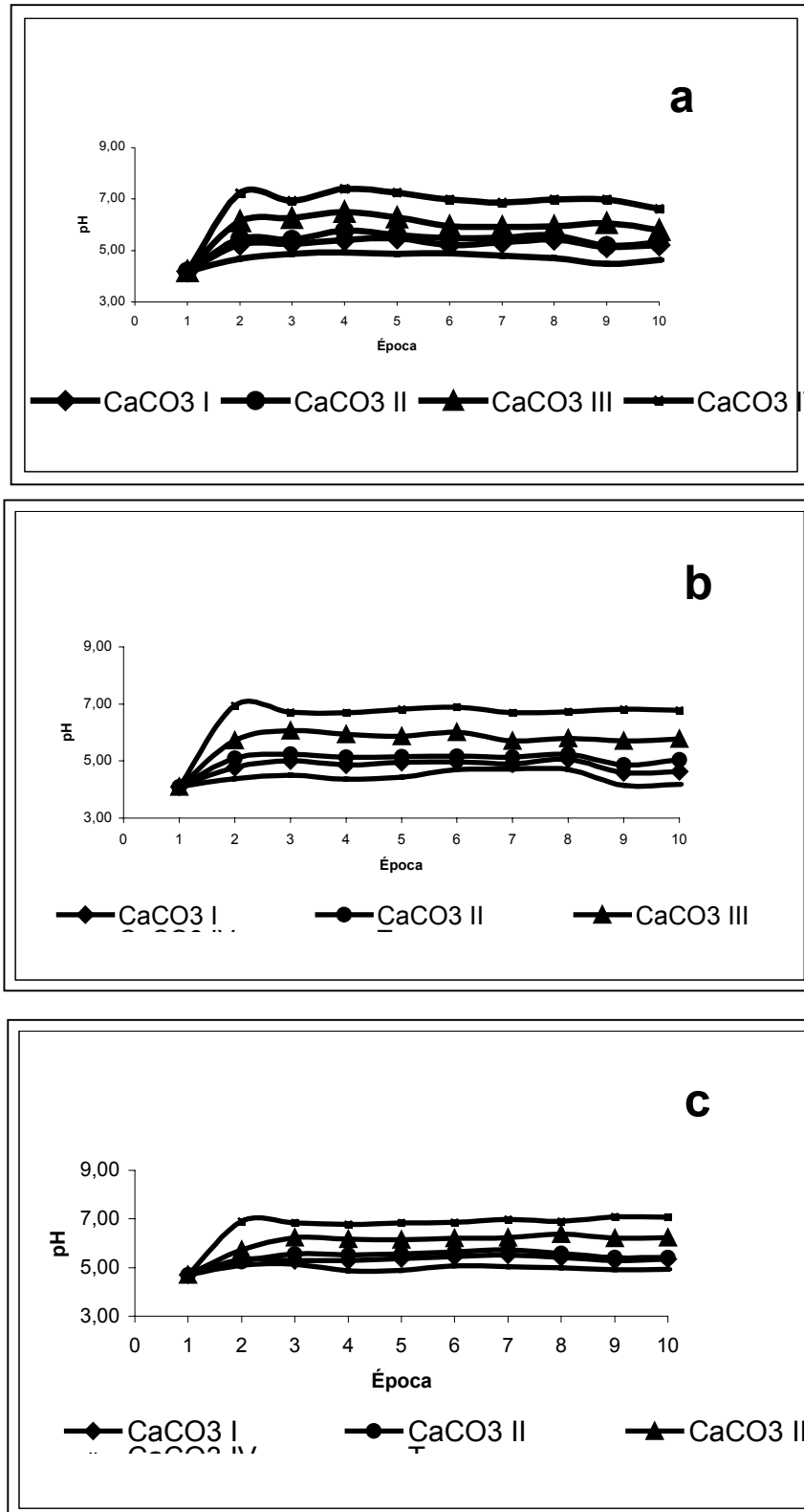
FIGURA 5 - CURVAS DE NEUTRALIZAÇÃO DO SOLO DE CASCAVEL EM FUNÇÃO DAS DOSES DE CARBONATO DE CÁLCIO APLICADAS. SENDO (a) pH EM ÁGUA, (b) pH CaCl 2 e (c) pH SMP
