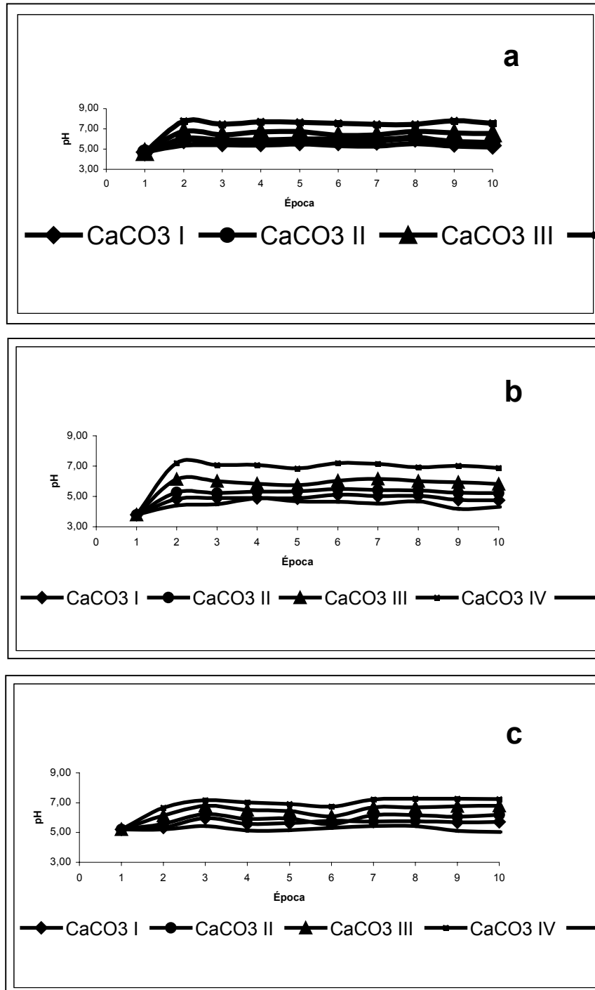
FIGURA 4 - CURVAS DE NEUTRALIZAÇÃO DO SOLO DE CONTENDA EM FUNÇÃO DAS DOSES DE CARBONATO DE CÁLCIO APLICADAS. SENDO (a) pH EM ÁGUA, (b) pH CaCl 2 e (c) pH SMP
