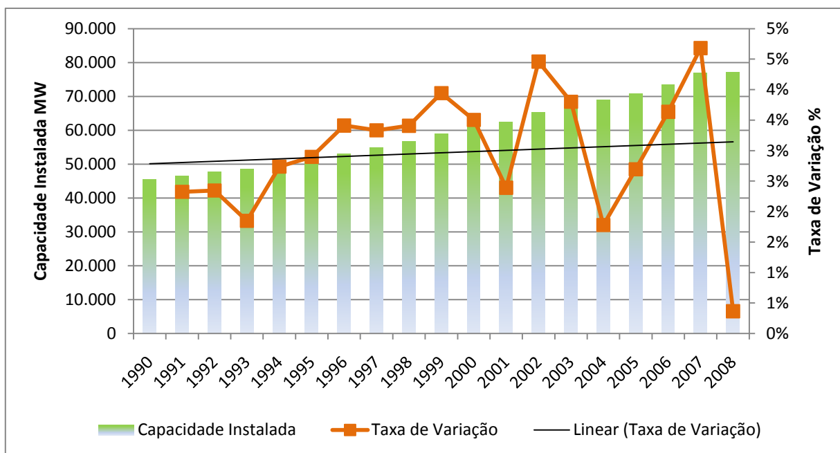
Gráfico 36 - Evolução da Potência Instalada de Fontes Hidrelétricas
