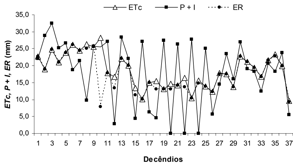
Figura 5.18 – Exemplo de balanço hídrico climatológico decendial ao longo de um ano, realizado para as localidades de (a) Colombo e (b) Campo Largo, considerando o armazenamento de água no solo respectivo das duas localidades, K_c para grãos/algodão (0,9) e fração p igual a 0,6
