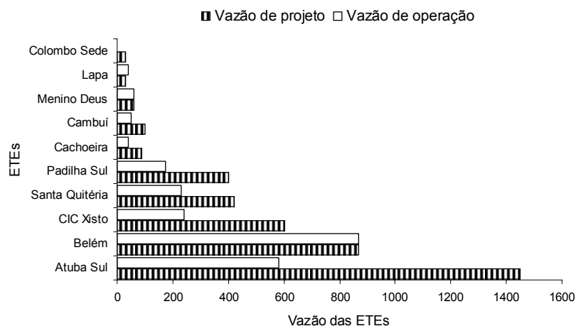
Figura 5.3 – Vazão de projeto e vazão média de efluentes tratados das principais Estações de Tratamento de Esgoto (ETEs) da Região Metropolitana de Curitiba
