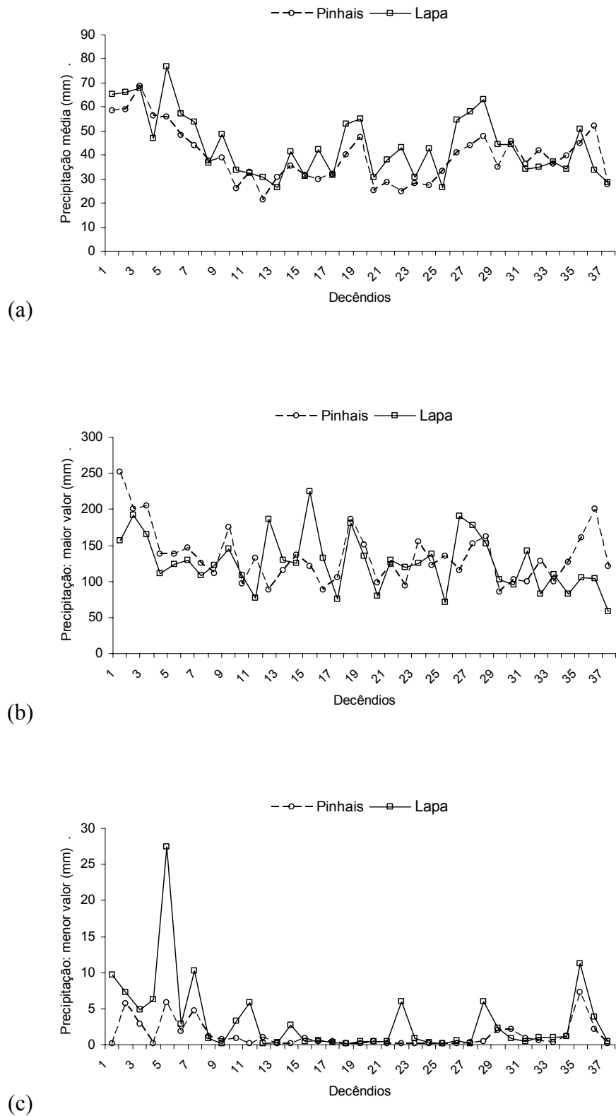
Figura 5.12 – Medidas dos valores de precipitação, agrupados em decênios, para a região de Pinhais e Lapa: (a) média; (b) maior valor e (c) menor valor
