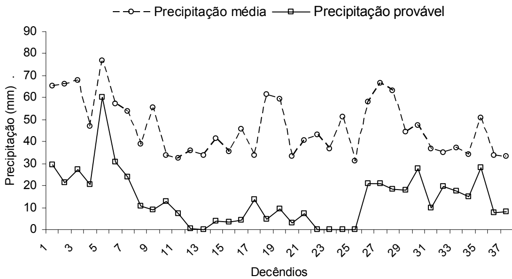
Figura 5.14 – Valores de precipitação, média e a 75% de probabilidade, calculados com a distribuição de melhor ajuste (Gama, Normal, Exponencial e Uniforme), para cidades de (a) Pinhais e (b) Lapa
