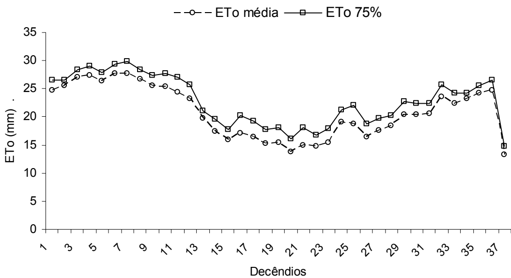
Figura 5.11 – Valores de evapotranspiração de referência ( ET_o ), média e a 75% de probabilidade, calculados com a distribuição de melhor ajuste (Gama, Normal, Exponencial e Uniforme), para cidades de (a) Pinhais e (b) Lapa
