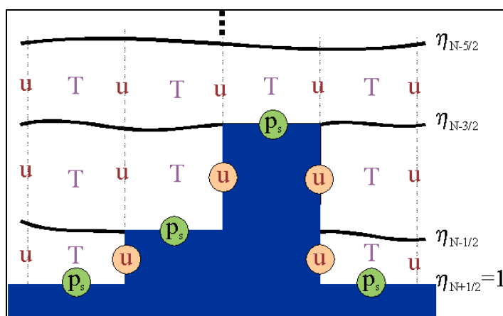
Figura 4.4 - Seção vertical idealizada da topografia do modelo Eta e distribuição das variáveis na vertical (u, T, Ps).
