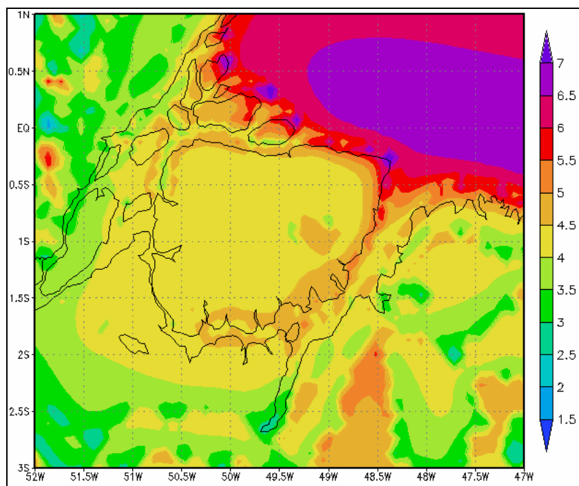
Figura 5.3 - Velocidade média sazonal do vento (m/s) a 50 m (JJA).
