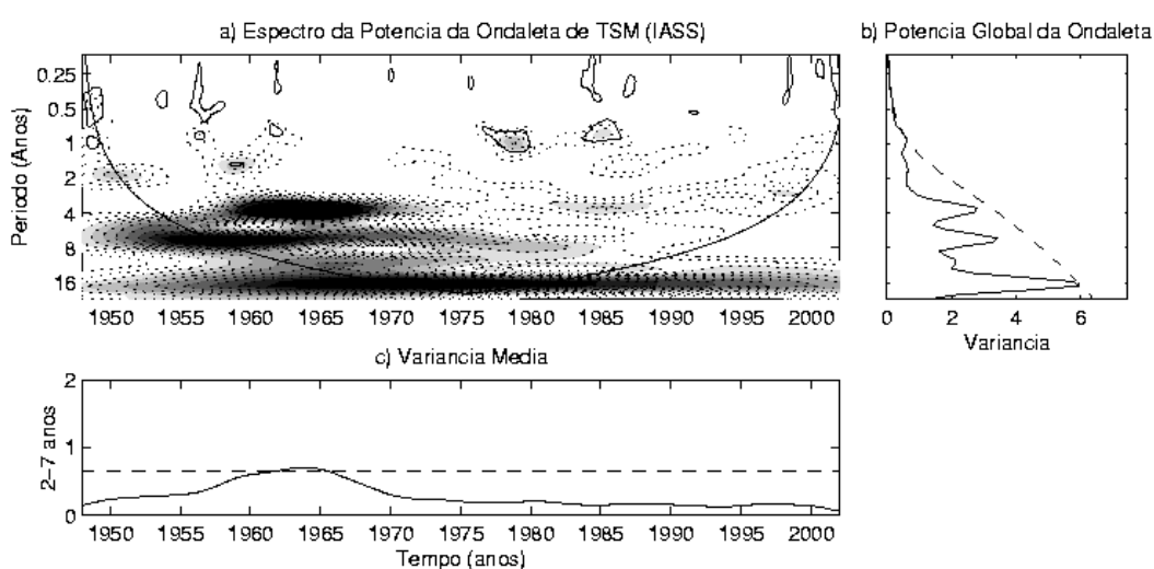
Figura 4.5 - Idem a Figura 4.1, exceto para o índice IASS e 1/\sigma^2 = 0,4385 .
