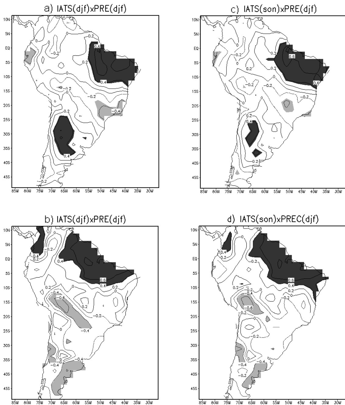
Figura 4.23 - Correlações totais simultâneas da precipitação com o IATS: a) para 1948-1976 e b) para 1977-2002. Correlações totais defasadas da precipitação em DJF com IATS em SON: c) para 1948-1976 e d) para 1977-2002, o intervalo das isolinhas é de 0,2.
