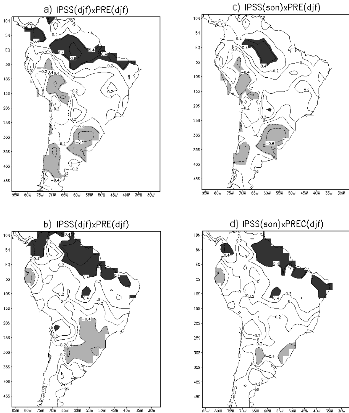
Figura 4.21 – Correlações totais simultâneas da precipitação com o IPSS: a) para 1948-1976 e b) para 1977-2002 e em c). Correlações totais defasadas da precipitação em DJF com IPSS em SON: c) para 1948-1976 e d) para 1977-2002, o intervalo das isolinhas é de 0,2.
