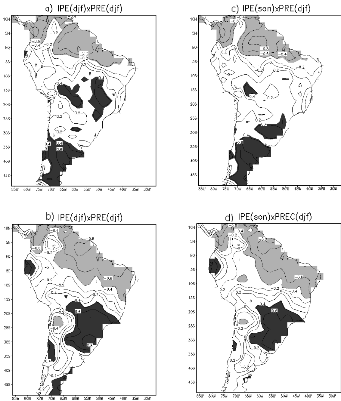
Figura 4.20 - Correlações totais simultâneas da precipitação com o IPE: a) para 1948-1976 e b) para 1977-2002. Correlações totais defasadas da precipitação em DJF com IPE em SON: c) para 1948-1976 e d) para 1977-2002, o intervalo das isolinhas é de 0,2.
