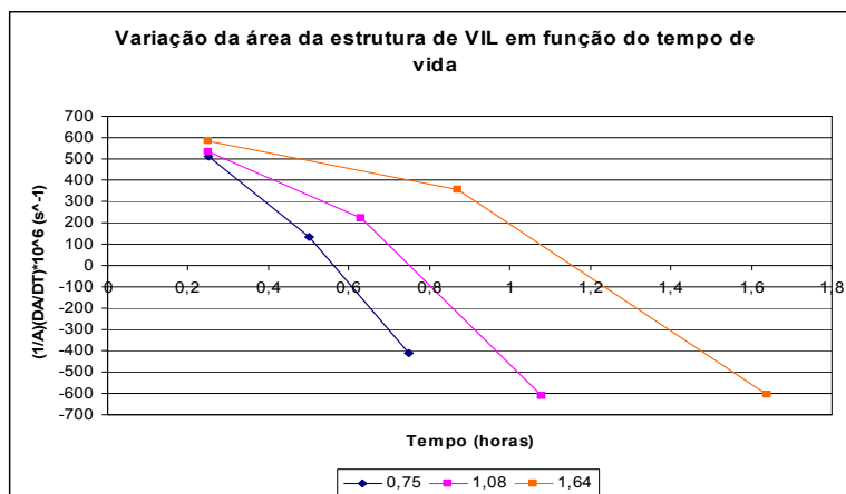
Figura 3.10 – Variação relativa da área com o tempo de acordo com o tempo de vida das estruturas de VIL . Valores positivos indicam crescimento, valores negativos significam decréscimo das estruturas de VIL .
