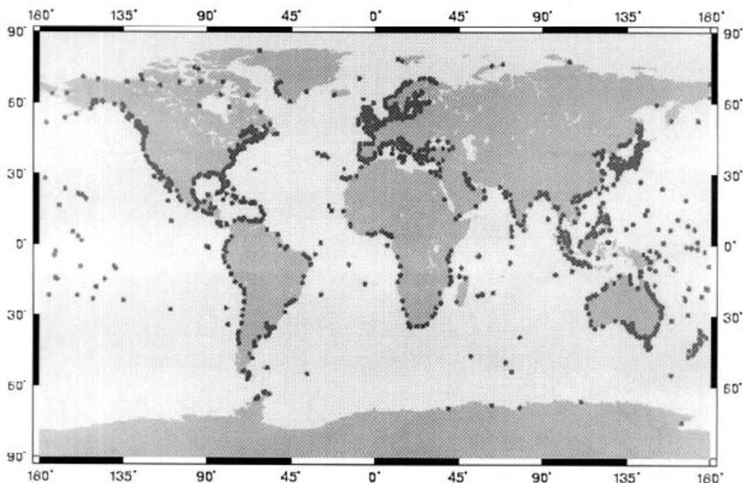
Figura 4 – Distribuição das estações (pontos) permanentes localizadas em todos os continentes e ilhas do planeta, colecionadas pelo Serviço Permanente para o Nível do Mar (PSMSL) 7
