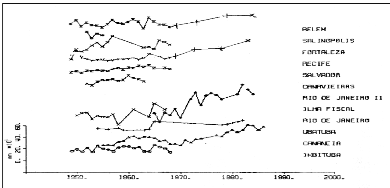
Figura 2 – Níveis de NMM em portos da costa Brasileira que mostra, na atualidade, uma tendência ao aumento do NMM da ordem de 40 cm/século 4
