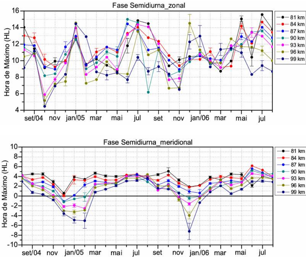
Figura 4.10 – Fases (hora de máximo) da maré semidiurna para a componente zonal (acima) e meridional (abaixo) variando ao longo do ano (meses) e em altitude (km), observadas em São João do Cariri entre o período que compreende agosto de 2004 a agosto de 2006.
