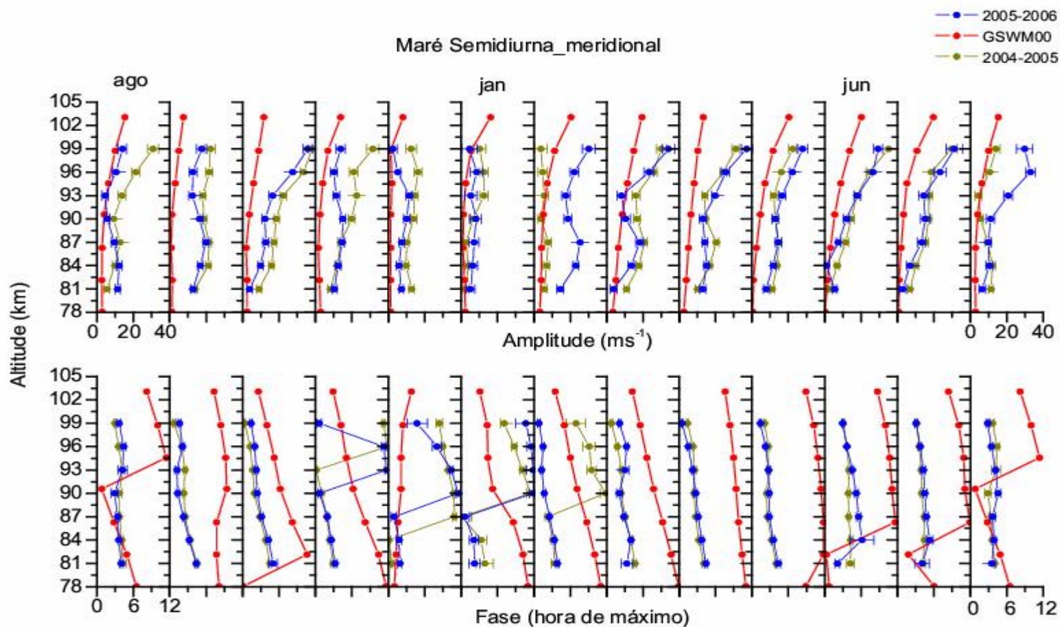
Figura 4.15 – Amplitudes (superior) e Fases (inferior) da maré semidiurna em função do tempo e da altitude observada em São João do Cariri entre o período que compreende de agosto de 2004 a agosto de 2006 para a componente meridional.
