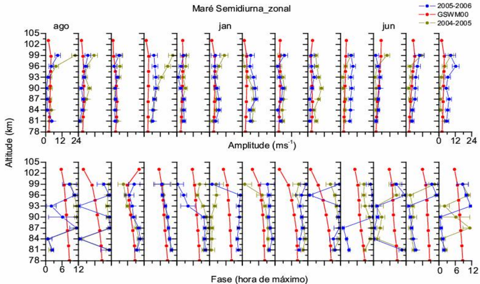
Figura 4.14 – Amplitudes (superior) e Fases (inferior) da maré semidiurna em função do tempo e da altitude observada em São João do Cariri entre o período que compreende de agosto de 2004 a agosto de 2006 para a componente zonal.
