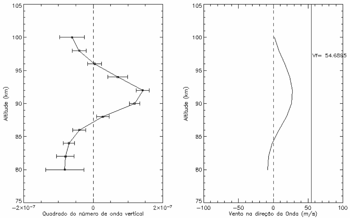
Figura 4.1 - Perfil de k_z^2 para o evento de onda canalizada (esquerda) e perfil do vento médio ao longo da direção da propagação da onda (direita) no dia 31/08/2005.
