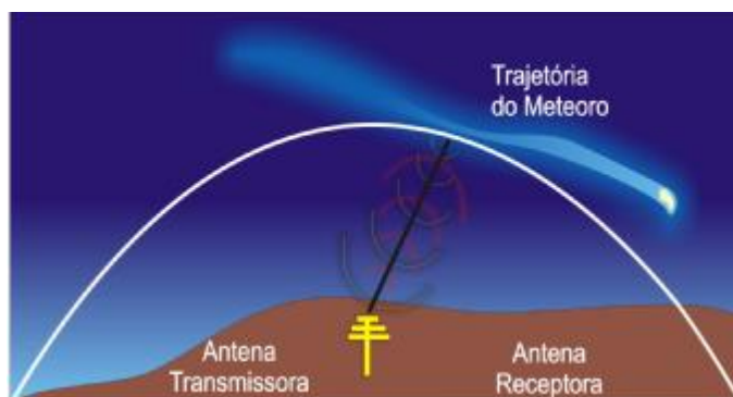
Figura 3.4 – Configuração para o radar mono-estático ( backscatter )
