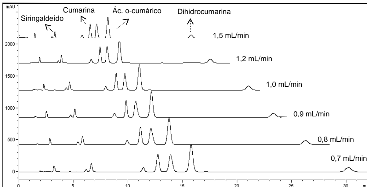
FIGURA 11 – CROMATOGRAMAS OBTIDOS ATRAVÉS DE CLAE-DAD UTILIZANDO DIFERENTES VAZÕES DE FLUXO.
