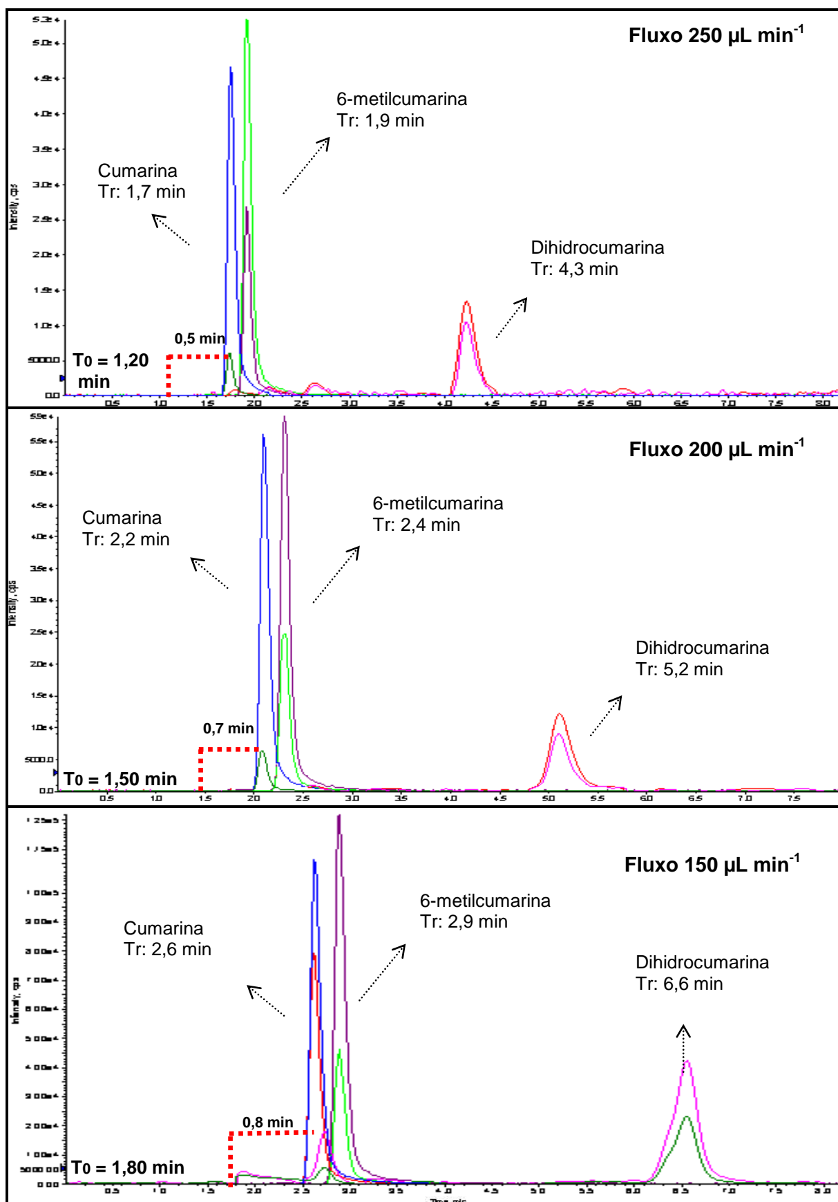
FIGURA 35: CROMATOGRAMAS DOS PADRÕES DE CUMARINA, 6-METILCUMARINA E DIHIDROACUMARINA OBTIDOS ATRAVÉS DE CLAE-EM/EM (ESI+) UTILIZANDO DIFERENTES VAZÕES DE FLUXO.
