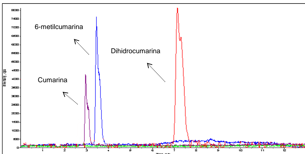
FIGURA 32 – CROMATOGRAMA DOS PADRÕES DE CUMARINA, 6-METILCUMARINA E DIHIDROACUMARINA OBTIDO ATRAVÉS DE CLAE-EM/EM (ESI+) UTILIZANDO COLUNA ZORBAX ® EM UMA VAZÃO DE FLUXO DE 800 \mu\text{L min}^{-1} .
