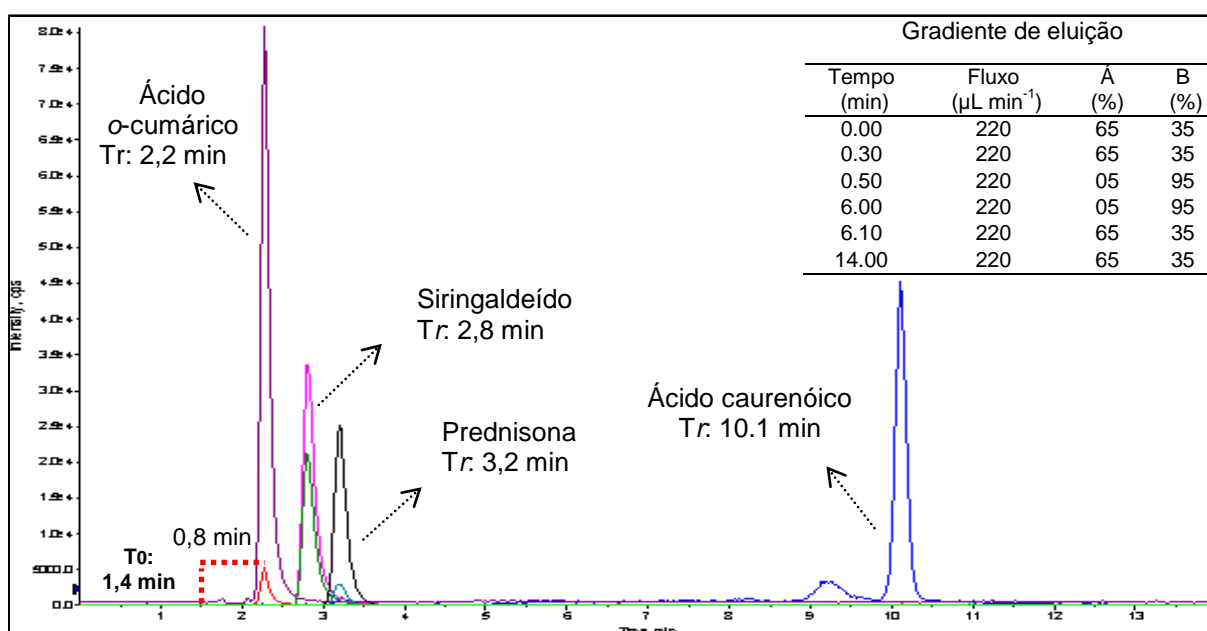
FIGURA 40 – CROMATOGRAMA DA PREDNISONA, ÁCIDO CAURENÓICO, ÁCIDO O-CUMÁRICO E SIRINGALDEÍDO OBTIDO APÓS AS OTIMIZAÇÕES DO MÉTODO (ESI-). NOTA: Condições de análise: Fase móvel: A%: Água (5mM formiato de amônio), B%: Solução acetonitrila/água 97:3 v/v (5 mM formiato de amônio); Temperatura de forno: 25 °C
