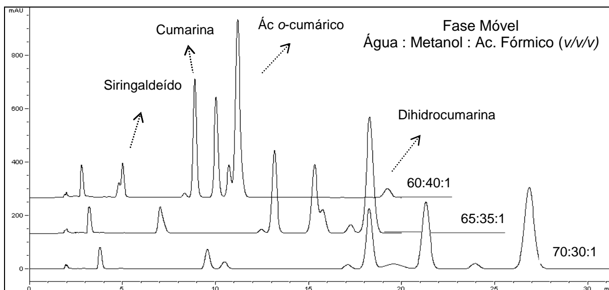
FIGURA 9 – PERFIL CROMATOGRÁFICO DA SOLUÇÃO ORAL DE GUACO (AMOSTRA 1) FORTIFICADA COM 25 \mu\text{g mL}^{-1} DE CUMARINA, ÁC. O-CUMÁRICO, DIHIDROCURARINA E SIRINGALDEÍDO UTILIZANDO DIFERENTES PROPORÇÕES DE ÁGUA E METANOL NA COMPOSIÇÃO DA FASE MÓVEL.
