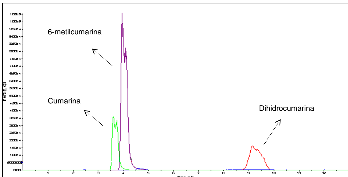
FIGURA 31 – CROMATOGRAMA DOS PADRÕES DE CUMARINA, 6-METILCUMARINA E DIHIDROACUMARINA OBTIDO ATRAVÉS DE CLAE-EM/EM (ESI+) UTILIZANDO COLUNA ZORBAX ® NO DESENVOLVIMENTO DO MÉTODO.
