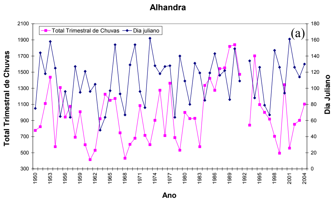
Figura 6 – Gráficos do total trimestral mais chuvoso e do início do período mais chuvoso do ano (91 dias consecutivos) em dia Juliano, (a) Alhandra; (b) Bananeiras; (c) Catolé do Rocha; (d) Ingá; (e) Monteiro; (f) Nova Olinda; (g) Pedra Lavrada; (h) Umbuzeiro.
