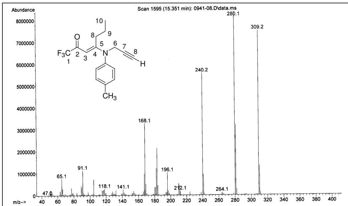
Figura 104. Espectro de massas da ( E )-1,1,1-Trifluor-4-[4-tolil-(2-propinil)amino]-3-hepten-2-ona 17c .
