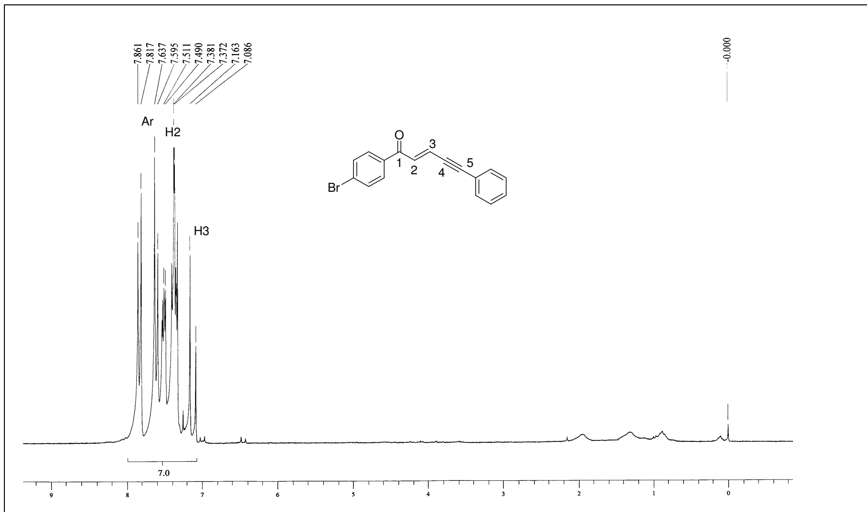
Figura 85. Espectro de RMN ^1\text{H} da (E)-1-(4-Bromofenil)-5-fenil-2-penten-4-in-1-ona 38 em \text{CDCl}_3 .
