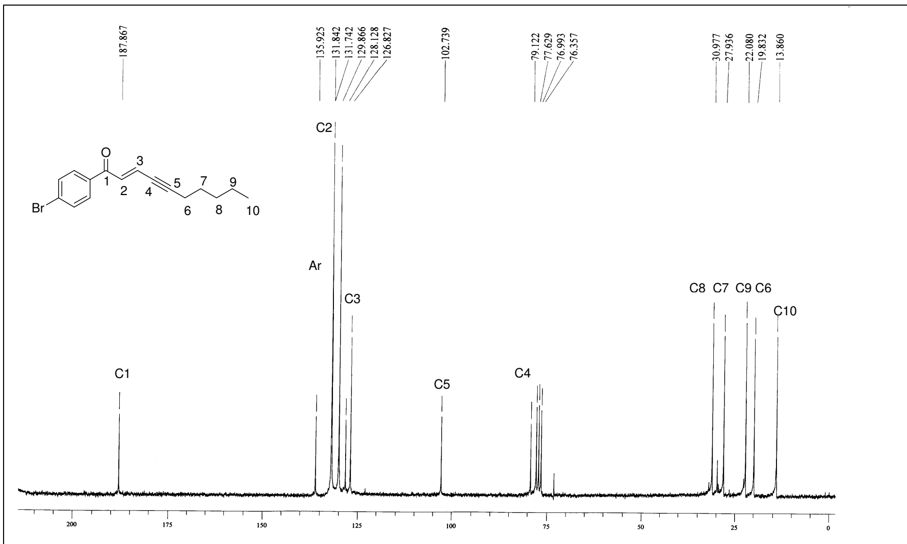
Figura 78. Espectro de RMN 13 C da (E)-1-(4-Bromofenil)-2-decen-4-in-1-ona 34 em CDCl 3 .
