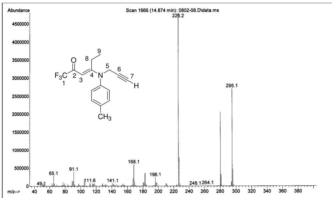
Figura 103. Espectro de massas da ( E )-1,1,1-Trifluor-4-[4-tolil-(2-propinil)amino]-3-hexen-2-ona 17b .
