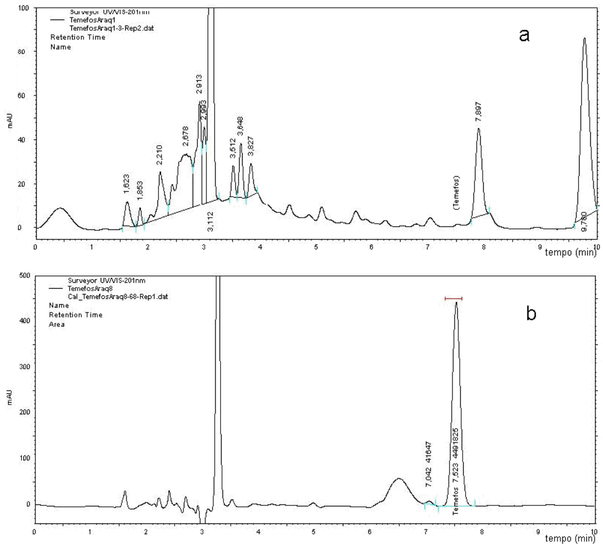
Figura 1. Cromatogramas: (a) amostra sem temefós, (b) amostra com 6,8 mg.L -1 de temefós.
